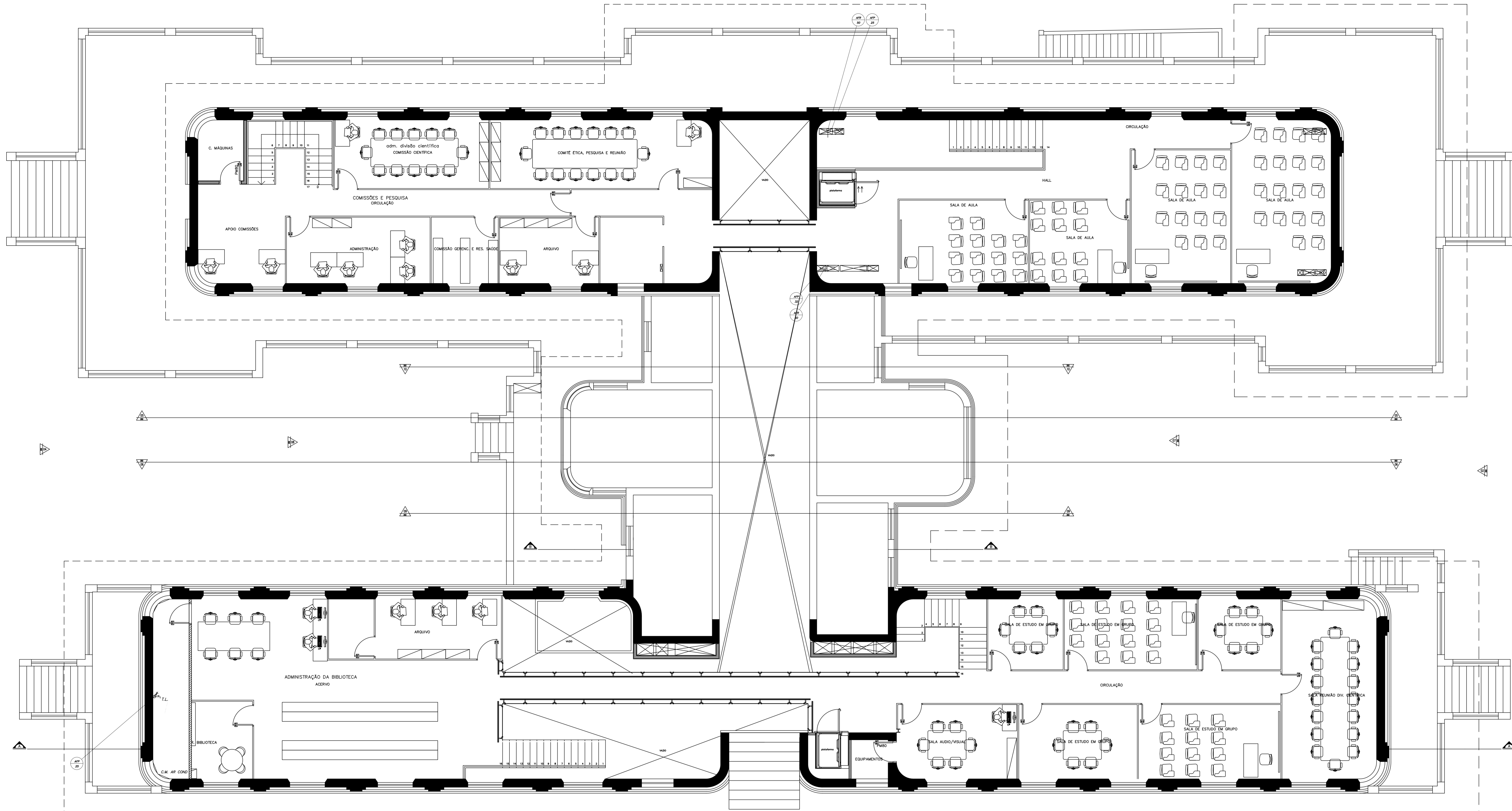
PLANTA SUPERIOR - LAYOUT
