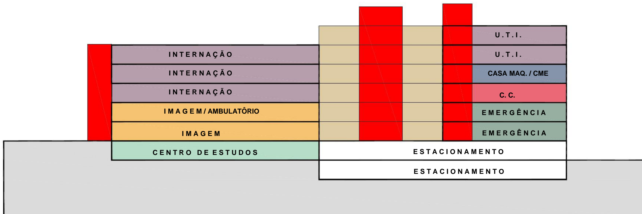
CORTE ESQUEMÁTICO HOSPITAL
