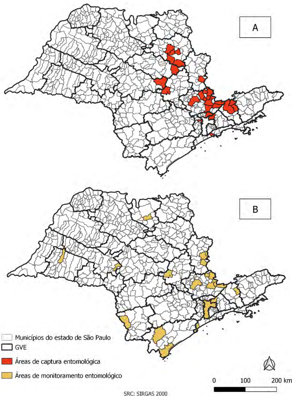
Figura 7. Capturas entomológicas realizadas decorrente da notificação de casos humanos autóctones e primatas não humanos confirmados para febre amarela (A) e monitoramento entomo-virológico (B). Estado de São Paulo, 2024-2025.
