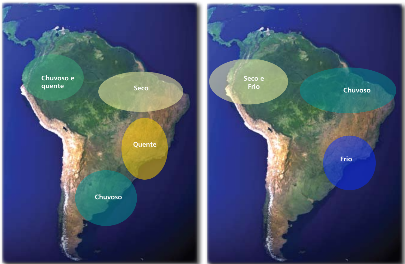
Figura 2: Impactos do El Niño (mapa da esquerda) e da La Niña (mapa da direita) sobre a América do Sul. Adaptada de INPE/CPTec (2006).
