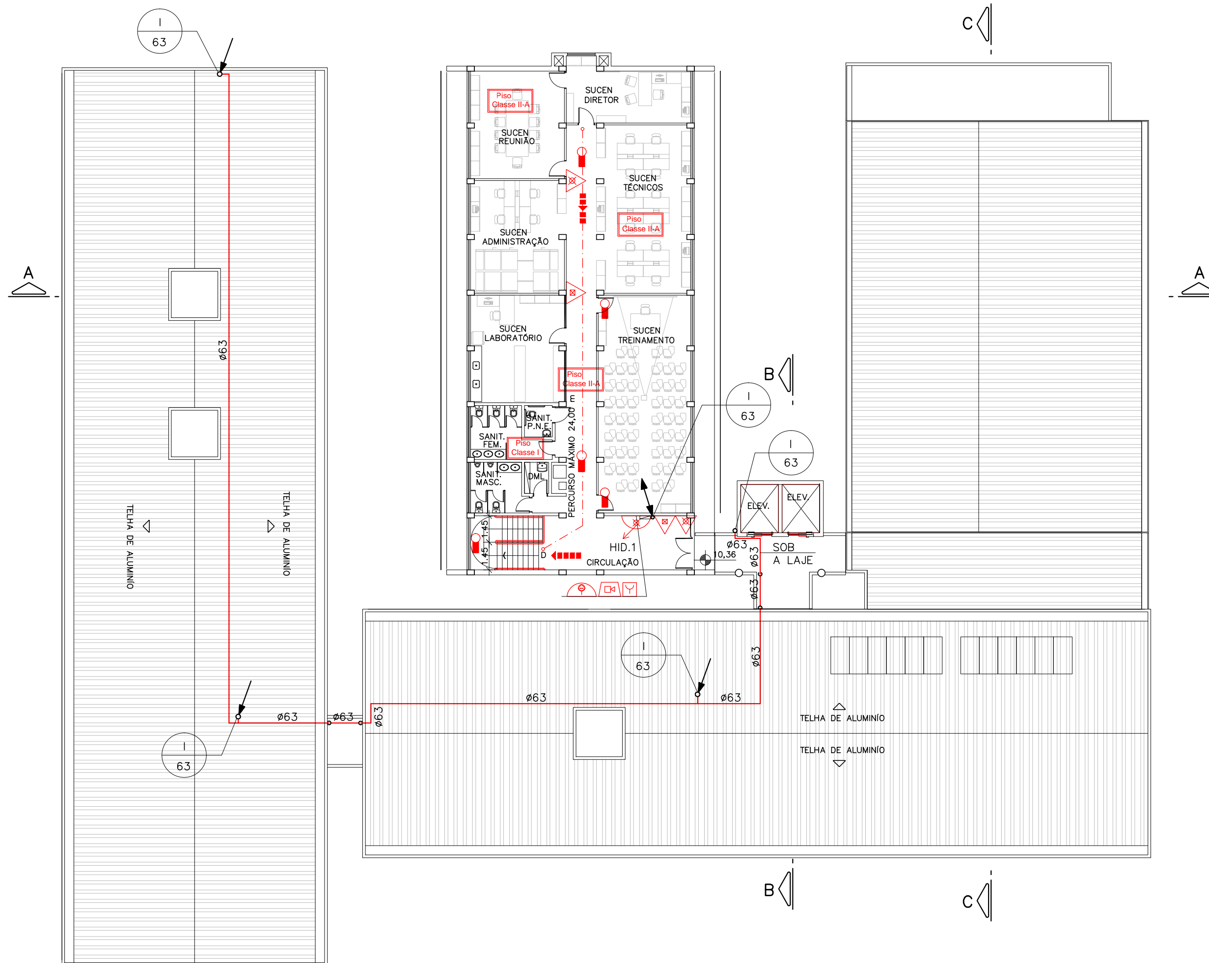
PLANTA 3º PAVIMENTO ESC. 1:200
