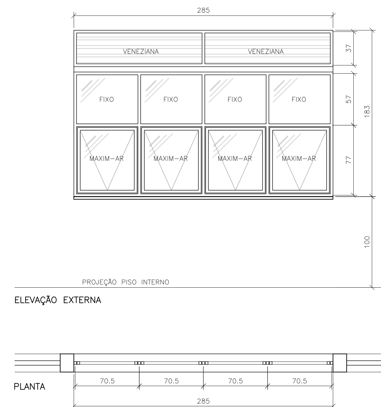
JA20 - 2,85 x 1,83m (30 unid.) ESCALA 1:25
