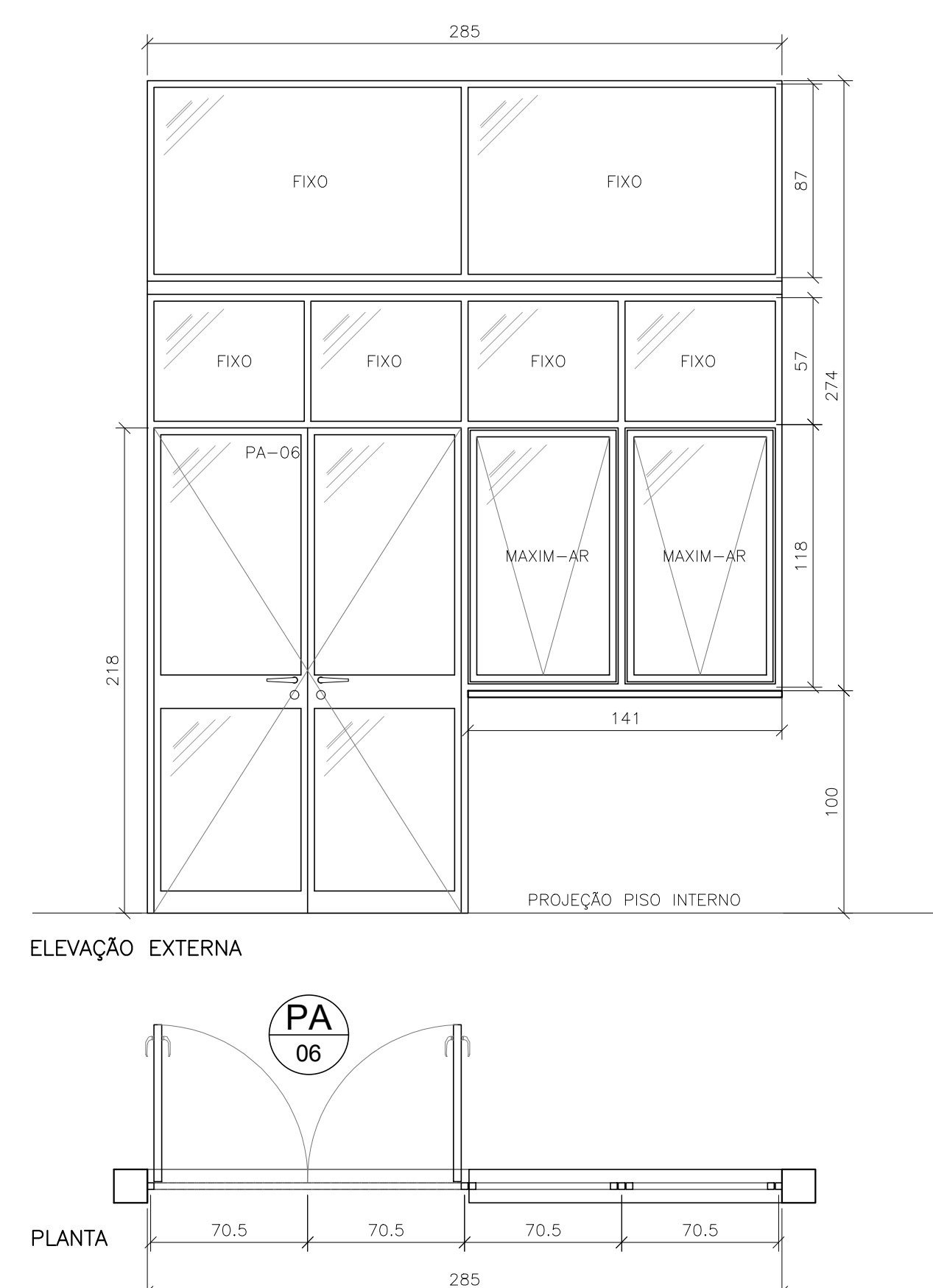
JA19 - 2,85 x 2,74m (01 unid.) ESCALA 1:25
