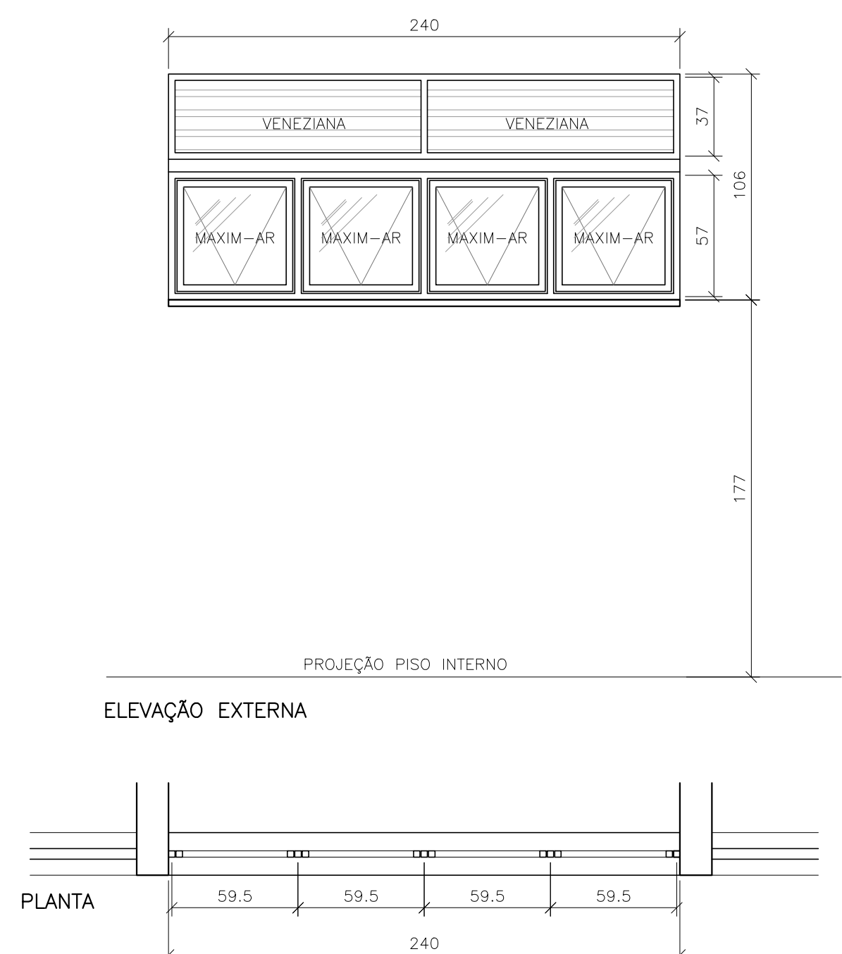
JA22 - 2,40 x 1,06m (10 unid.) ESCALA 1:25
