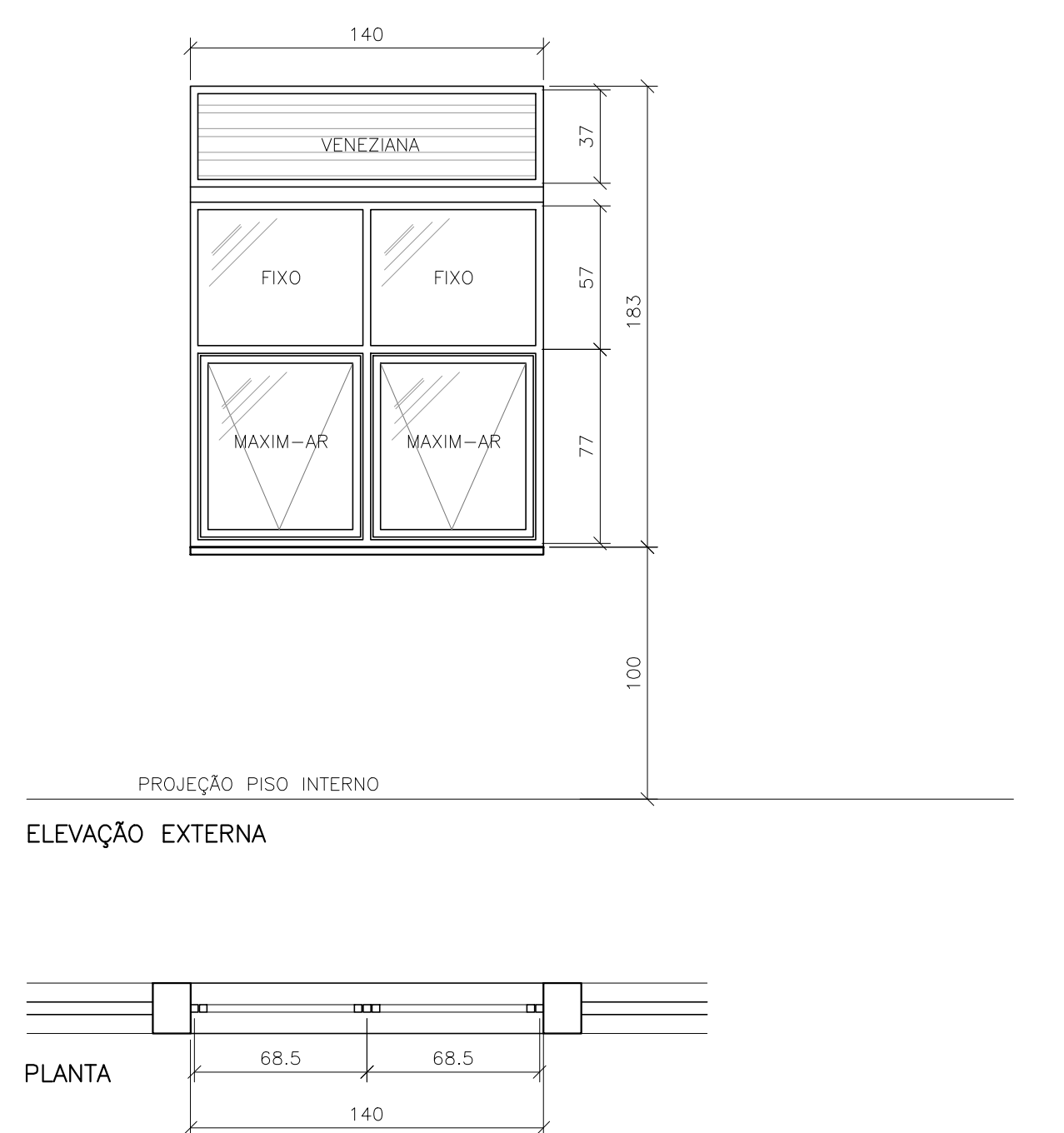
JA24 - 1,40 x 1,83m (02 unid.) ESCALA 1:25
