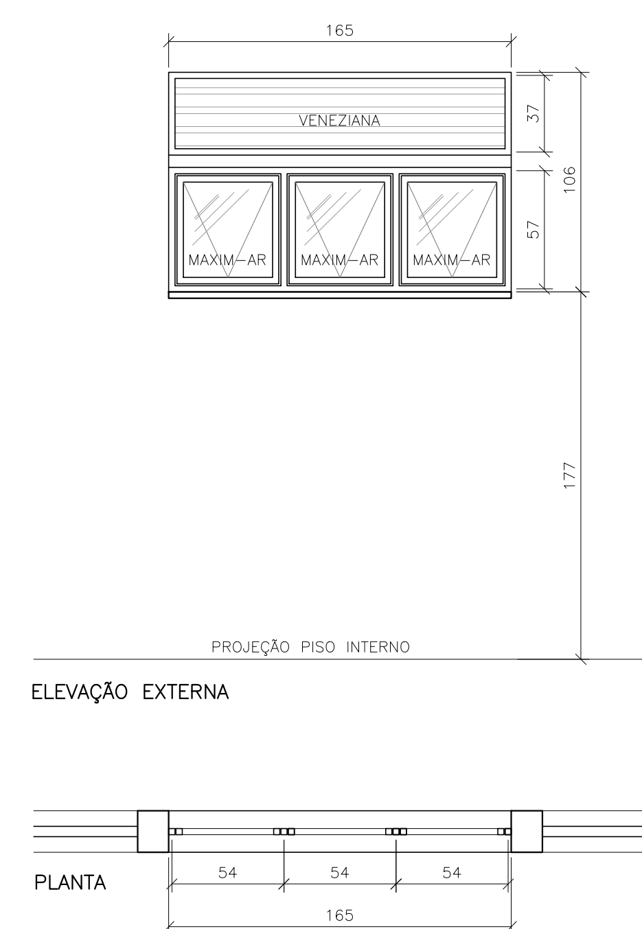
JA23 - 1,65 x 1,06m (04 unid.) ESCALA 1:25
