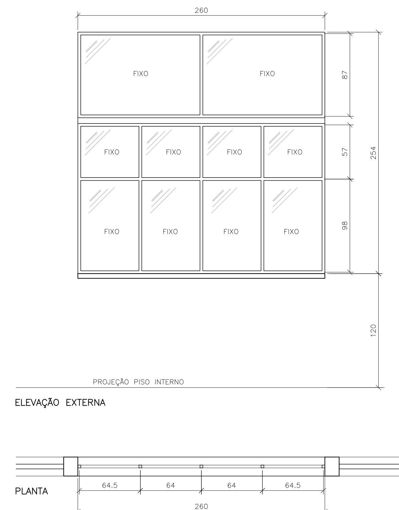
JA18 - 2,60 x 2,54 (01 unid.) ESCALA 1:25
