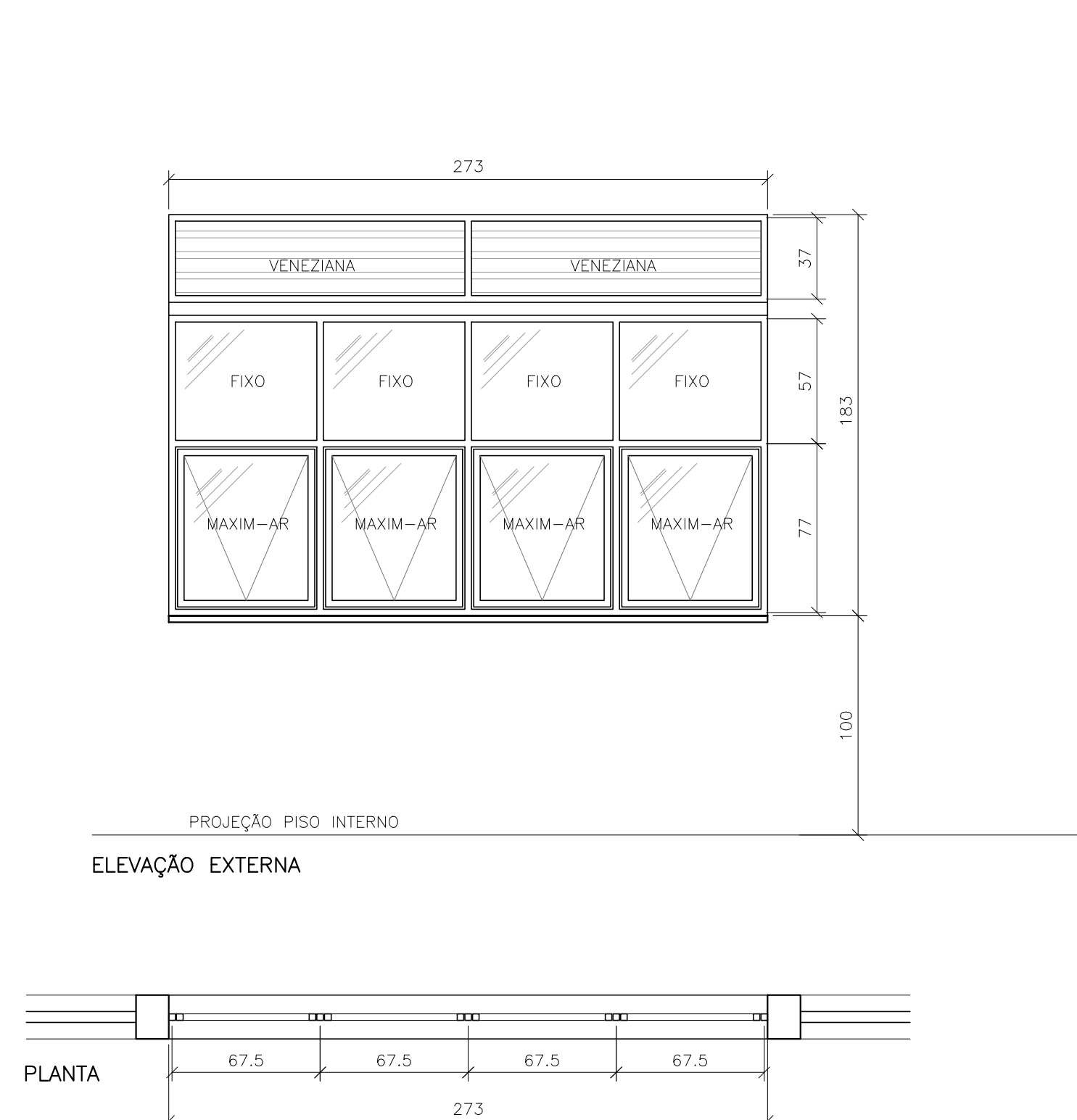
JA21 - 2,73 x 1,83m (12 unid.) ESCALA 1:25
