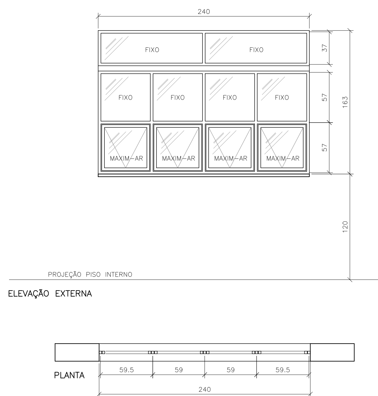
JA25 - 2,40 x 1,63m (04 unid.) ESCALA 1:25
