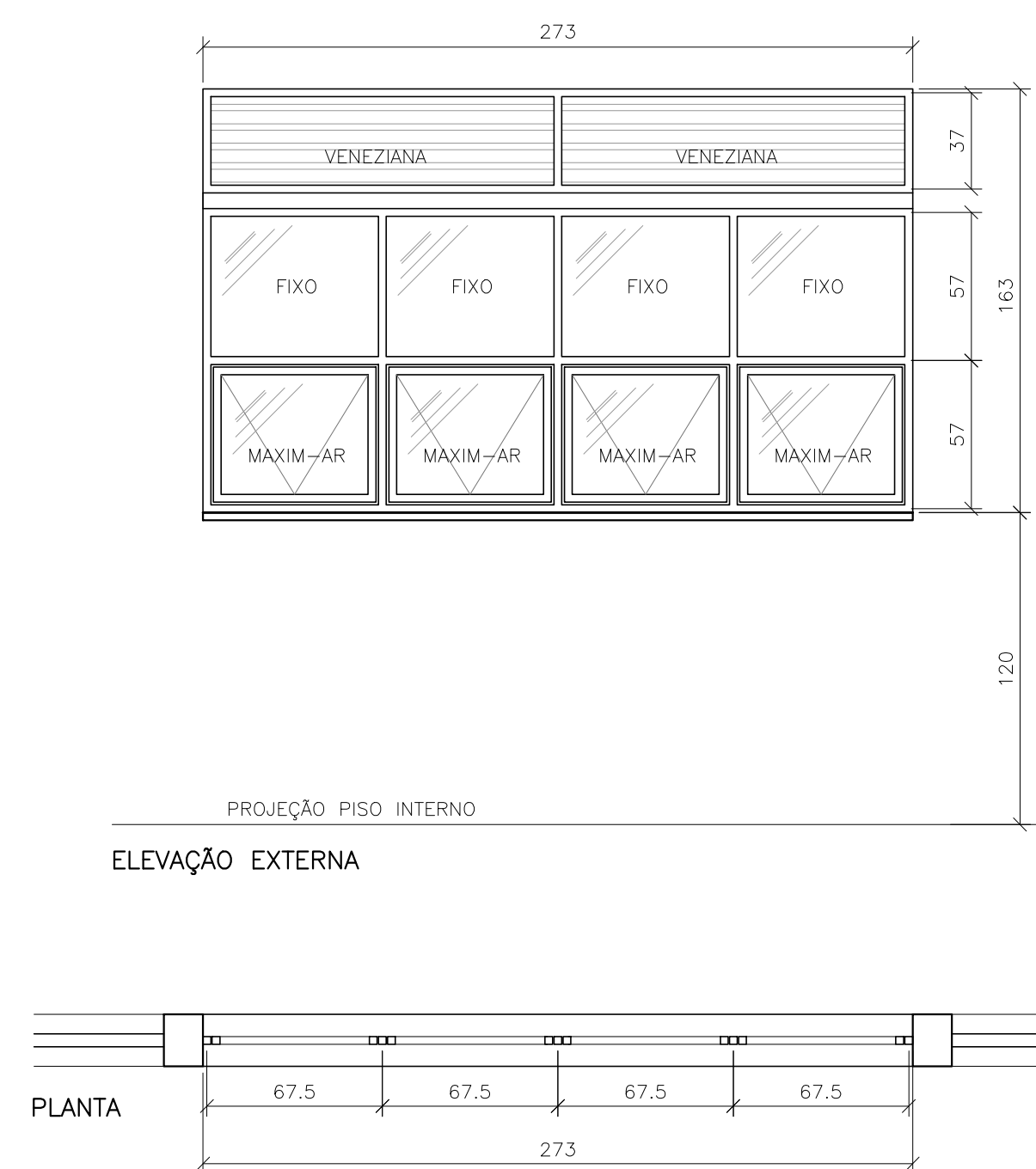
JA26 - 2,73 x 1,63m (06 unid.) ESCALA 1:25
