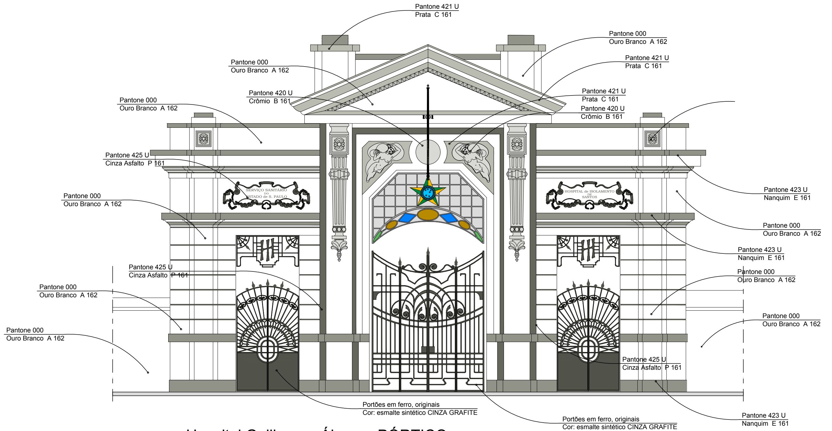
Hospital Guilherme Álvaro - PÓRTICO ELEVAÇÃO FRONTAL Estudo Cromático desenvolvido com base no Laudo Estratigráfico Escala 1:75
