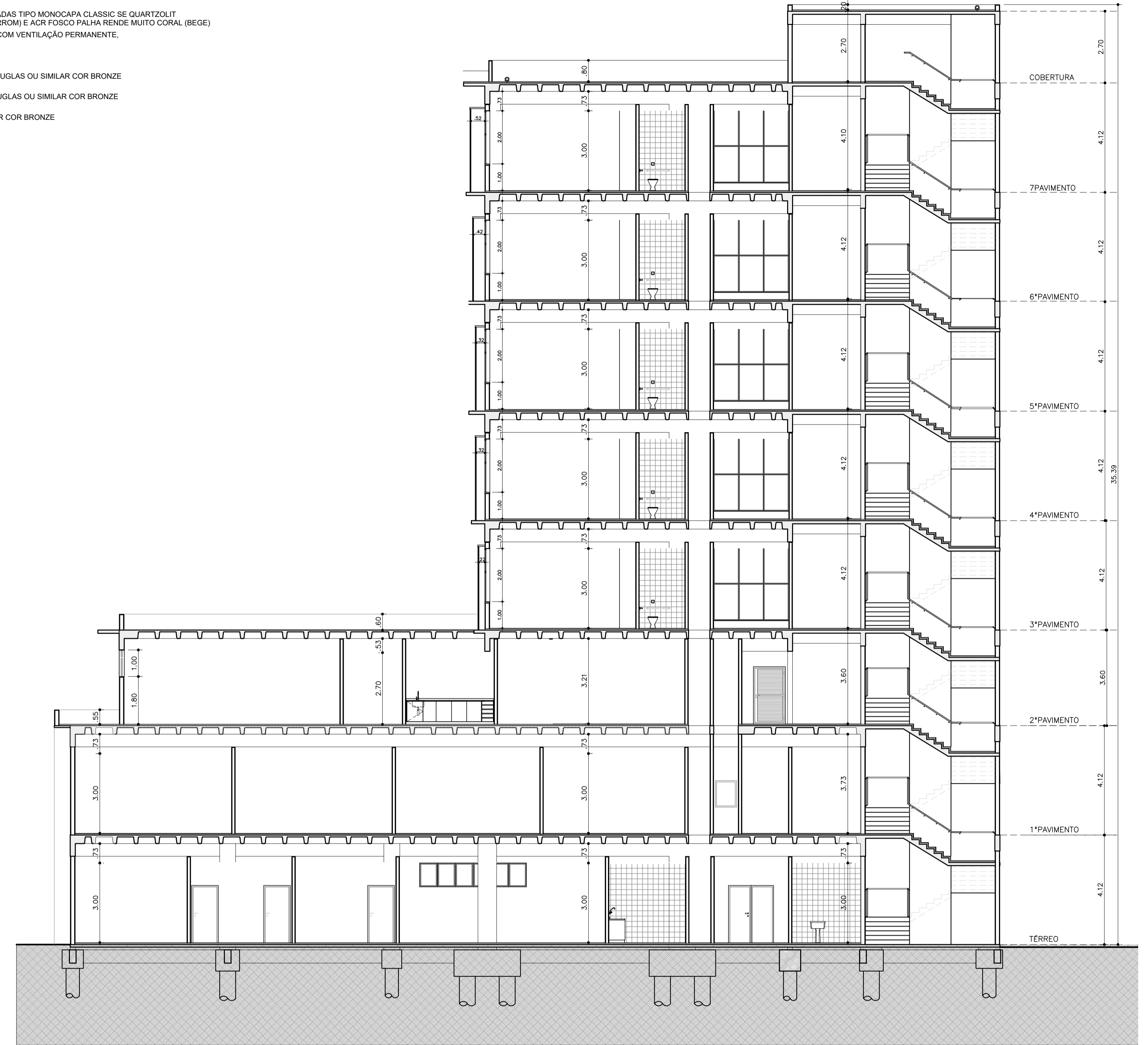
CORTE TRANSVERSAL
