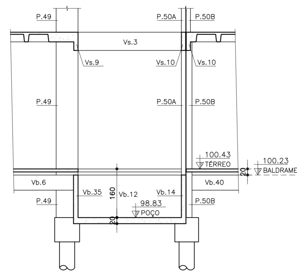
CORTE 1-1 ESCALA 1:75
