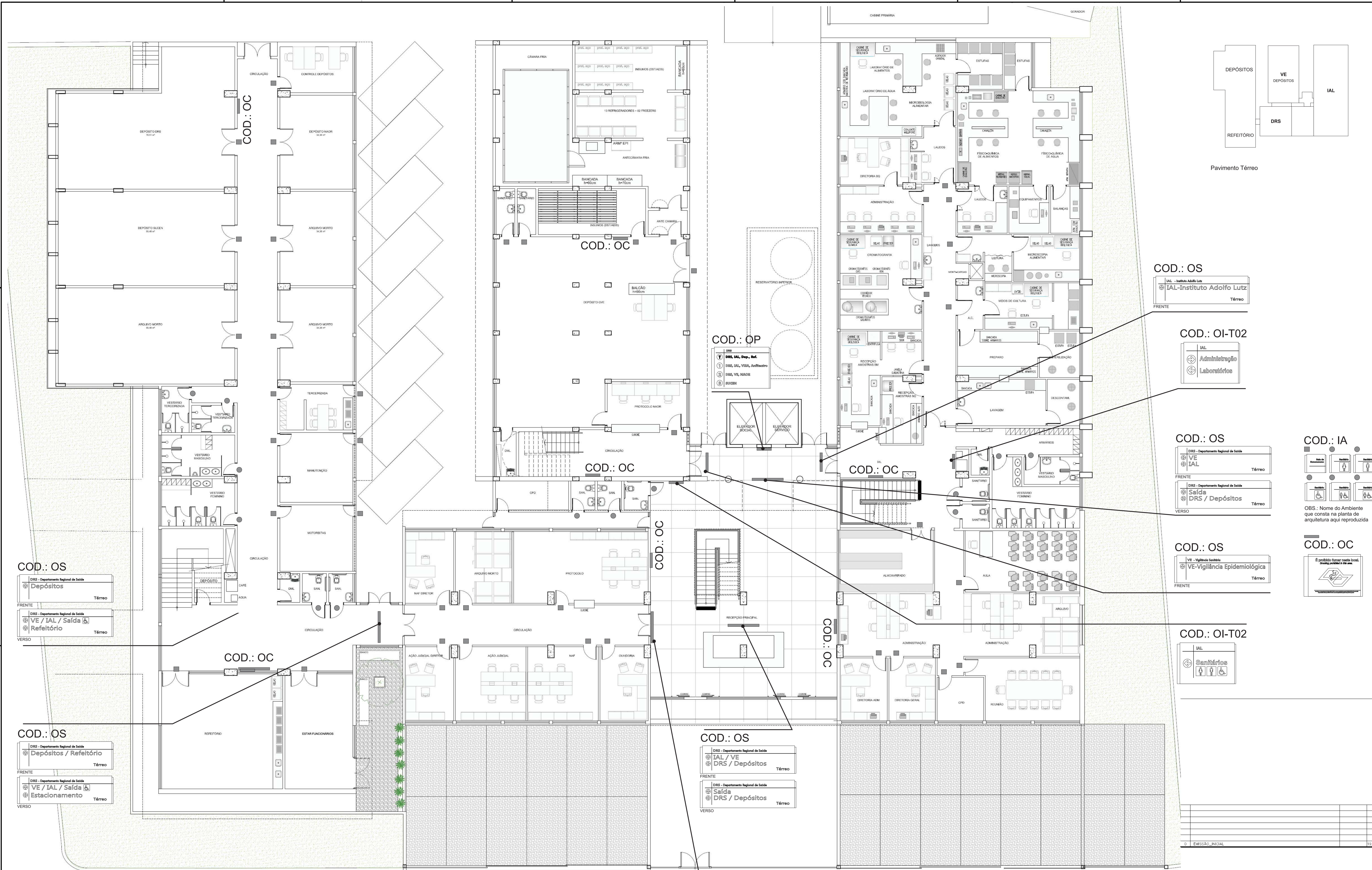
PLANTA - PAVIMENTO TÉRREO esc 1:75
