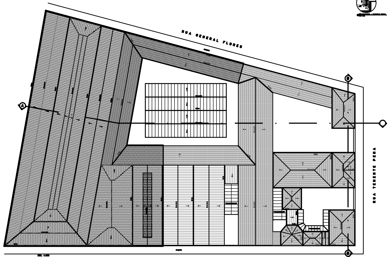
ESC. 1/200 RUA DOS ITALIANOS PLANTA DA COBERTURA - ÁREA A SER REFORMADA
