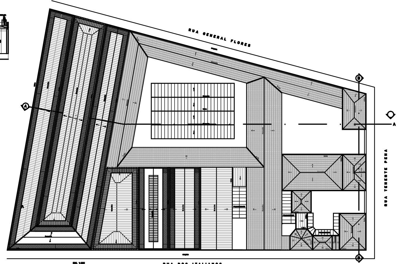
ESC. 1/200 RUA DOS ITALIANOS PLANTA DA COBERTURA - PLATAFORMAS
