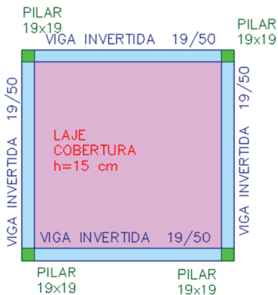
Figura 30 – PRÉDIO CCI - RESERVA DE INCÊNDIO E CASA DE BOMBAS - PLANTA ESTRUTURAL DA FUNDAÇÃO
