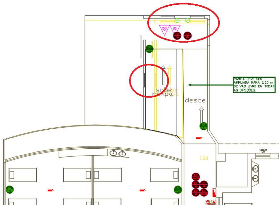
Figura 4 – PRÉDIO CCC - PAVIMENTO TÉRREO – Relocação de janelas
