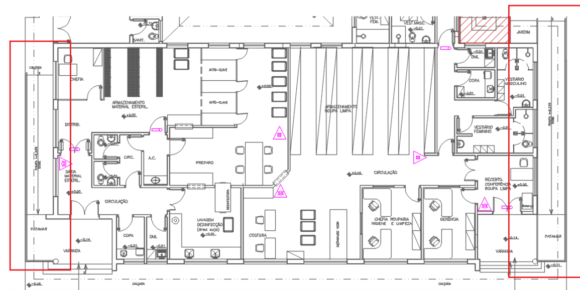
Figura 50 – PRÉDIO LAVANDERIA – RAMPAS 2 e 3 – RAMPAS EXISTENTES
