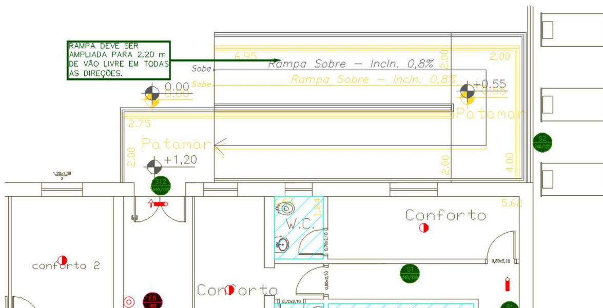
Figura 26 – PRÉDIO CCC – RAMPA 2 – SOBREPÓSICÃO RAMPA Á DEMOLIR (AMARELO) x NOVO LAYOUT DA RAMPA
