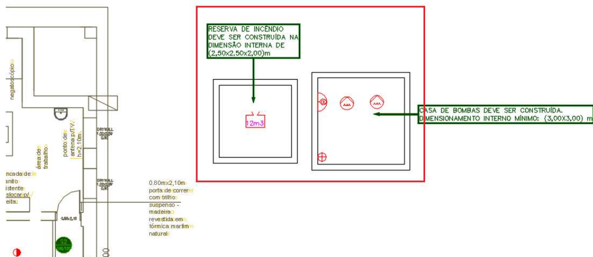
Figura 17 – PRÉDIO CCC – RESERVA DE INCÊNCIO E CASA DE BOMBAS - LAYOUT ARQUITETURA
