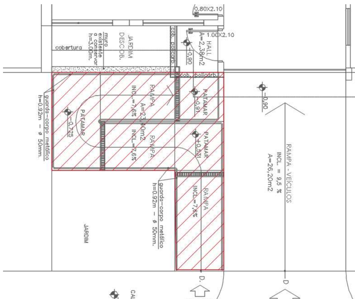
Figura 71 – PRÉDIO FROTA E PATRIMÔNIO – RAMPA – RAMPA EXISTENTE Á DEMOLIR
