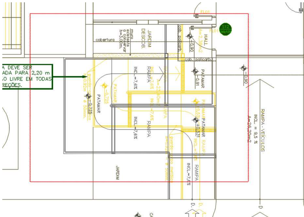
Figura 73 – PRÉDIO FROTA E PATRIMÔNIO – RAMPA – SOBREPOSIÇÃO RAMPA EXISTENTE (amarelo) x NOVO LAYOUT DA RAMPA
