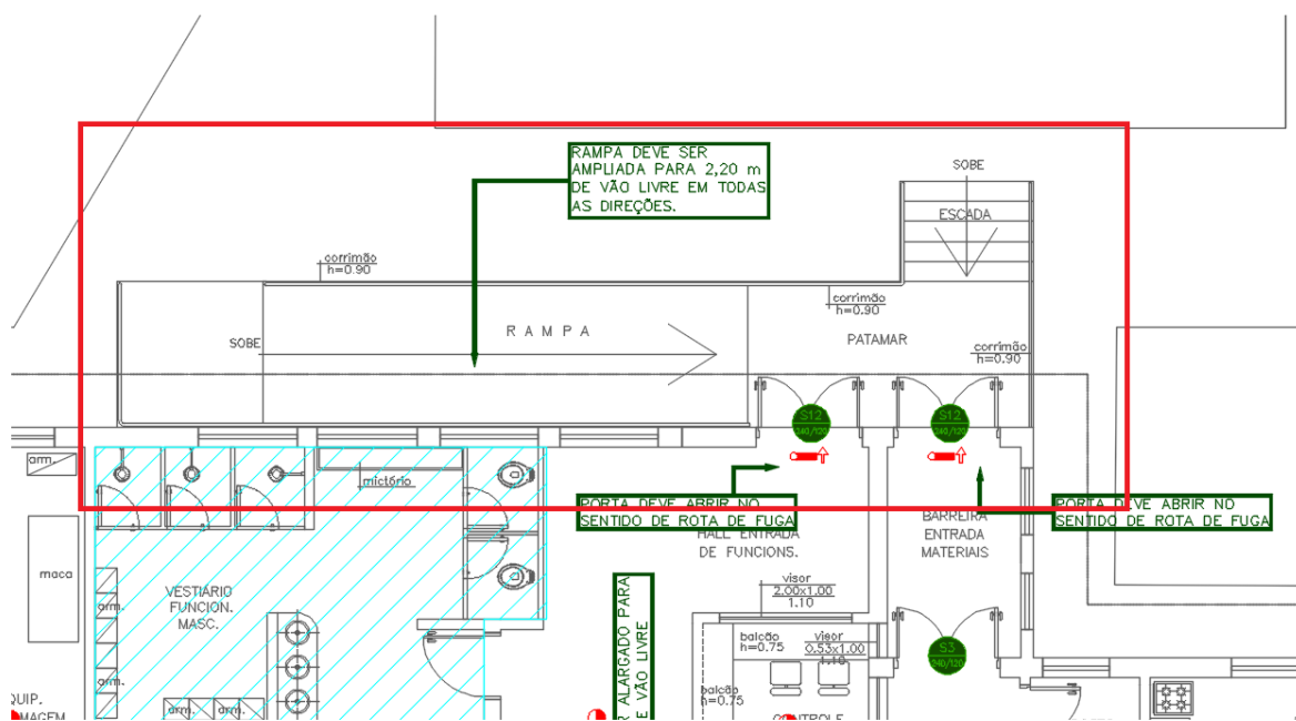
Figura 33 – PRÉDIO CCC – RAMPA 1 – NOVO LAYOUT DA RAMPA + ESCADA
