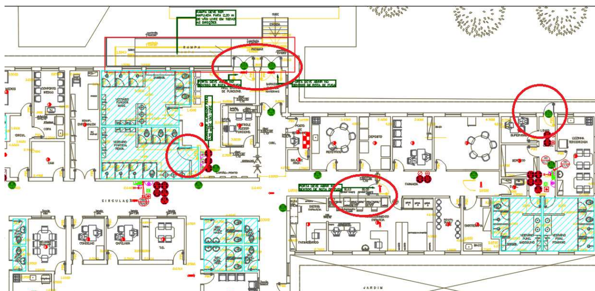
Figura 5 – PRÉDIO CCI - PAVIMENTO TÉRREO – Inversão sentido de porta
