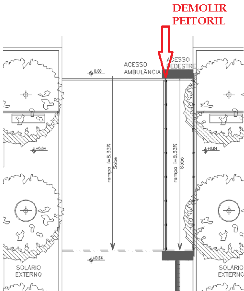
Figura 41 – PRÉDIO CPI – RAMPA 1 – RAMPA EXISTENTE
