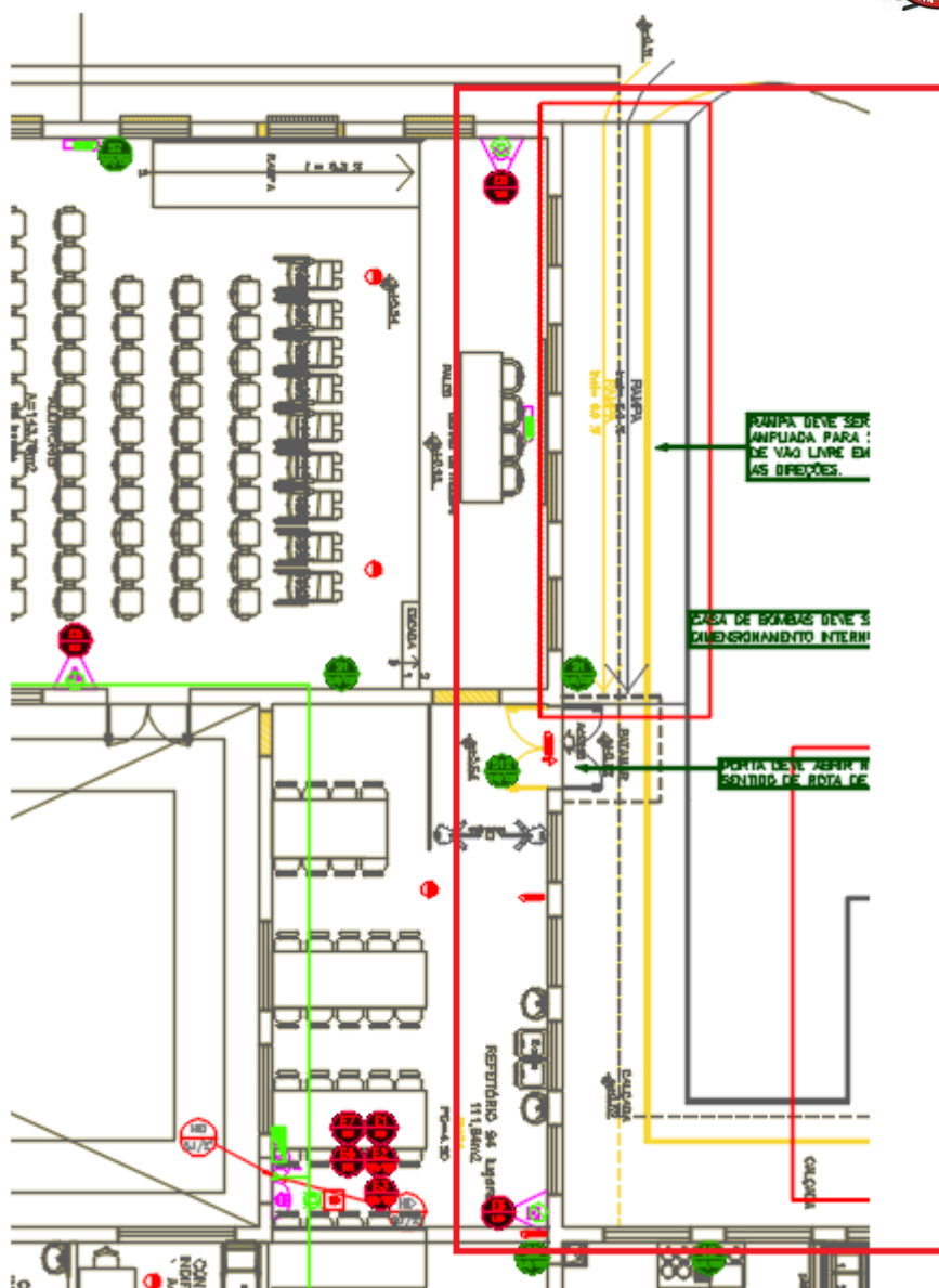
Figura 58 – PRÉDIO FISIOTERAPIA/AMBULATÓRIO/AUDITÓRIO – RAMPA+CALÇADA 1 – SOBREPOSIÇÃO RAMPA EXISTENTE (amarelo) x NOVO LAYOUT DA RAMPA
