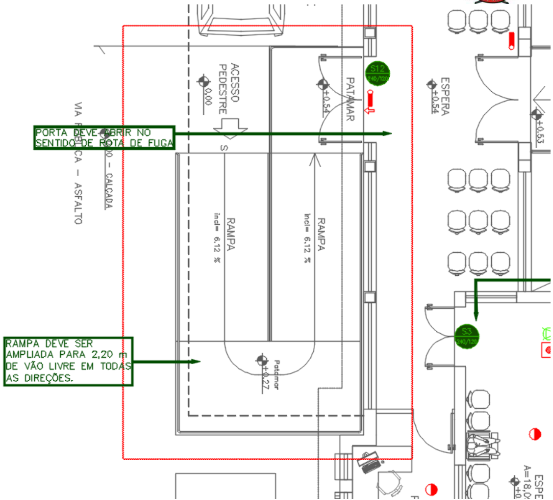
Figura 66 – PRÉDIO FISIOTERAPIA/AMBULATÓRIO/AUDITÓRIO – RAMPA 4 – NOVO LAYOUT DO ALARGAMENTO
