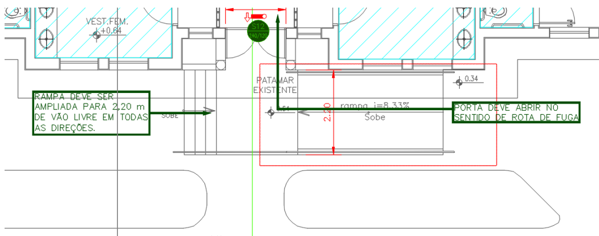
Figura 45 – PRÉDIO CPI – RAMPA 2 – NOVO LAYOUT DO ALARGAMENTO DA RAMPA/ESCALADA
