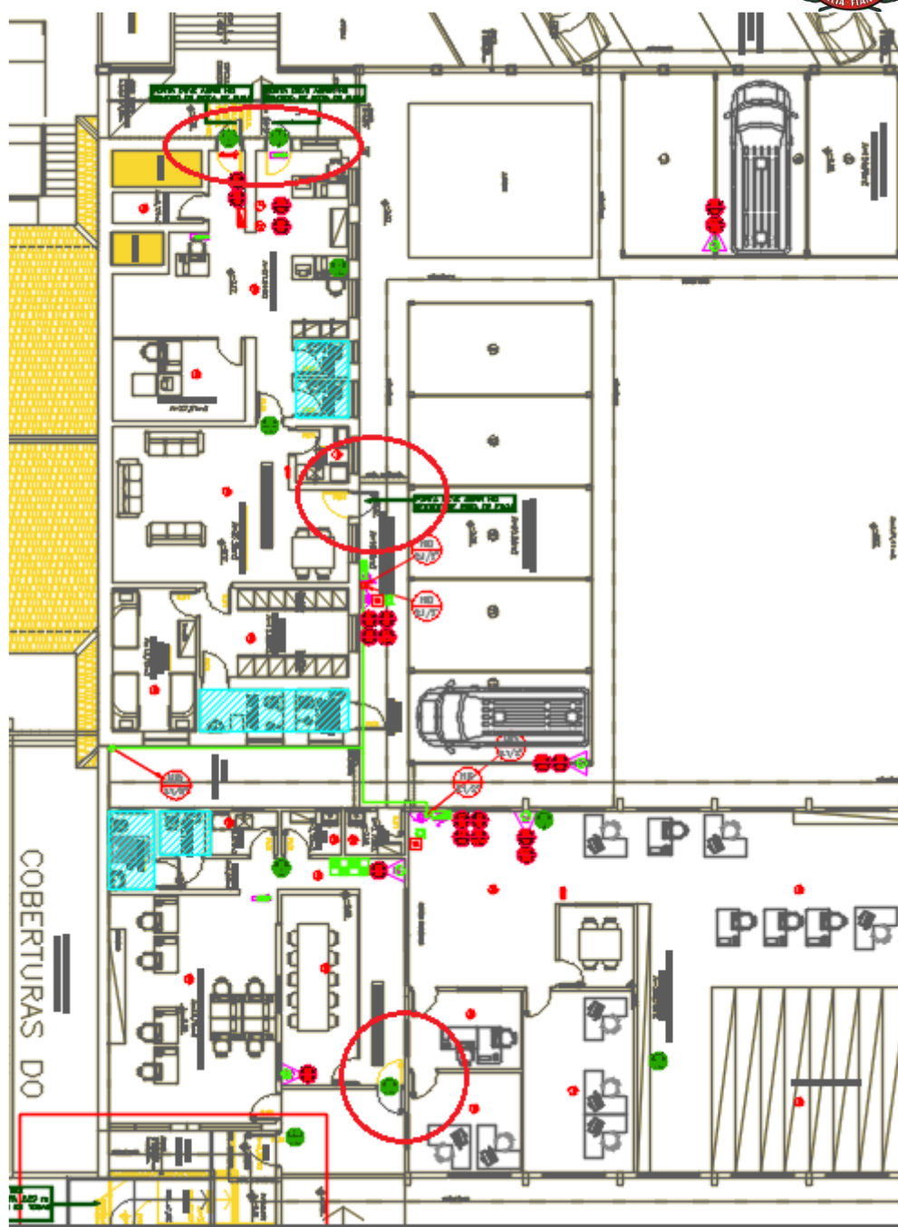
Figura 15 – PRÉDIO FROTA E PATRIMÔNIO - PAVIMENTO TÉRREO – Inversão sentido de porta
