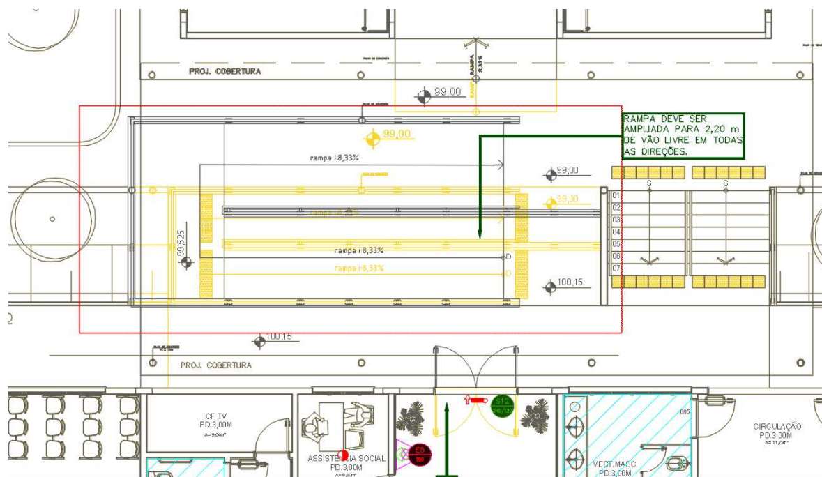
Figura 40 – PRÉDIO CER – RAMPA 1 – SOBREPOSIÇÃO RAMPA Á DEMOLIR (AMARELO) x NOVO LAYOUT DA RAMPA
