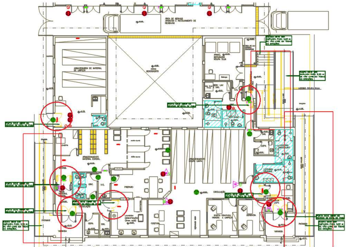
Figura 11 – PRÉDIO LAVANDERIA - PAVIMENTO TÉRREO – Inversão sentido de porta
