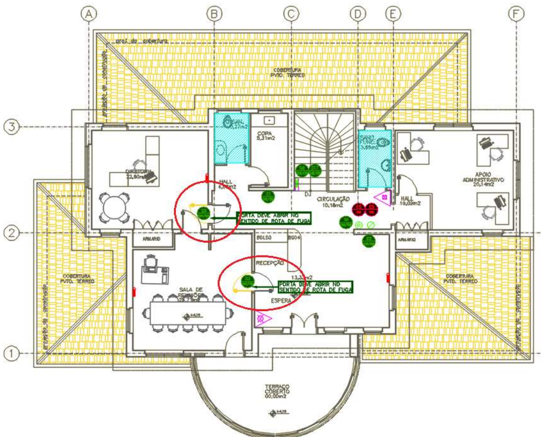
Figura 2 – PRÉDIO CASTELINHO - PAVIMENTO TÉRREO – Inversão sentido de porta
