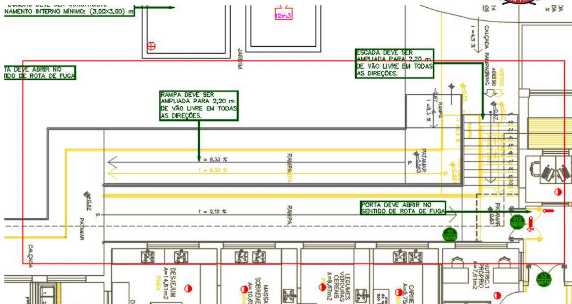
Figura 61 – PRÉDIO FISIOTERAPIA/AMBULATÓRIO/AUDITÓRIO – RAMPA+ESCALADA 2 – SOBREPOSIÇÃO RAMPA À DEMOLIR (AMARELO) x NOVO LAYOUT DA RAMPA
