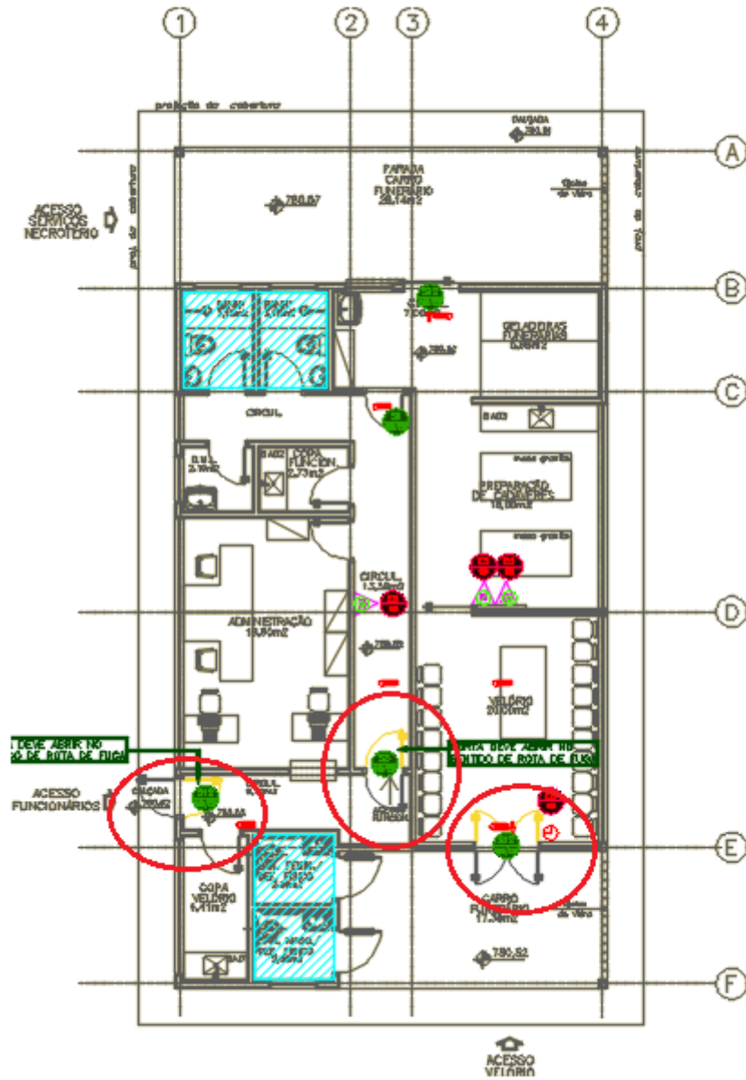
Figura 12 – PRÉDIO NECROTÉRIO - PAVIMENTO TÉRREO – Inversão sentido de porta
