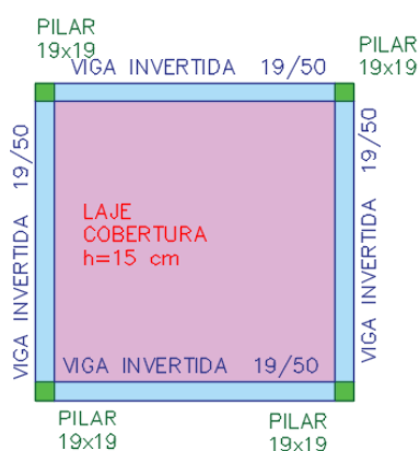
Figura 36 – PRÉDIO CER - RESERVA DE INCÊNDIO E CASA DE BOMBAS - PLANTA ESTRUTURAL DA FUNDAÇÃO
