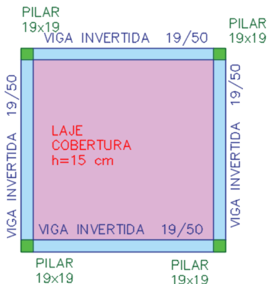
Figura 19 – PRÉDIO CCC - CASA DE BOMBAS - PLANTA ESTRUTURAL DA COBERTURA
