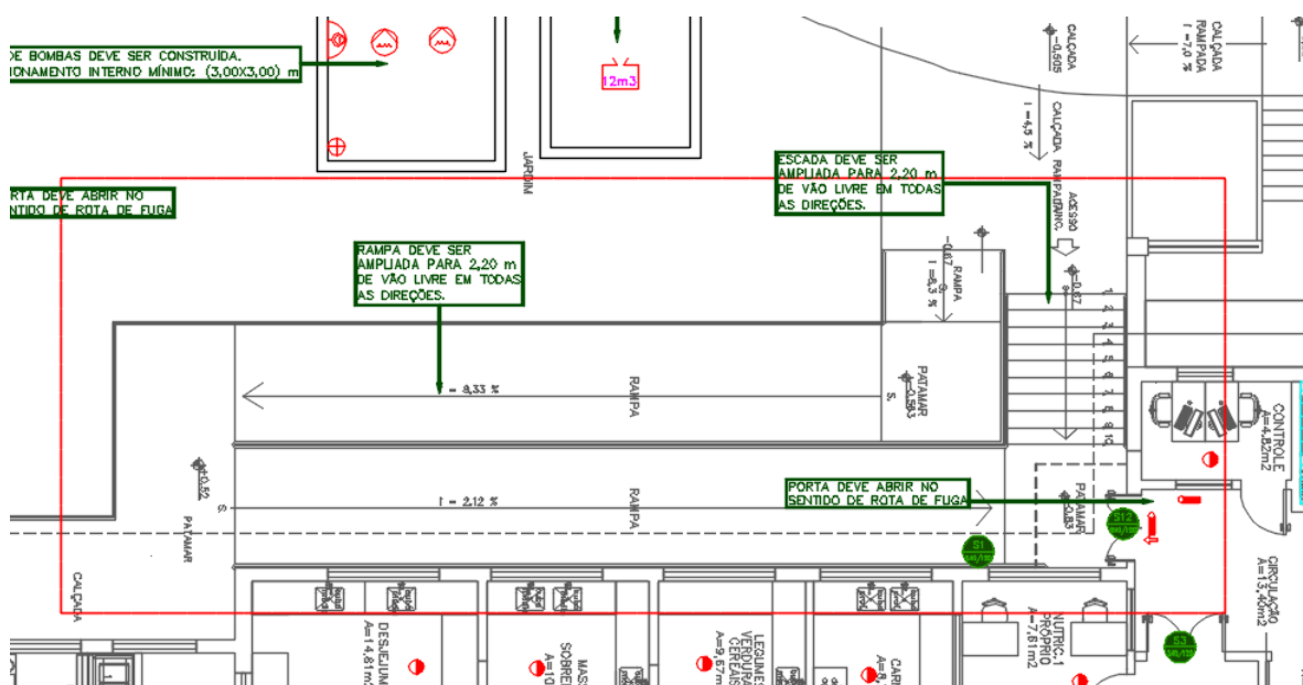
Figura 60 – PRÉDIO FISIOTERAPIA/AMBULATÓRIO/AUDITÓRIO – RAMPAS+ESCADA 2 – NOVO LAYOUT DA RAMPAS
