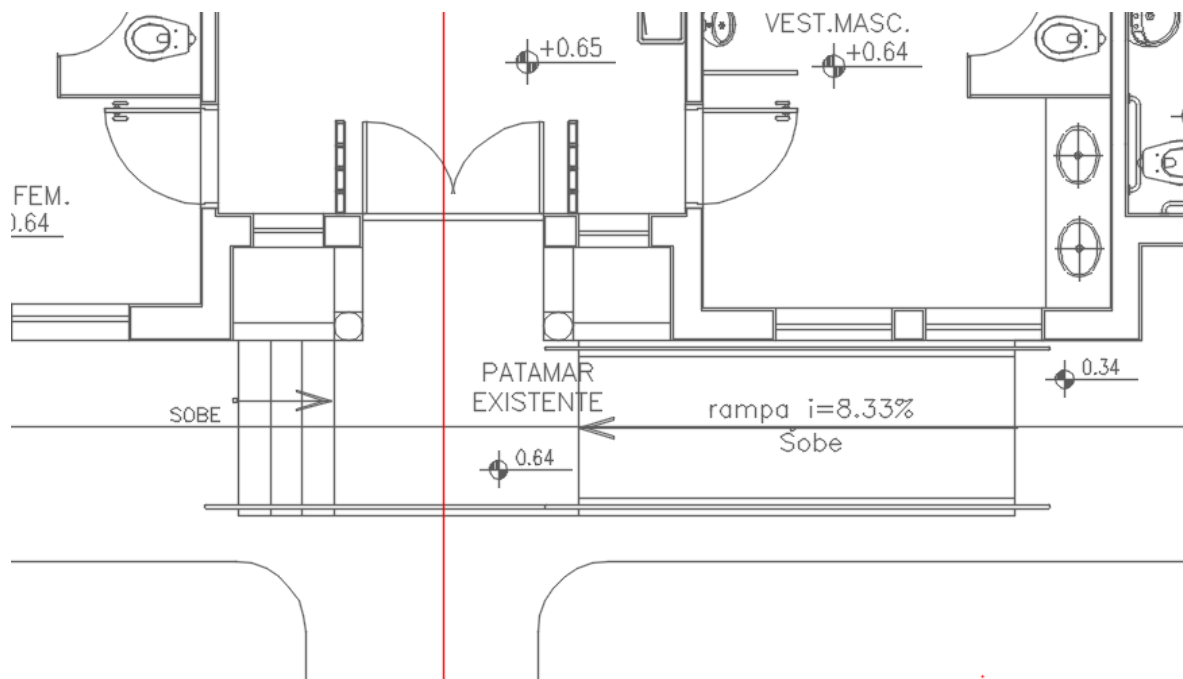
Figura 44 – PRÉDIO CPI – RAMPA 2 – RAMPA EXISTENTE
