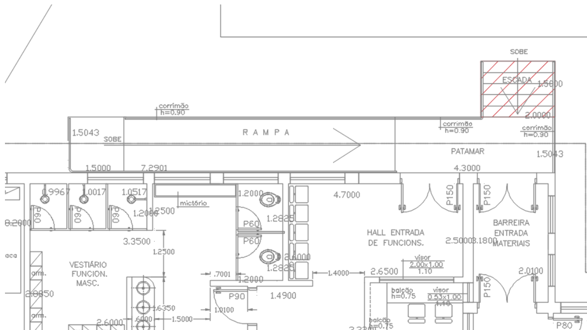
Figura 32 – PRÉDIO CCI – RAMPA + ESCADA 1 – Á DEMOLIR
