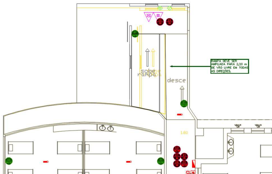
Figura 22 – PRÉDIO CCC – RAMPA 1 – SOBREPOSIÇÃO RAMPA Á DEMOLIR (AMARELO) x NOVO LAYOUT DA RAMPA
