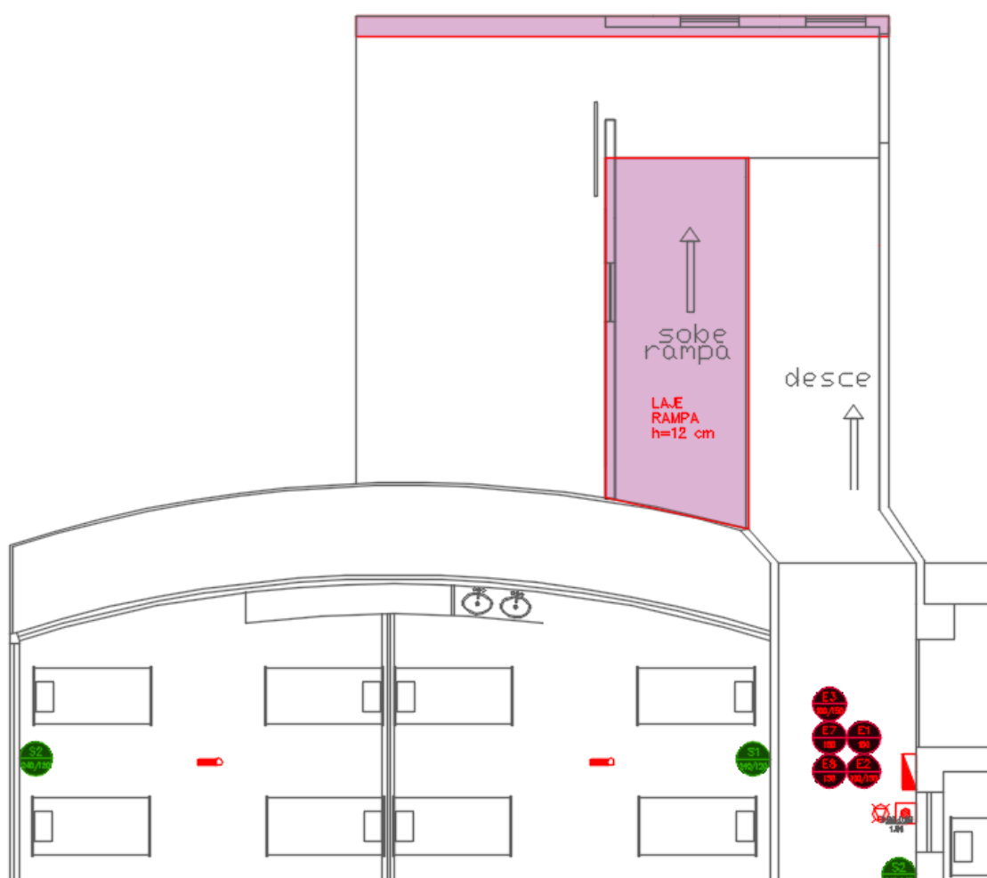
Figura 23 – PRÉDIO CCC - ESTRUTURA DA RAMPA 1 - EST x ARQ
