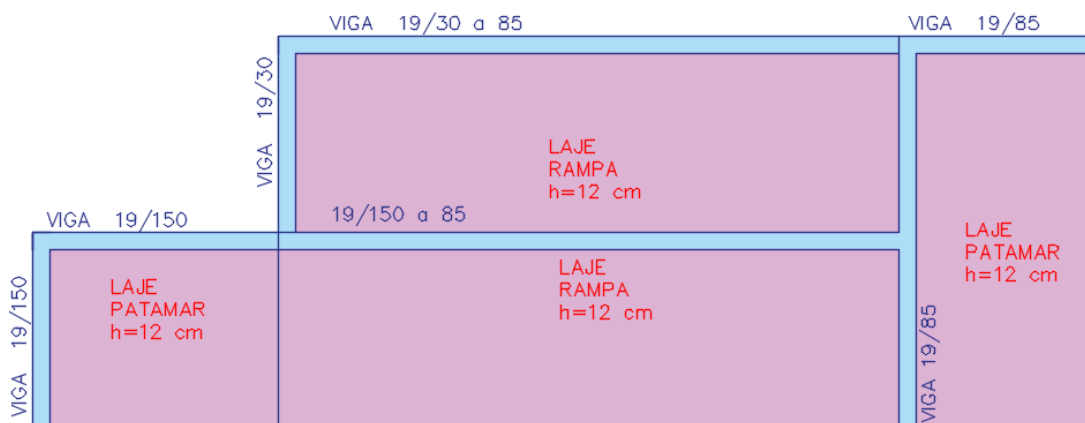
Figura 27 – PRÉDIO CCC - RAMPA 2 - PLANTA DE ESTRUTURA
