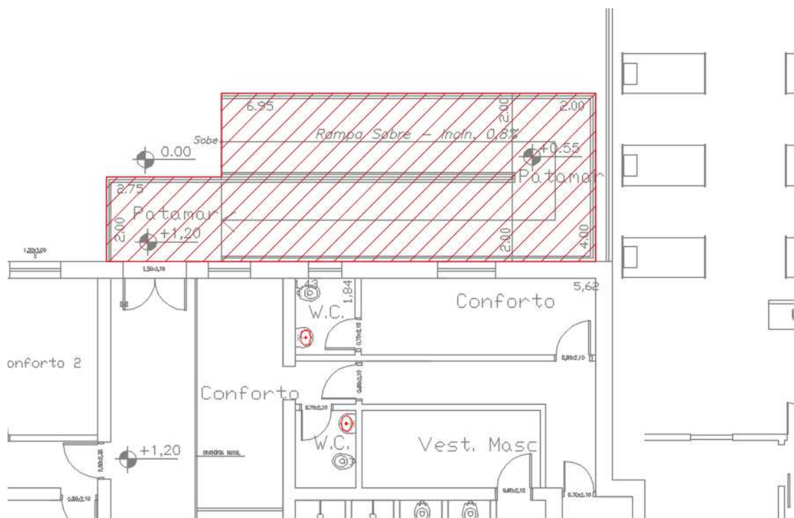
Figura 24 – PRÉDIO CCC – RAMPA 2 – Á DEMOLIR
