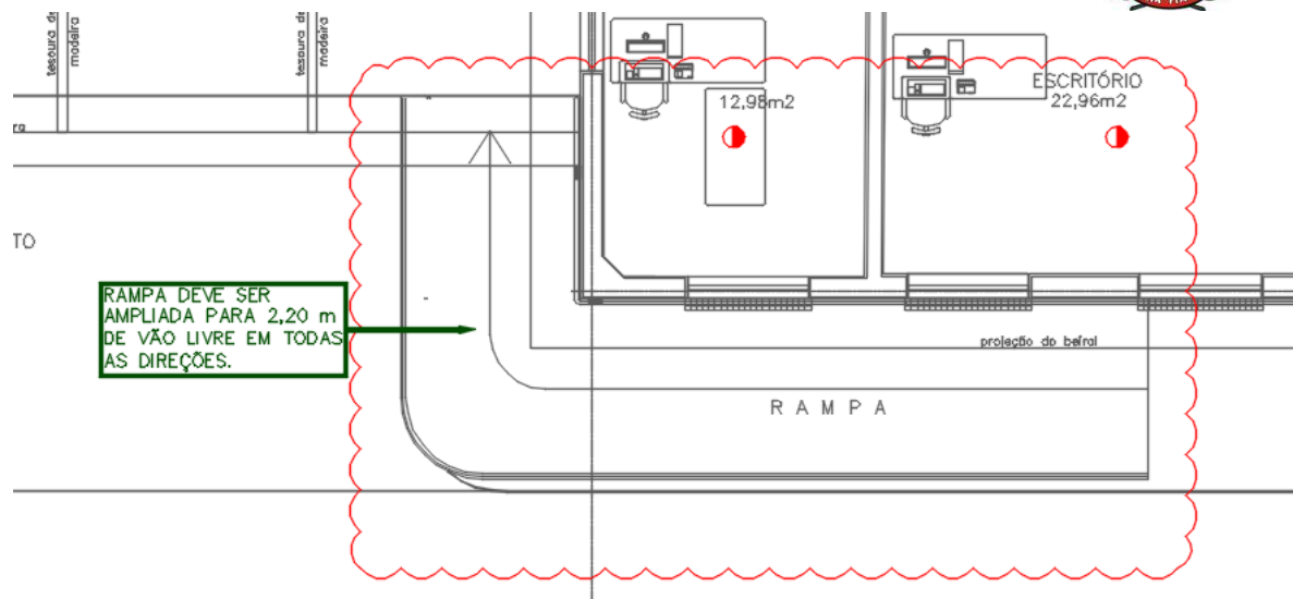
Figura 75 – PRÉDIO SUPRIMENTOS – RAMPA – NOVO LAYOUT
