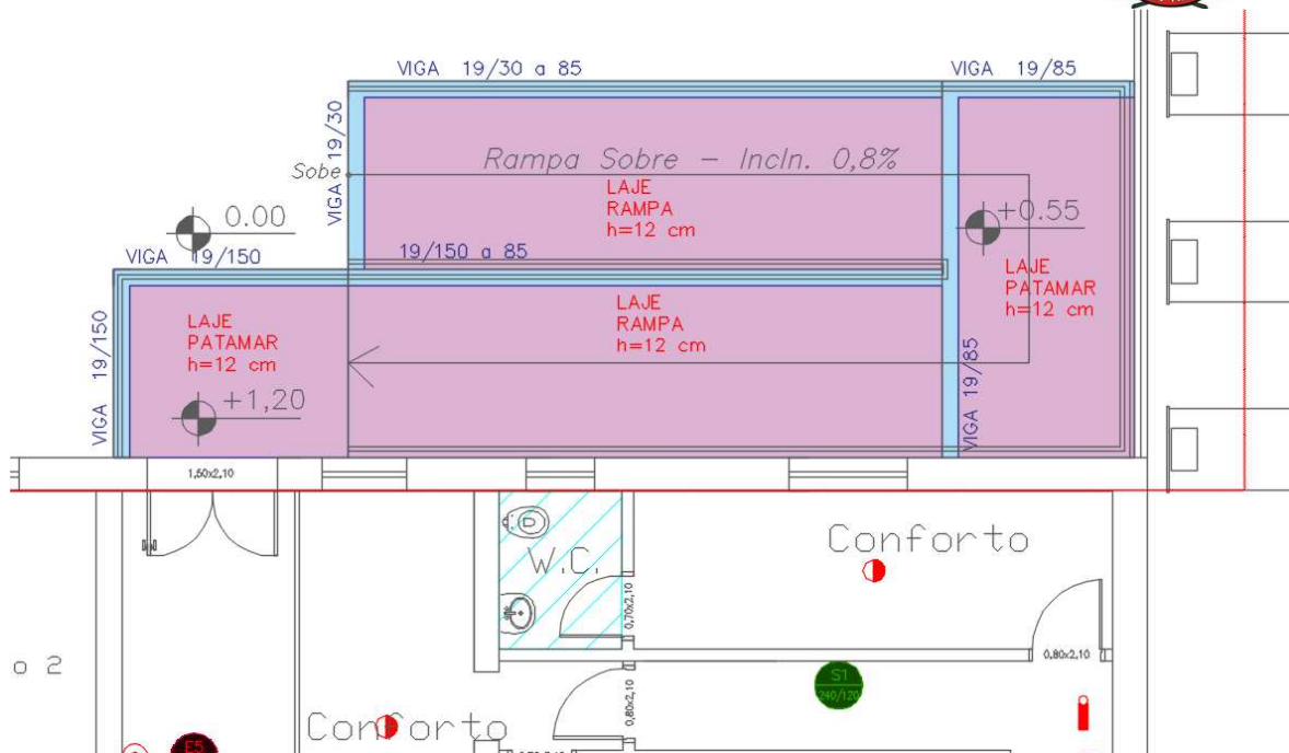
Figura 28 – PRÉDIO CCC - ESTRUTURA DA RAMPA 2 - EST x ARQ
