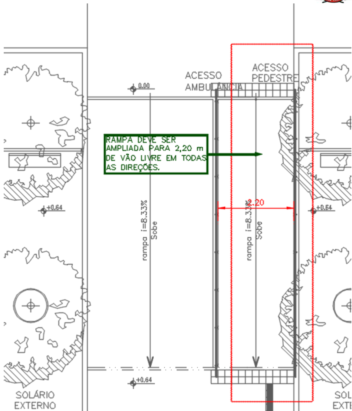
Figura 42 – PRÉDIO CPI – RAMPA 1 – NOVO LAYOUT DA RAMPA
