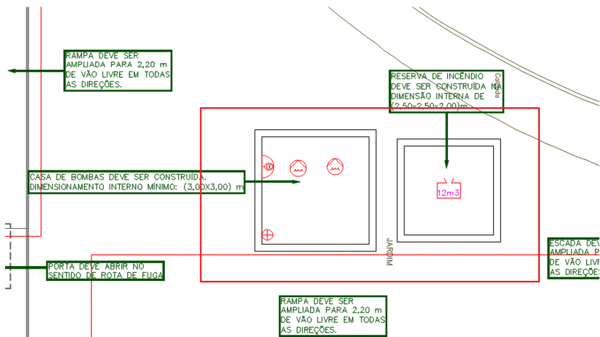
Figura 53 – PRÉDIO FISIOTERAPIA/AMBULATÓRIO/AUDITÓRIO – RESERVA DE INCÊNDIO E CASA DE BOMBAS - LAYOUT ARQUITETURA
