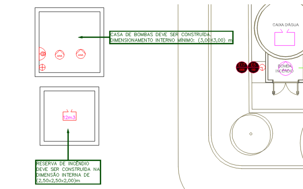
Figura 35 – PRÉDIO CER - RESERVA DE INCÊNDIO E CASA DE BOMBAS - LAYOUT ARQUITETURA
