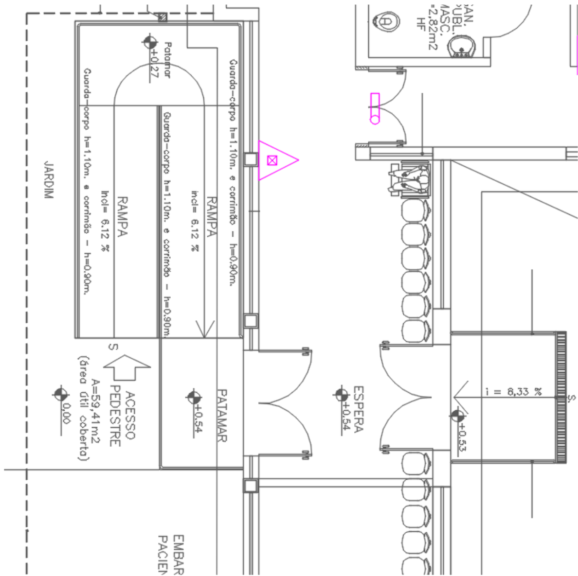
Figura 62 – PRÉDIO FISIOTERAPIA/AMBULATÓRIO/AUDITÓRIO – RAMPA 3 – RAMPA EXISTENTE
