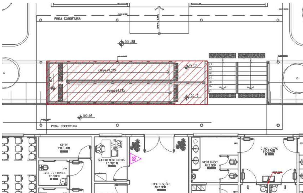
Figura 38 – PRÉDIO CER – RAMPA 1 – Á DEMOLIR
