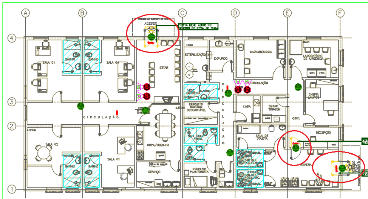
Figura 10 – PRÉDIO LABORATÓRIO - PAVIMENTO TÉRREO – Inversão sentido de porta
