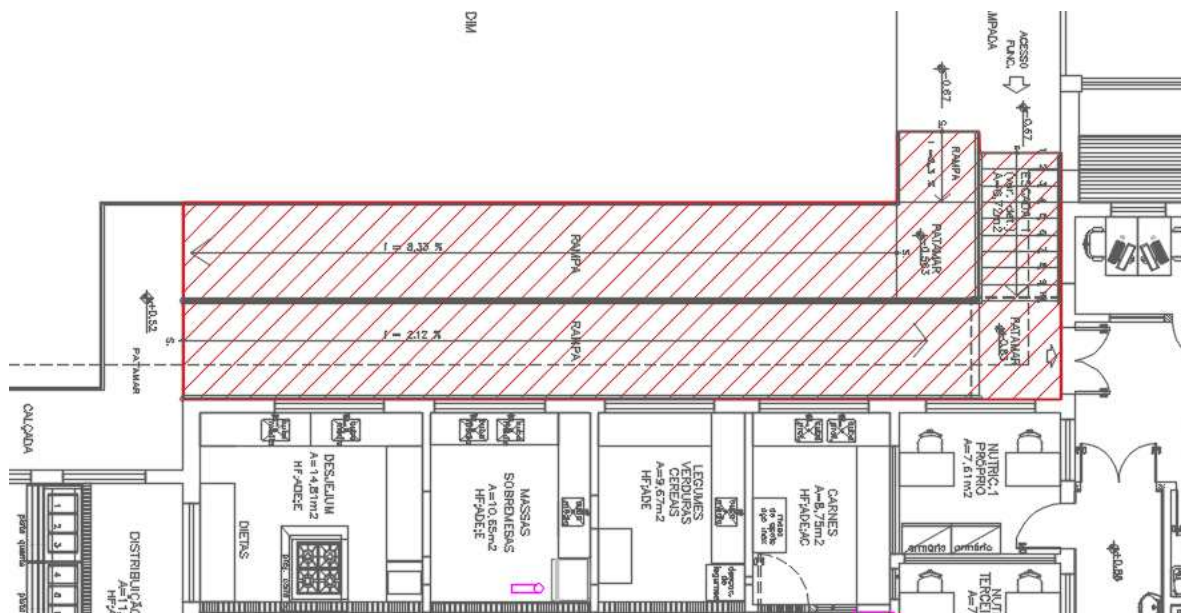
Figura 59 – PRÉDIO FISIOTERAPIA/AMBULATÓRIO/AUDITÓRIO – RAMPAS+ESCADA 2 – À DEMOLIR
