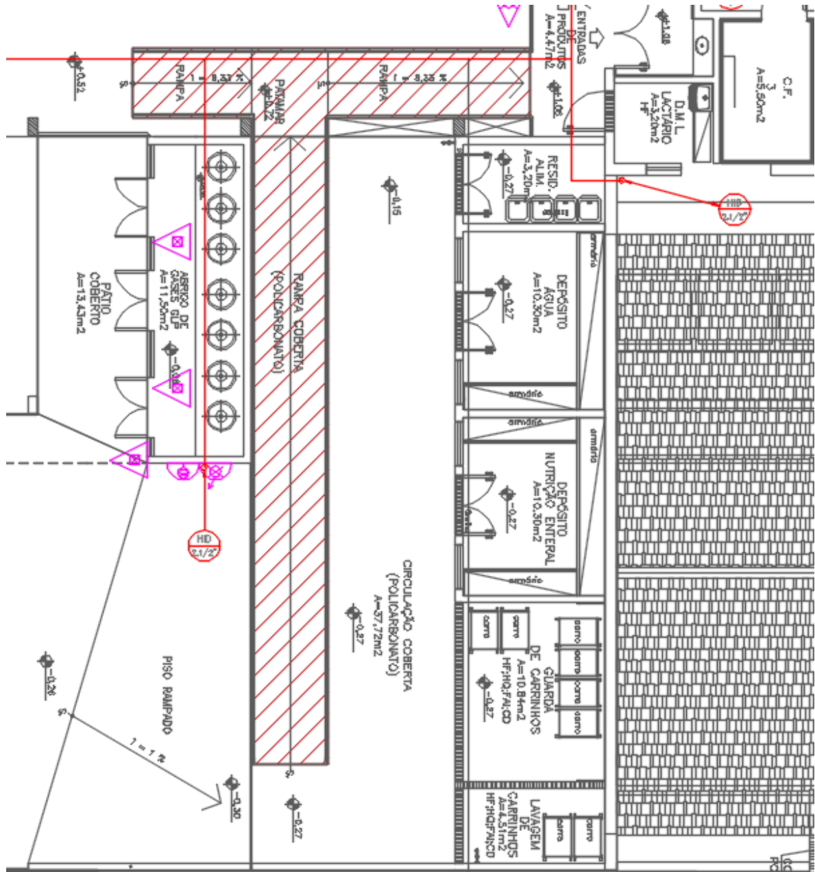
Figura 68 – PRÉDIO FISIOTERAPIA/AMBULATÓRIO/AUDITÓRIO – RAMPA 5 – Á DEMOLIR
