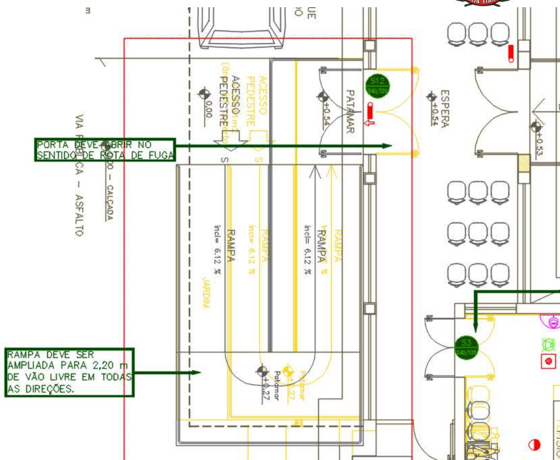
Figura 67 – PRÉDIO FISIOTERAPIA/AMBULATÓRIO/AUDITÓRIO – RAMPA 4 – SOBREPOSIÇÃO RAMPA EXISTENTE (amarelo) x NOVO LAYOUT DA RAMPA
