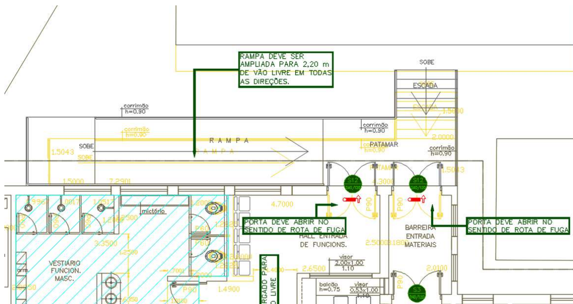
Figura 34 – PRÉDIO CCC – RAMPA 1 – SOBREPOSIÇÃO RAMPA E ESCADA ANTIGA (AMARELO) x NOVO LAYOUT DA RAMPA E ESCADA
