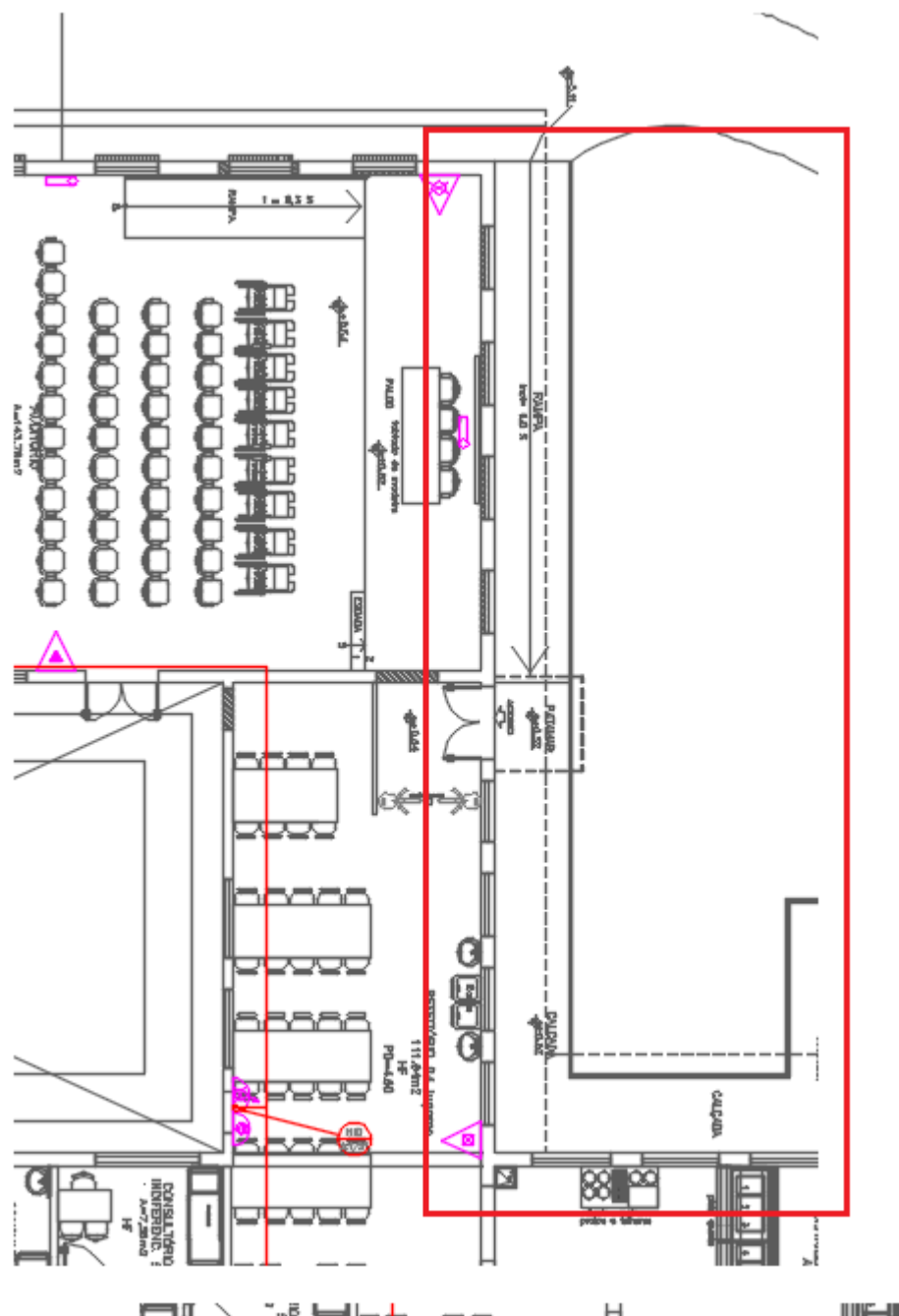
Figura 56 – PRÉDIO FISIOTERAPIA/AMBULATÓRIO/AUDITÓRIO – RAMPA 1 – RAMPA+CALÇADA EXISTENTE
