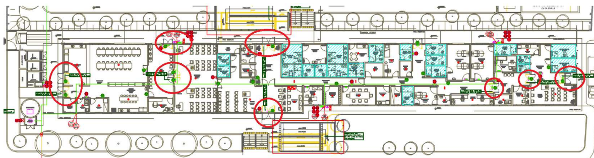
Figura 8 – PRÉDIO CER - PAVIMENTO TÉRREO – Inversão sentido de porta
