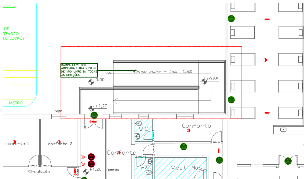
Figura 25 – PRÉDIO CCC – RAMPA 2 – NOVO LAYOUT DA RAMPA
