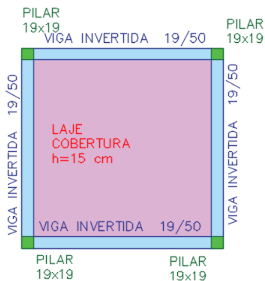
Figura 54 – PRÉDIO FISIOTERAPIA/AMBULATÓRIO/AUDITÓRIO - PLANTA ESTRUTURAL DA FUNDAÇÃO
