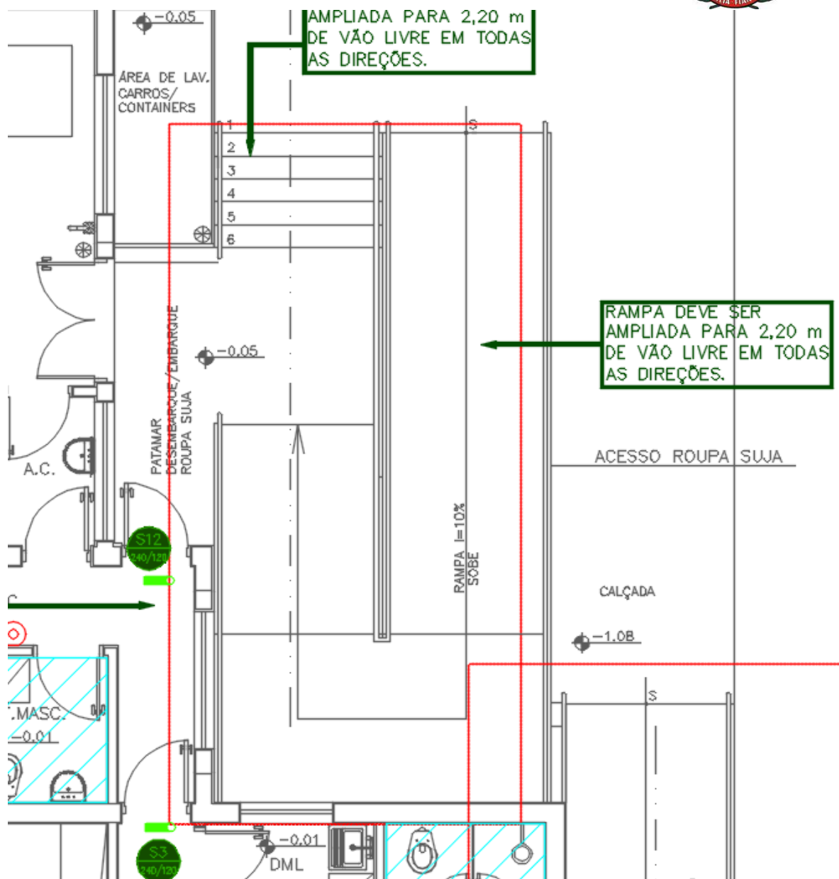
Figura 48 – PRÉDIO LAVANDERIA – RAMPA E ESCADA 1 – NOVO LAYOUT DA RAMPA
