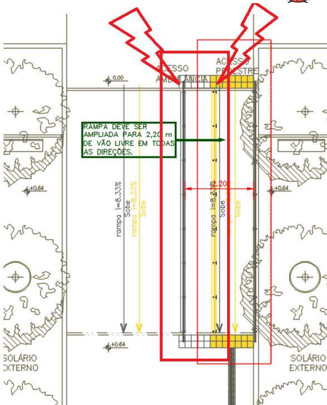
Figura 43 – PRÉDIO CPI – RAMPA 1 – SOBREPOSIÇÃO RAMPA EXISTENTE (amarelo) x NOVO LAYOUT DA RAMPA
