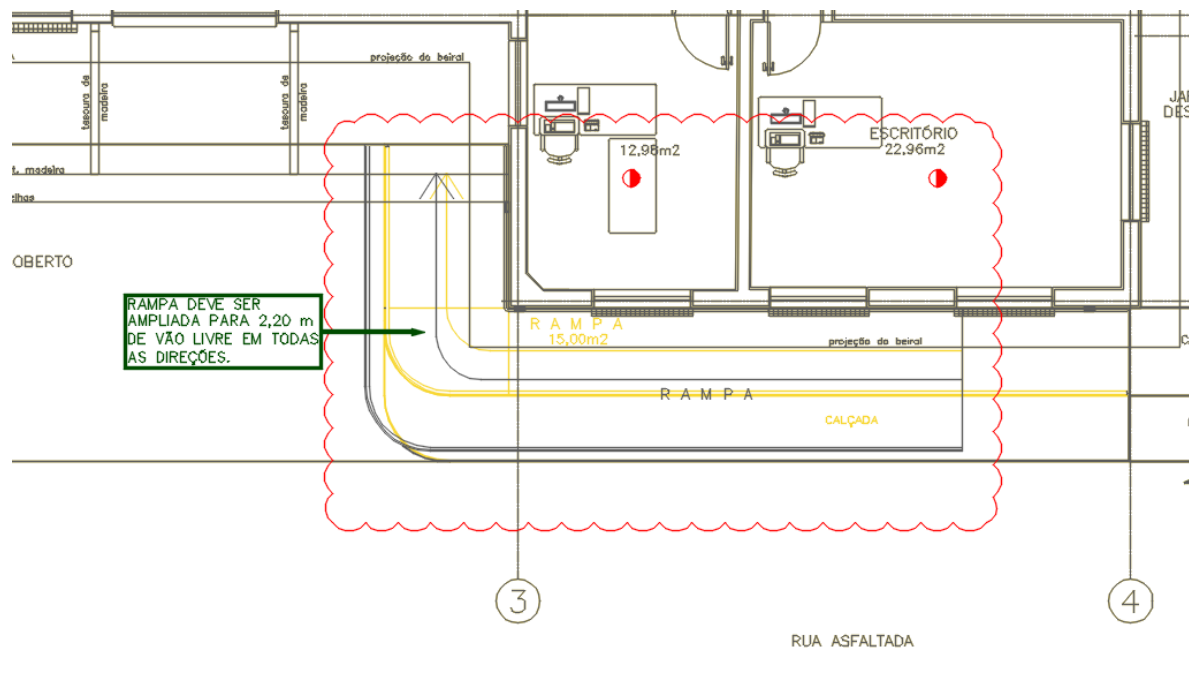
Figura 75 – PRÉDIO SUPRIMENTOS – RAMPA – NOVO LAYOUT
