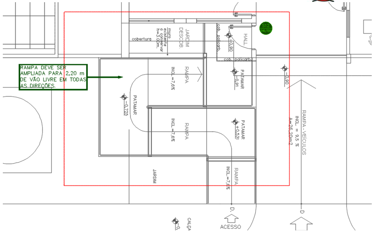
Figura 72 – PRÉDIO FROTA E PATRIMÔNIO – RAMPA – NOVO LAYOUT
