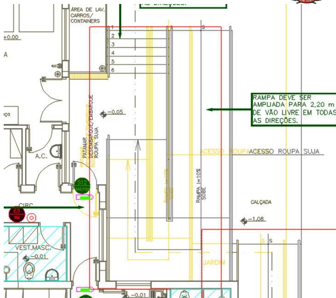
Figura 49 – PRÉDIO LAVANDERIA – RAMPA E ESCADA 1 – SOBREPOSIÇÃO RAMPA Á DEMOLIR (AMARELO) x NOVO LAYOUT DA RAMPA
