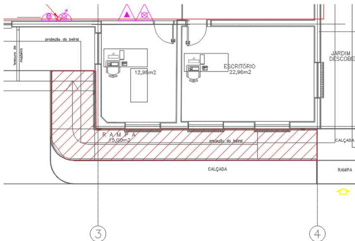
Figura 74 – PRÉDIO SUPRIMENTOS – RAMPA – RAMPA EXISTENTE Á DEMOLIR
