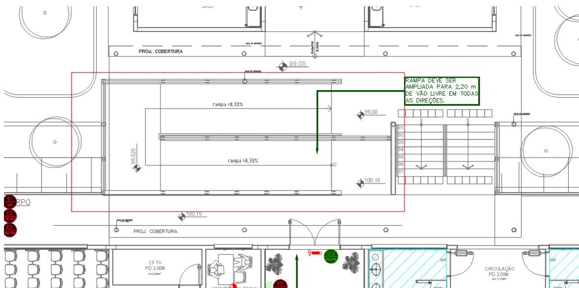
Figura 39 – PRÉDIO CER – RAMPA 1 – NOVO LAYOUT DA RAMPA
