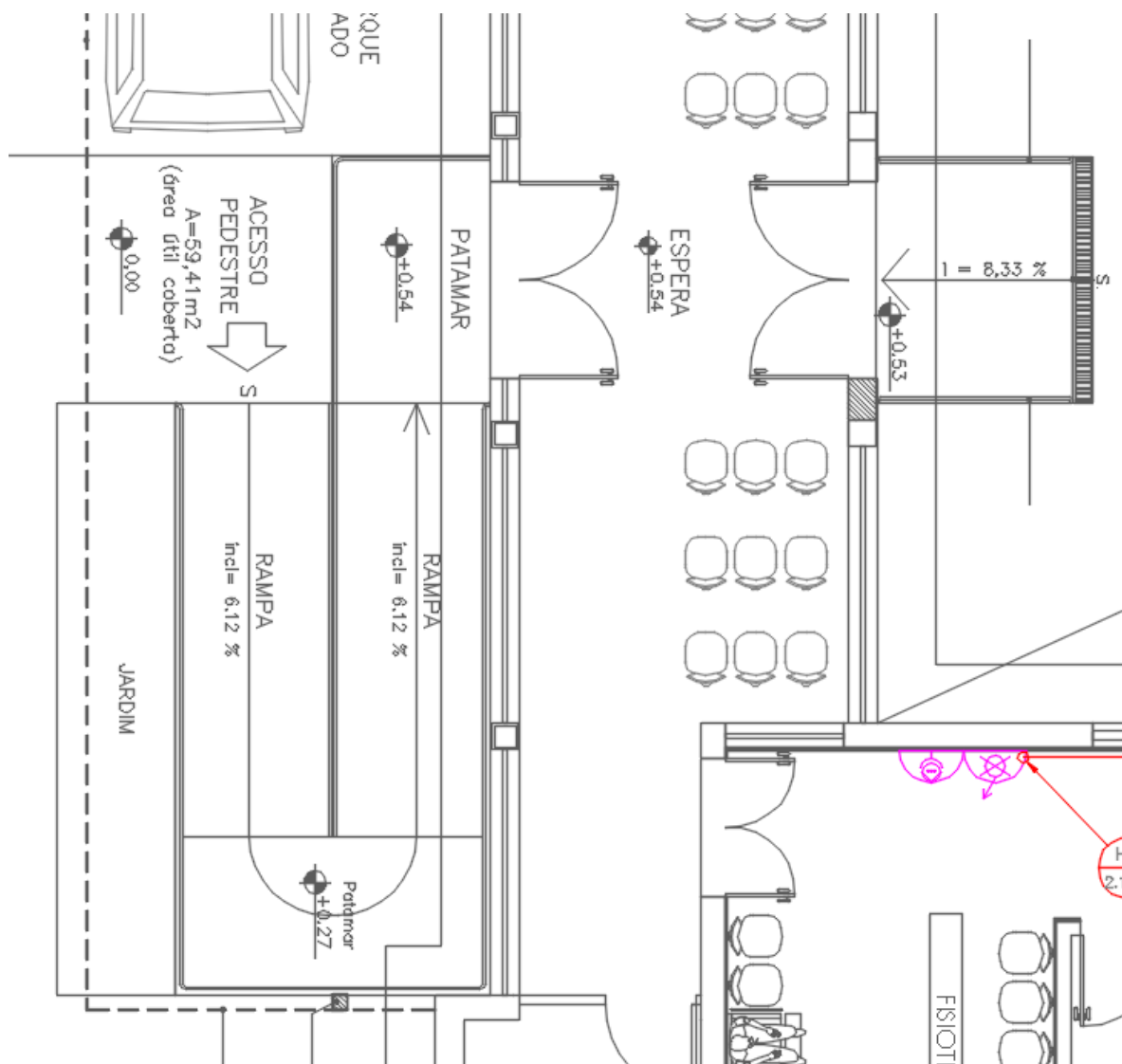
Figura 65 – PRÉDIO FISIOTERAPIA/AMBULATÓRIO/AUDITÓRIO – RAMPA 4 – RAMPA EXISTENTE
