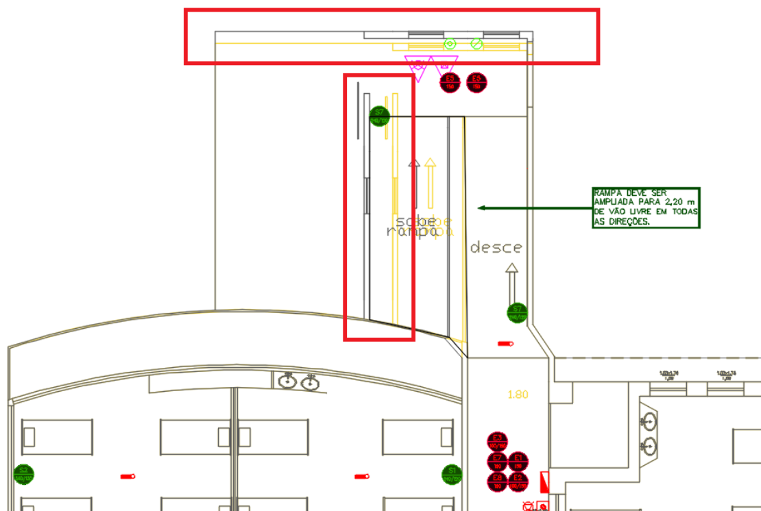
Figura 16 – PRÉDIO CCC – RAMPA 1 – Demolição/Reconstrução paredes
