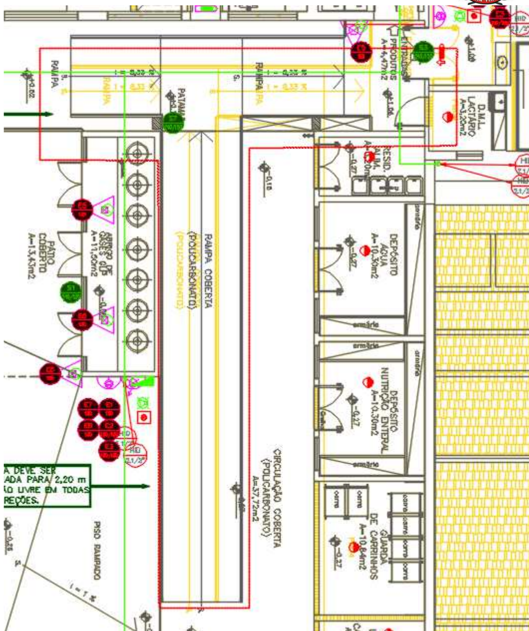
Figura 70 – PRÉDIO FISIOTERAPIA/AMBULATÓRIO/AUDITÓRIO – RAMPA 5 – SOBREPOSIÇÃO RAMPA Á DEMOLIR (AMARELO) x NOVO LAYOUT DA RAMPA
