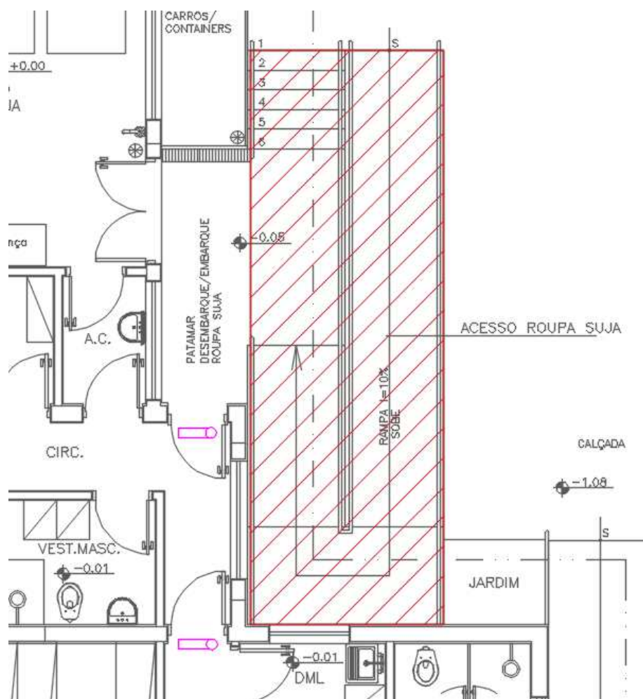
Figura 47 – PRÉDIO LAVANDERIA – RAMPA E ESCADA 1 – Á DEMOLIR
