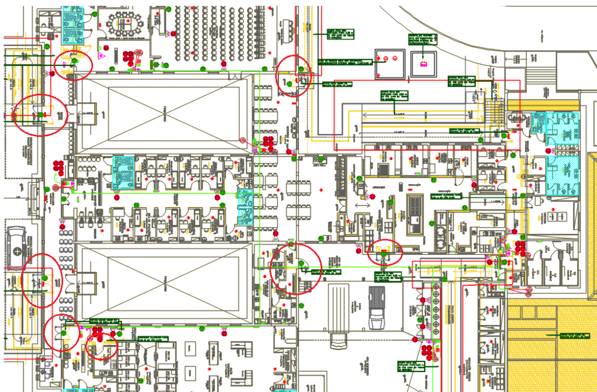
Figura 14 – PRÉDIO FISIOTERAPIA/AMBULATÓRIO E AUDITÓRIO - PAVIMENTO TÉRREO – Inversão sentido de porta
