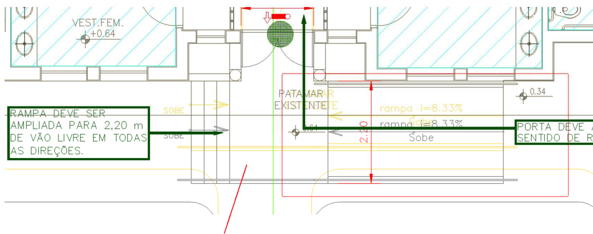
Figura 46 – PRÉDIO CPI – RAMPA 2 – SOBREPOSIÇÃO RAMPA EXISTENTE (amarelo) x NOVO LAYOUT DA RAMPA
