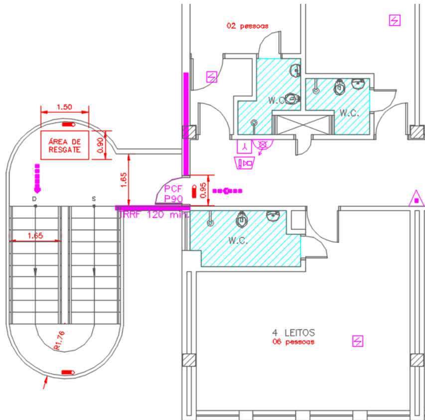
Figura 13 – PLANTA DA NOVA ESCADA METÁLICA 4 – SAÍDA DO 2ºPAVIMENTO AO 3º PAVIMENTO
