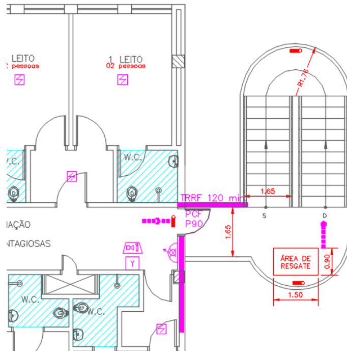
Figura 10 – PLANTA DA NOVA ESCADA METÁLICA 1 – SAÍDA DO 1ºPAVIMENTO AO 2º PAVIMENTO
