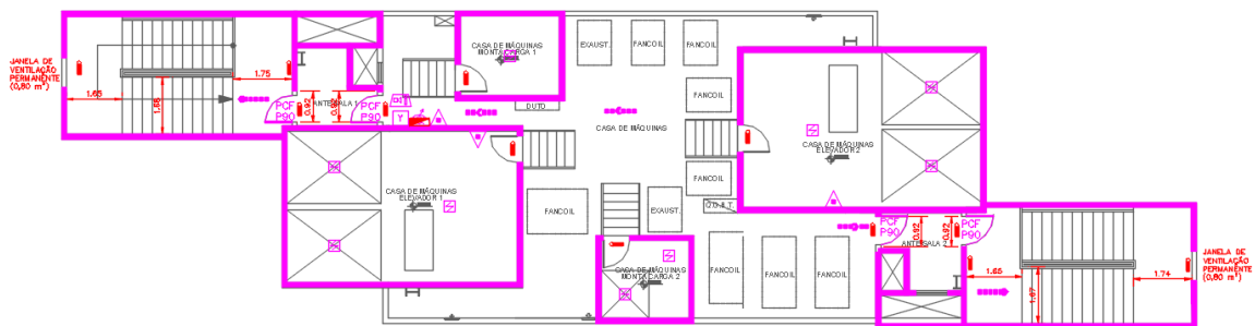
Figura 24 – PLANTA DA NOVA ESCADA DE CONCRETO 2 e 3 – CHEGADA A CASA DE MÁQUINAS
