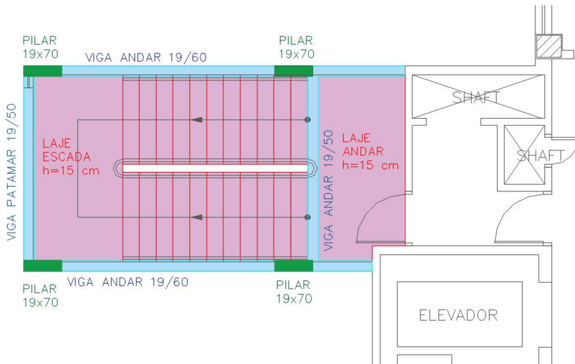
Figura 27 – ESTRUTURA TÍPICA DA NOVA ESCADA DE CONCRETO 2 – TÉRREO A CASA DE MÁQUINAS
