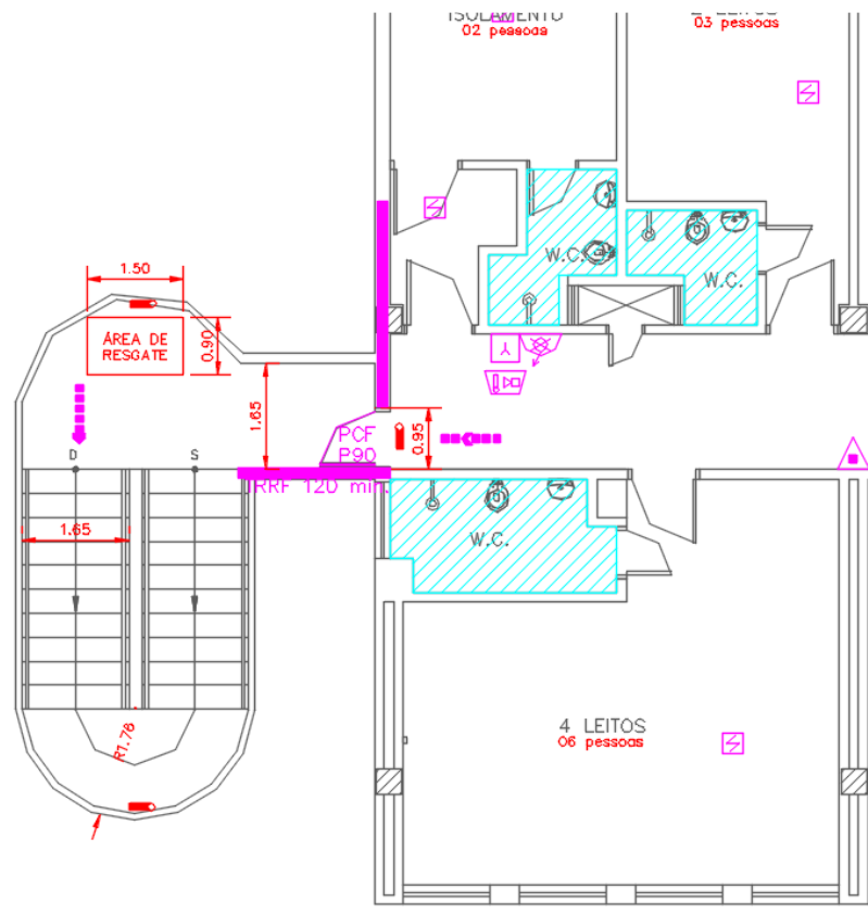
Figura 15 – PLANTA DA NOVA ESCADA METÁLICA 4 – SAÍDA DO 3ºPAVIMENTO AO 4º PAVIMENTO
