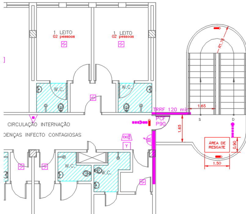
Figura 12 – PLANTA DA NOVA ESCADA METÁLICA 1 – SAÍDA DO 2ºPAVIMENTO AO 3º PAVIMENTO
