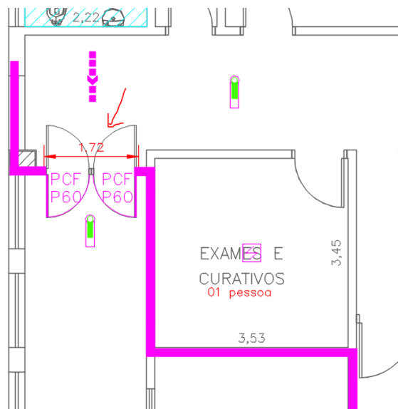
Figura 1 – EXEMPLO 1º PAVIMENTO – Inversão sentido de porta
