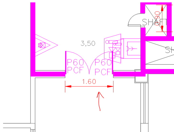
Figura 2 – EXEMPLO 1º PAVIMENTO – Instalação de porta corta-fogo na abertura existente
