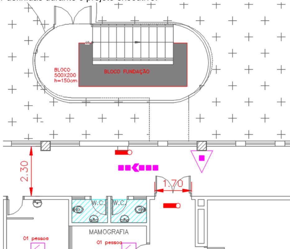
Figura 8 – PLANTA DA NOVA ESCADA METÁLICA 1 – SAÍDA DA ÁREA EXTERNA DO TÉRREO AO 1º PAVIMENTO – REPRESENTAÇÃO DO BLOCO ESTRUTURAL
