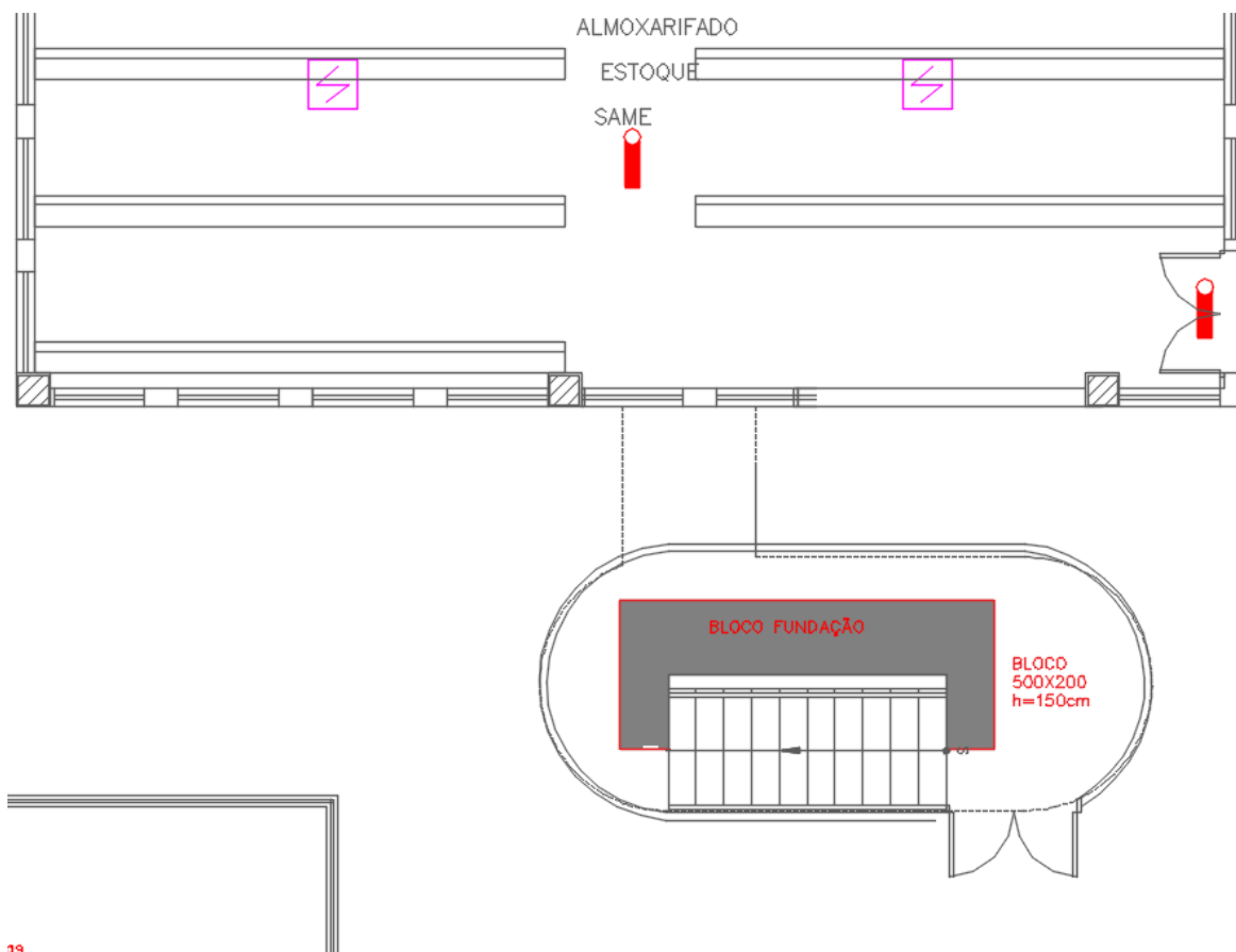
Figura 9 – PLANTA DA NOVA ESCADA METÁLICA 4 – SAÍDA DA ÁREA EXTERNA DO TÉRREO AO 1ºPAVIMENTO – REPRESENTAÇÃO DO BLOCO ESTRUTURAL
