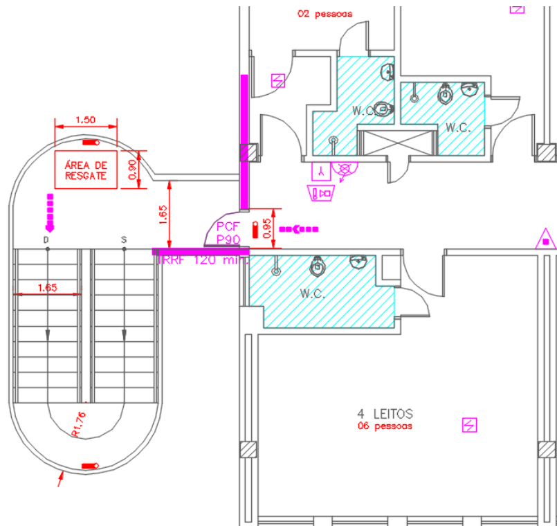
Figura 11 – PLANTA DA NOVA ESCADA METÁLICA 4 – SAÍDA DO 1ºPAVIMENTO AO 2º PAVIMENTO
