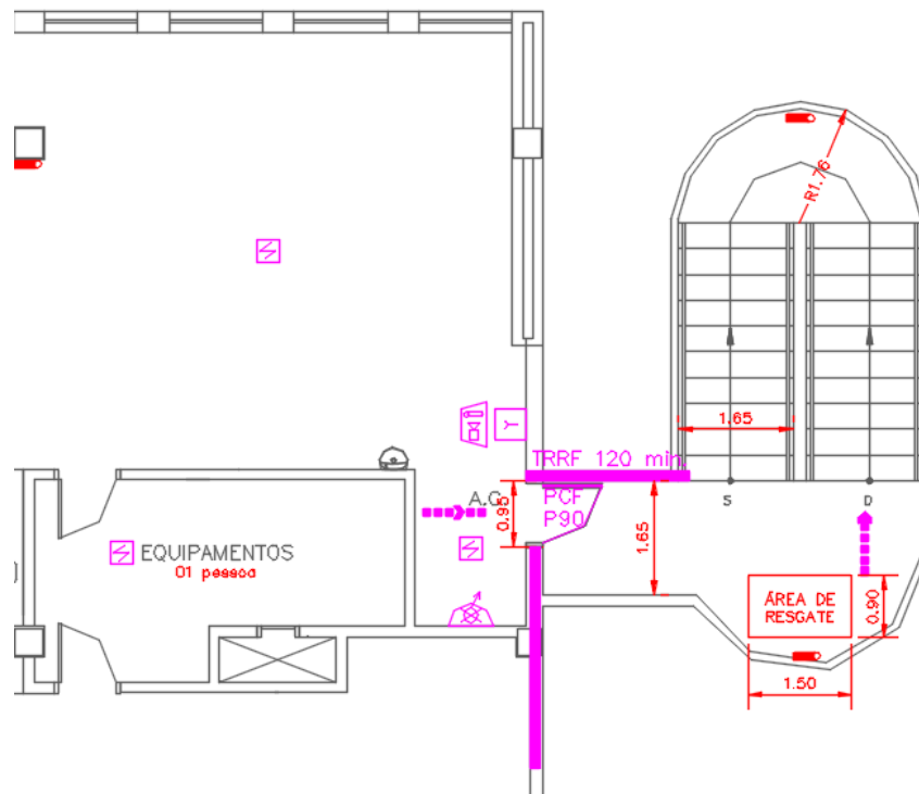
Figura 16 – PLANTA DA NOVA ESCADA METÁLICA 1 – SAÍDA DO 4º PAVIMENTO A COBERTURA
