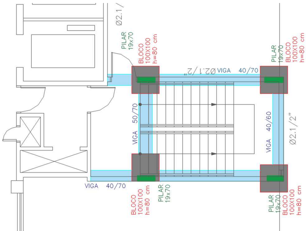
Figura 26 – ESTRUTURA DA NOVA ESCADA DE CONCRETO 3 – SAÍDA DA ÁREA EXTERNA DO TÉRREO AO 1º PAVIMENTO
