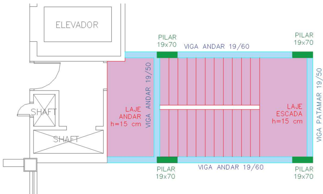
Figura 28 – ESTRUTURA TÍPICA DA NOVA ESCADA DE CONCRETO 2 –TÉRREO A CASA DE MÁQUINAS
