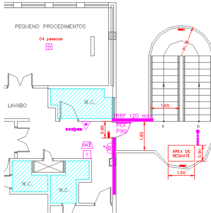
Figura 14 – PLANTA DA NOVA ESCADA METÁLICA 1 – SAÍDA DO 3ºPAVIMENTO AO 4º PAVIMENTO
