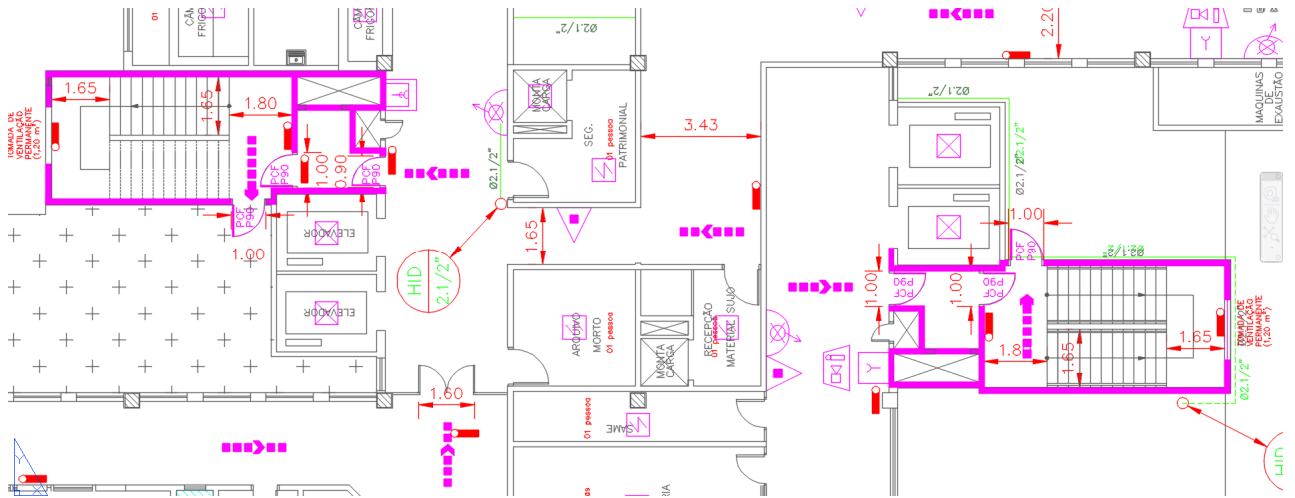
Figura 19 – PLANTA DA NOVA ESCADA DE CONCRETO 2 e 3 – SAÍDA DA ÁREA EXTERNA DO TÉRREO AO 1ºPAVIMENTO
