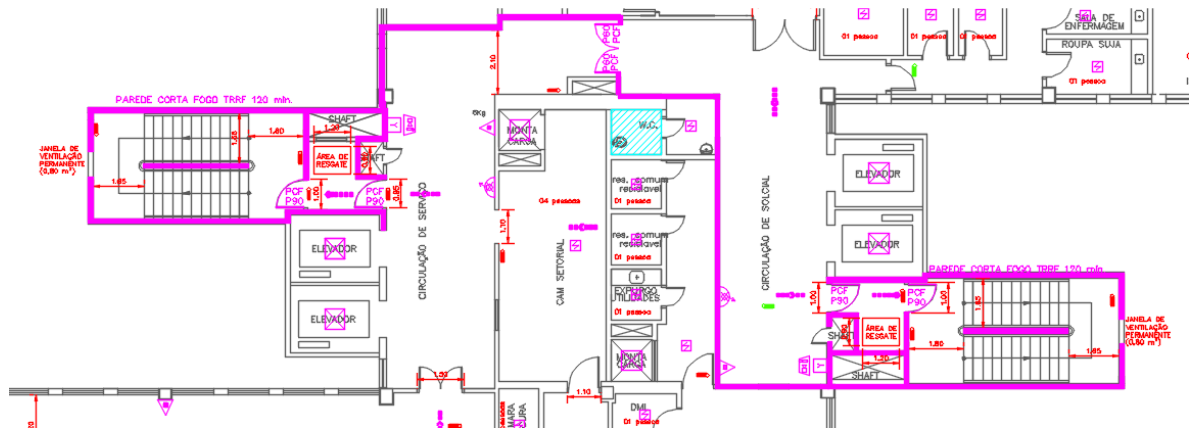
Figura 23 – PLANTA DA NOVA ESCADA DE CONCRETO 2 e 3 – SAÍDA DO 4º PAVIMENTO A COBERTURA
