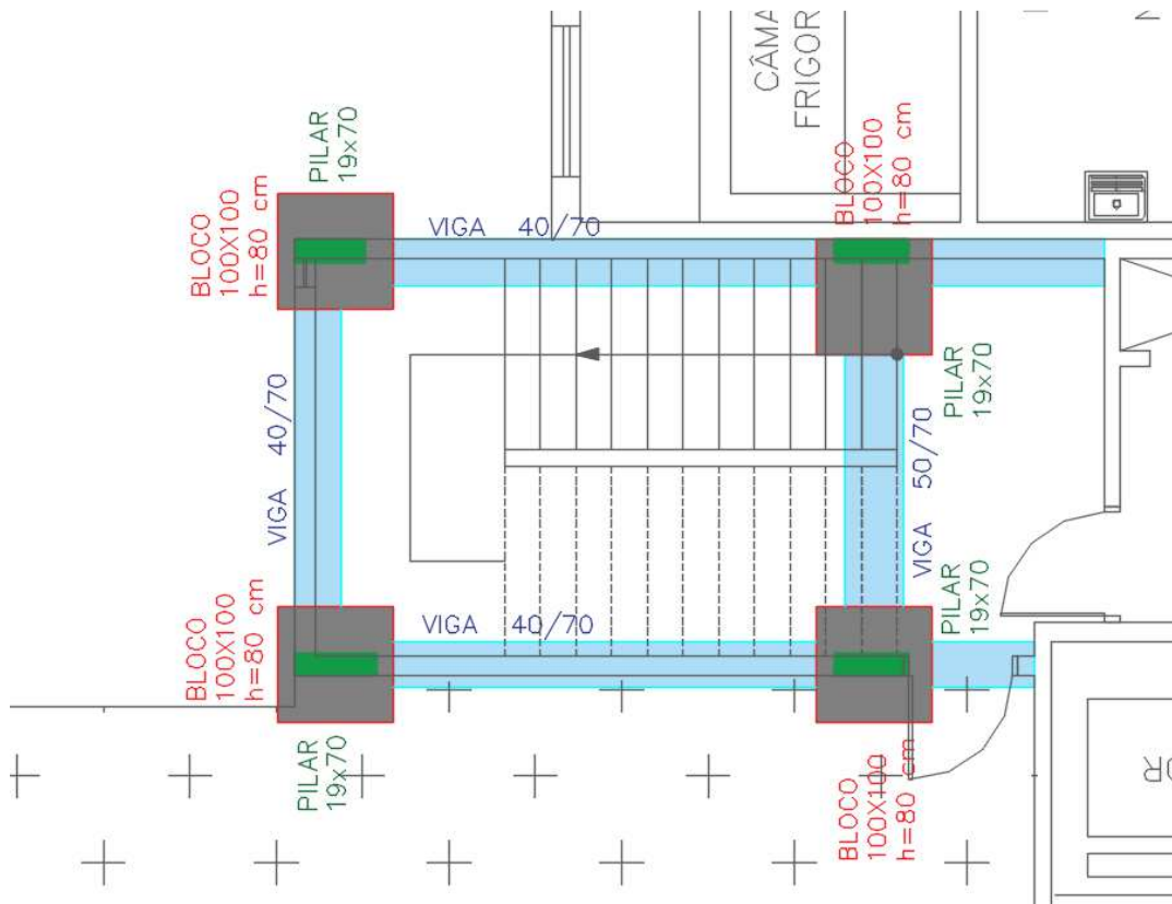
Figura 25 – ESTRUTURA DA NOVA ESCADA DE CONCRETO 2 – SAÍDA DA ÁREA EXTERNA DO TÉRREO AO 1ºPAVIMENTO
