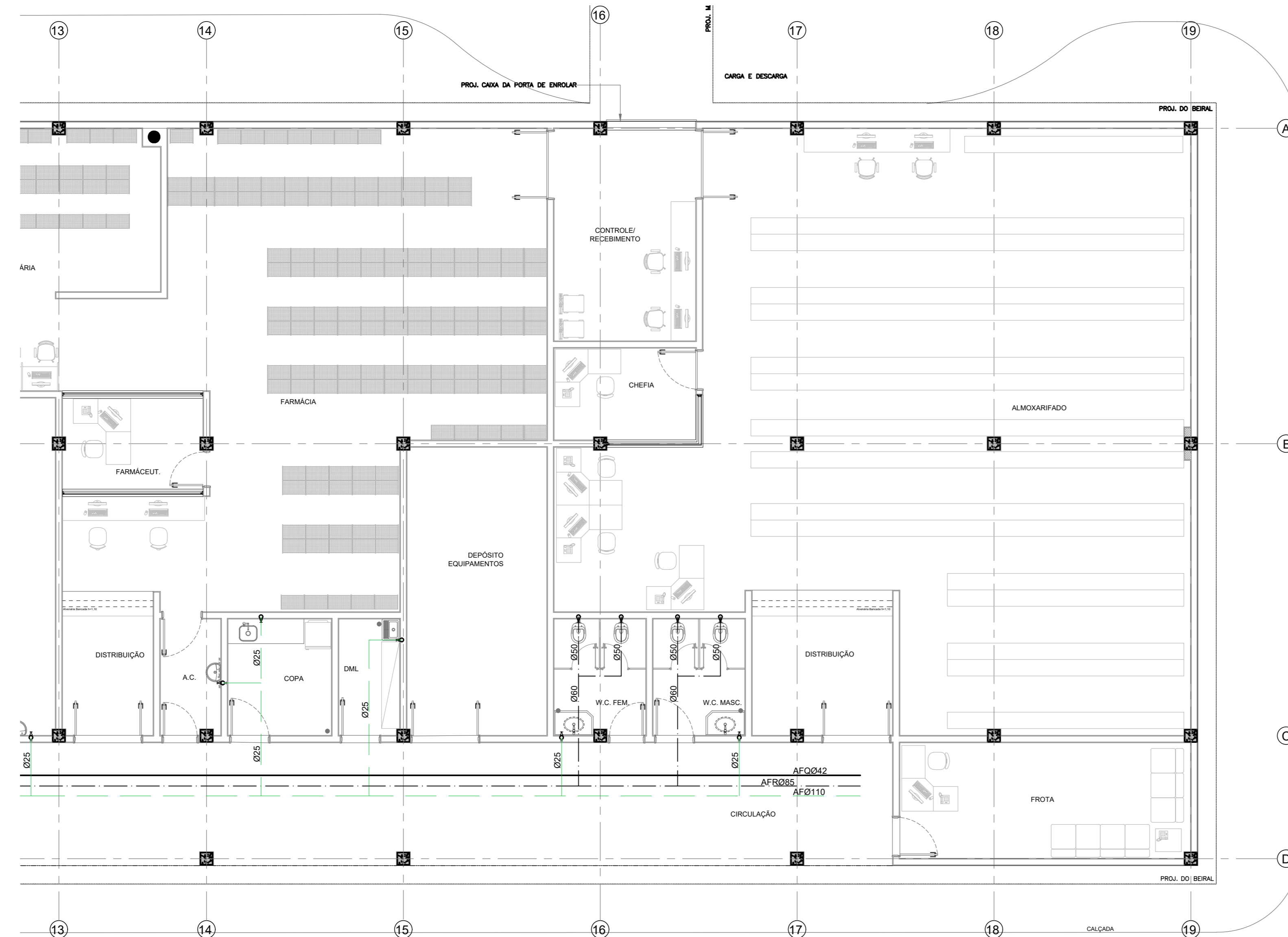
PLANTA PAVIMENTO TÉRREO_BLOCO 2 PARTE 1 - AGUA FRIA / AGUA QUENTE / AGUA REUSO ESC. 1:75
