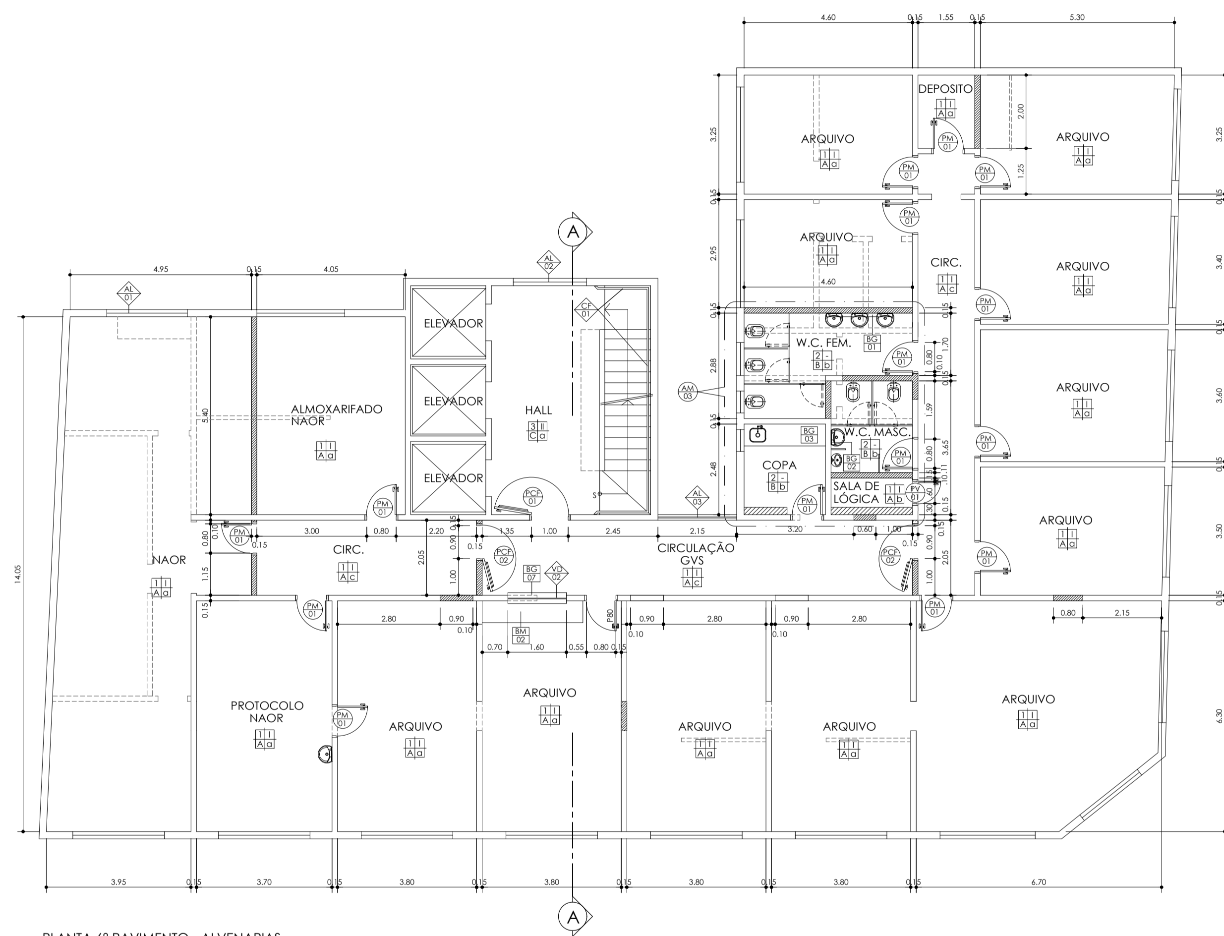
PLANTA 6º PAVIMENTO - ALVENARIAS ESC: 1/25
