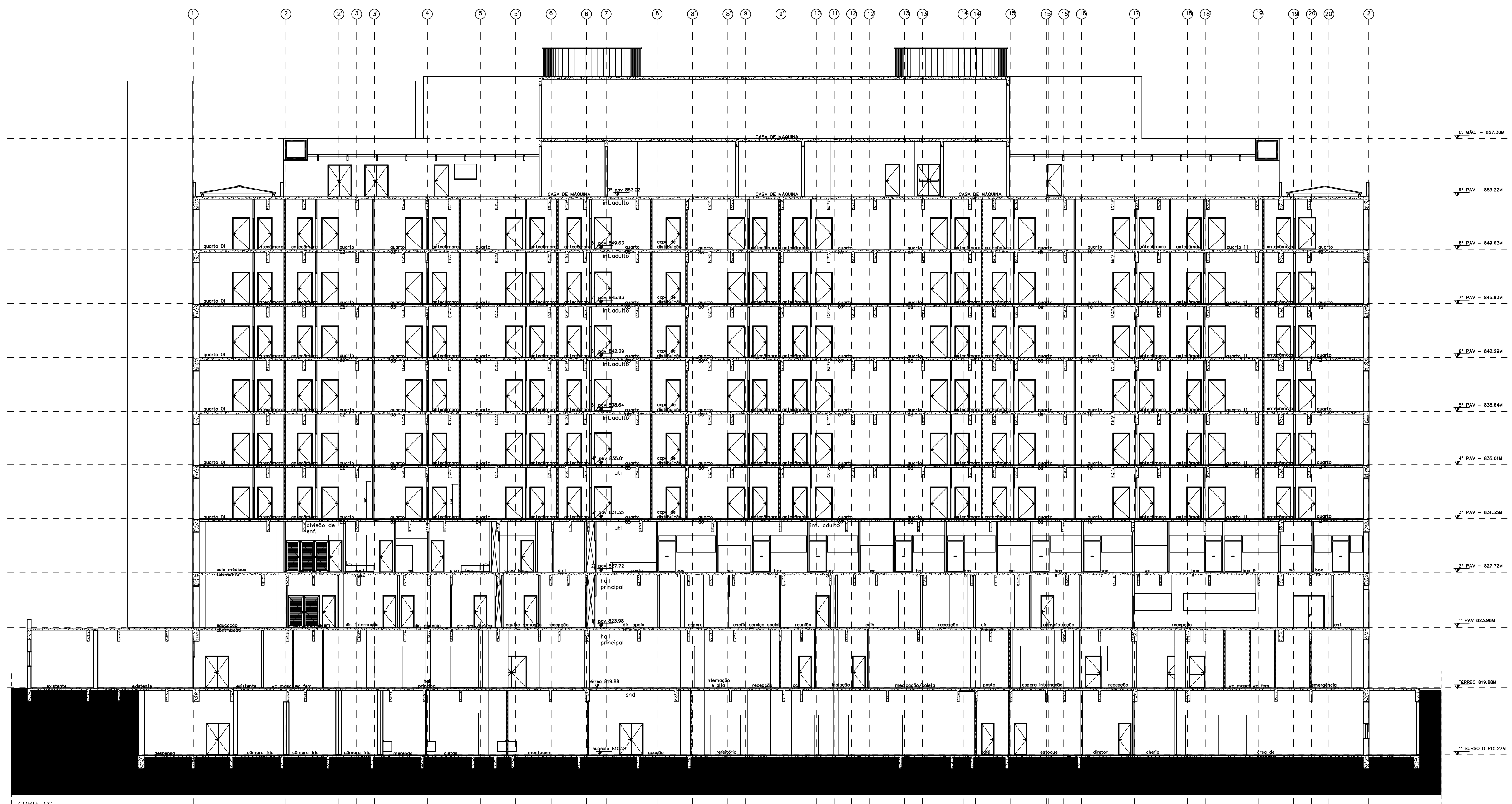
CORTE_CC ESC 1/500
