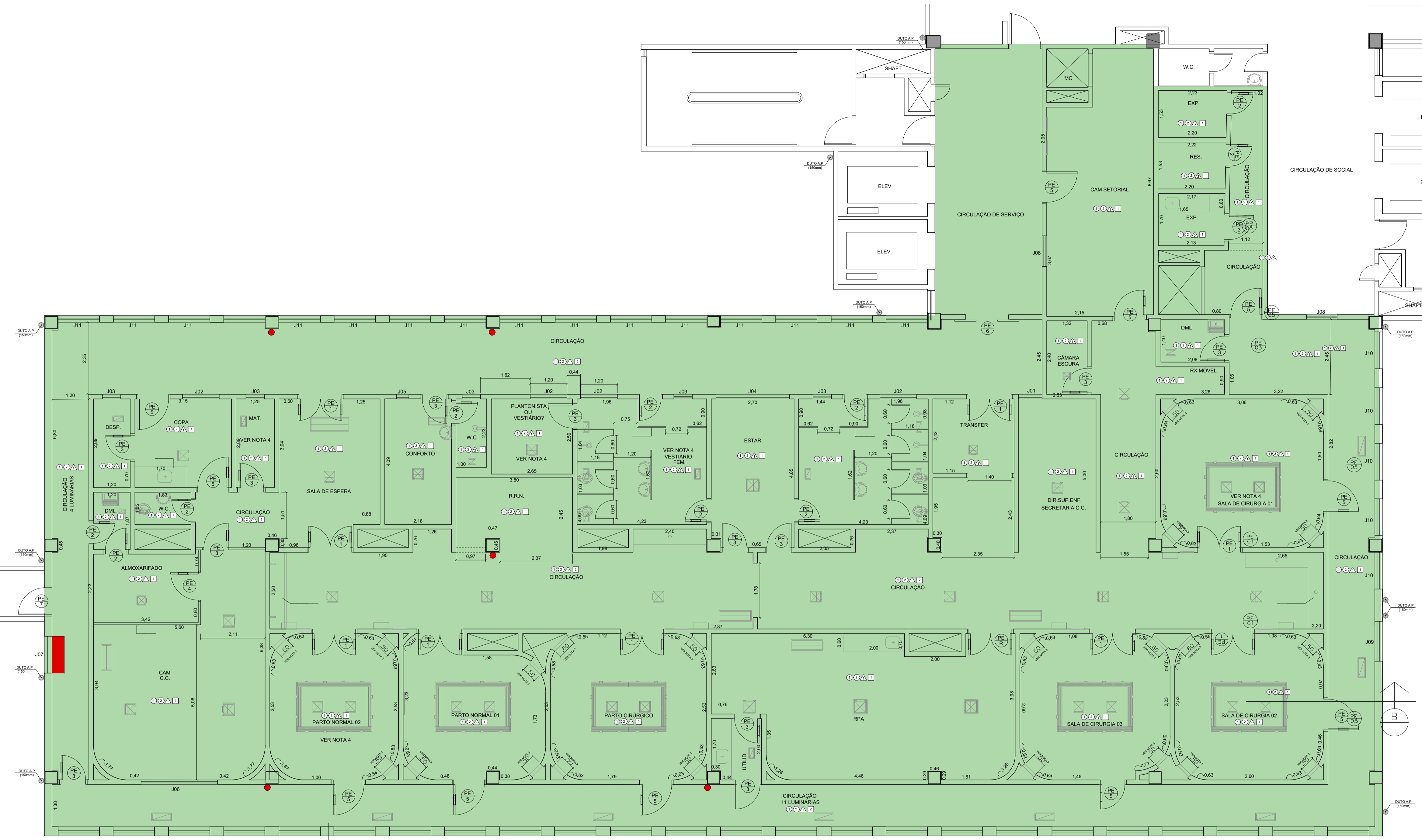
PLANTA LEVANTAMENTO CADASTRAL - CC ESCALA 1/75 PROJETO BÁSICO
