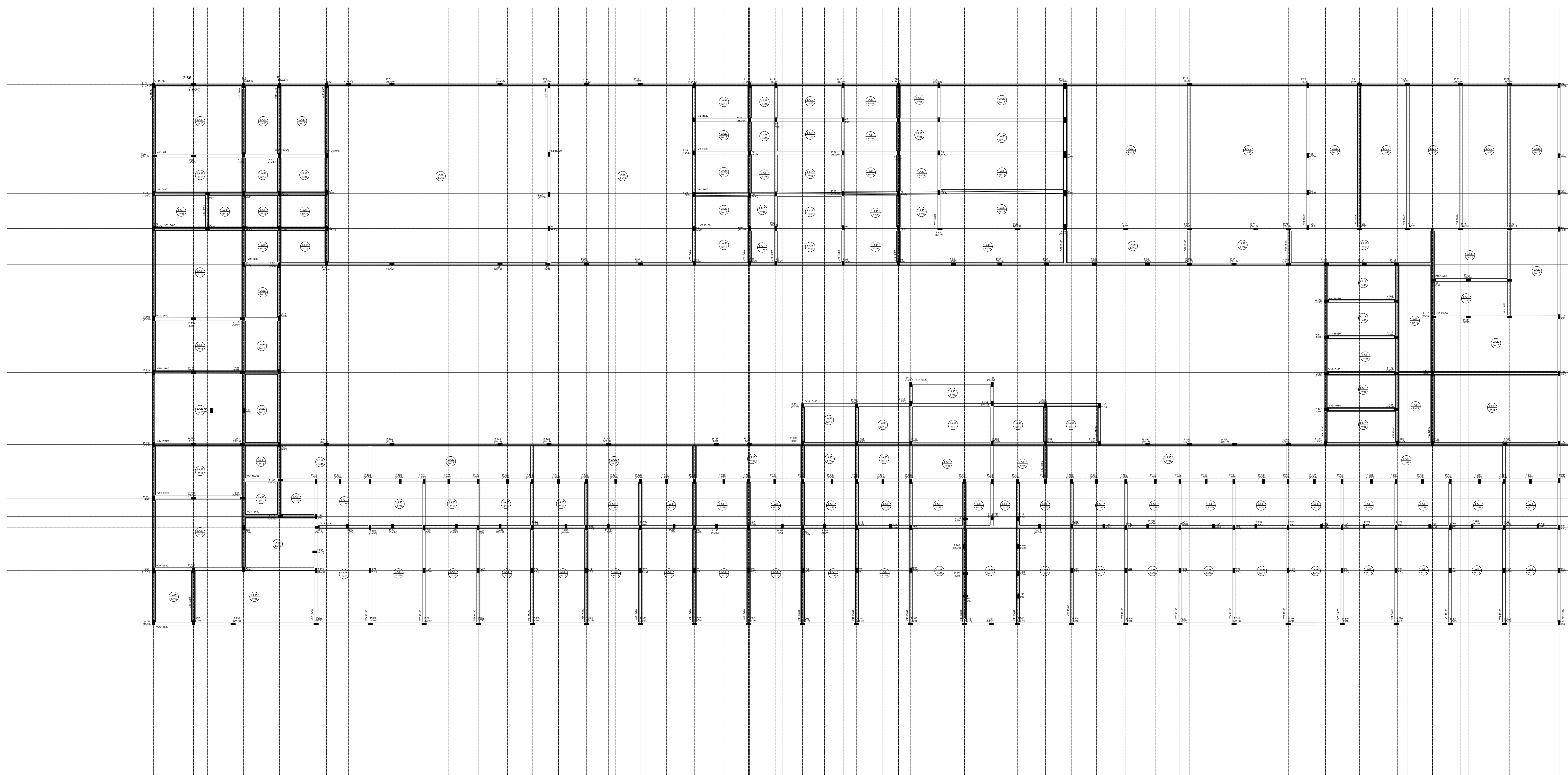
FORMA - LAJES, VIGAS E PILARES 1:100
