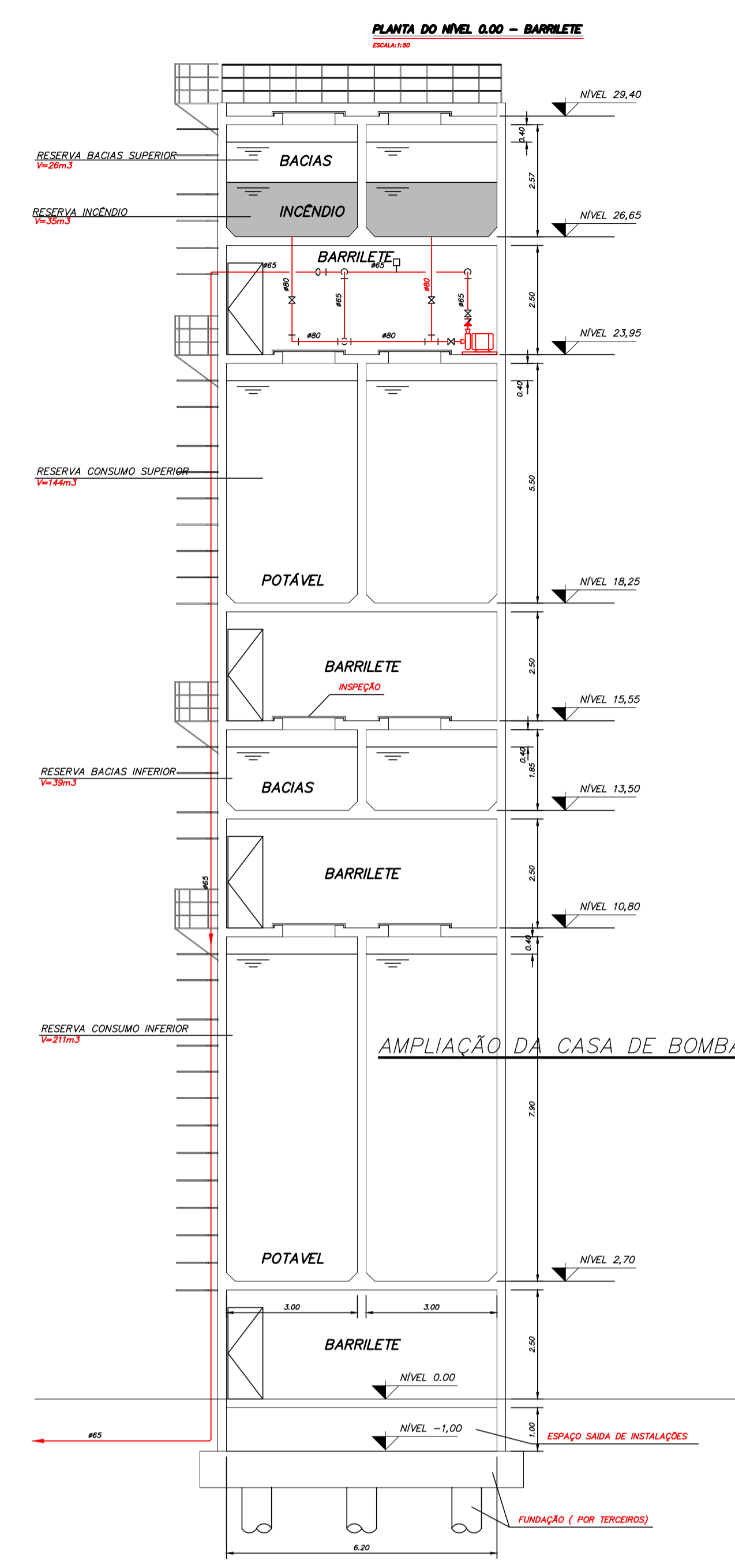
DETALHE DO RESERVATÓRIO ESCALA: 1:75
