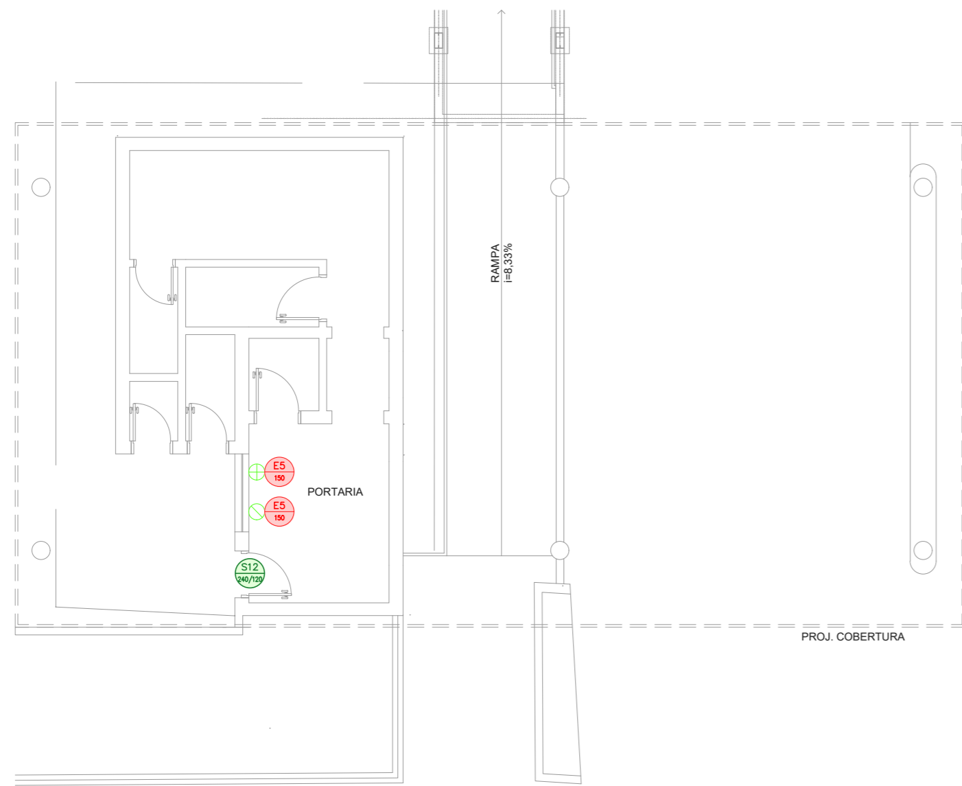
1 CONJUNTO HOSPITALAR MANDAQUI PROJETO BÁSICO DOS SISTEMAS DE INCÊNDIO PLANTA BAIXA - PORTARIA ESCALA 1:100 METRO
