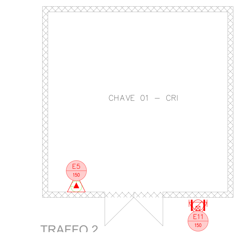
5 CONJUNTO HOSPITALAR MANDAQUI PROJETO BÁSICO DOS SISTEMAS DE INCÊNDIO PLANTA BAIXA - TRAFFO II ESCALA 1:50 METRO
