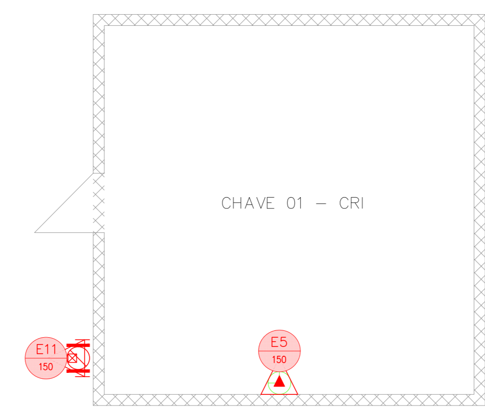
3 CONJUNTO HOSPITALAR MANDAQUI PROJETO BÁSICO DOS SISTEMAS DE INCÊNDIO PLANTA BAIXA - TRAFFO I ESCALA 1:50 METRO
