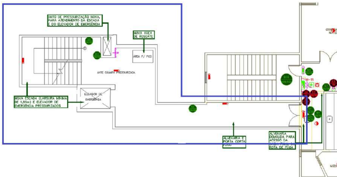
Figura 33 –1º PAVIMENTO– CONJUNTO EMERGÊNCIA 01 – Novo layout
