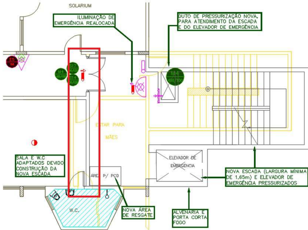
Figura 14 – 3º PAVIMENTO – Demolição (amarelo) /reconstrução paredes
