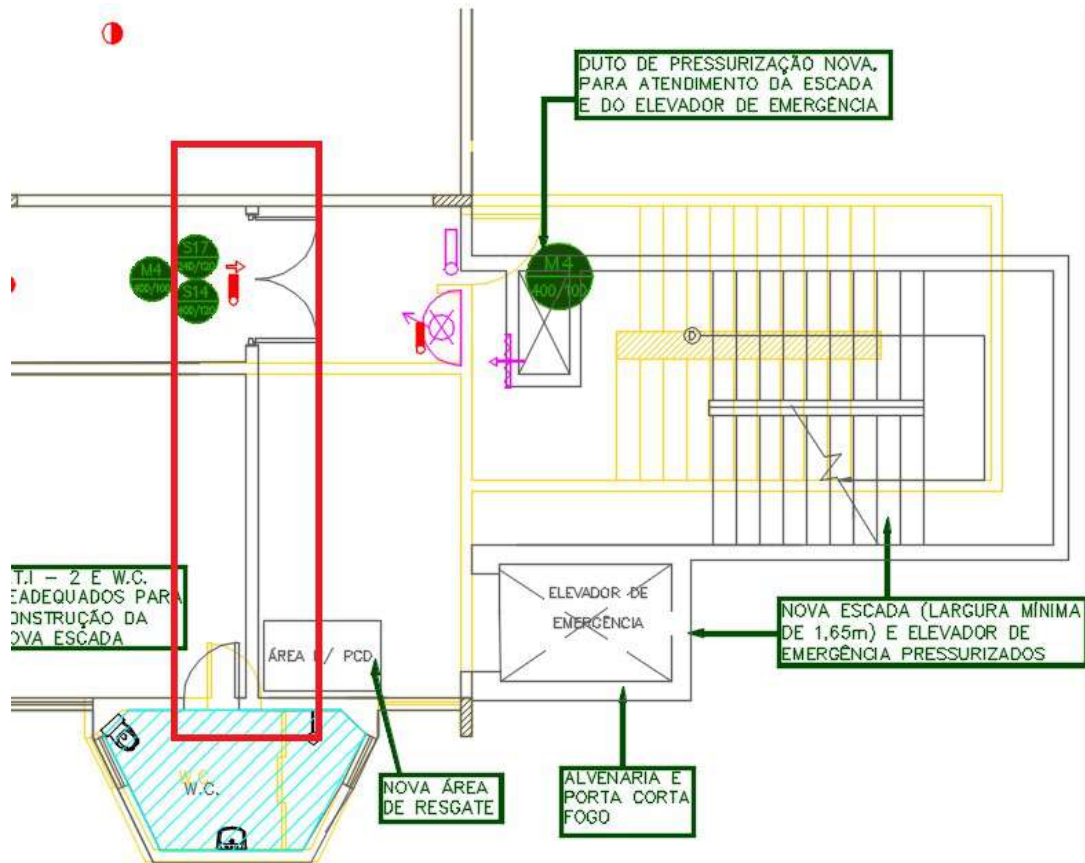
Figura 12 – 2º PAVIMENTO – Demolição (amarelo) /reconstrução paredes
