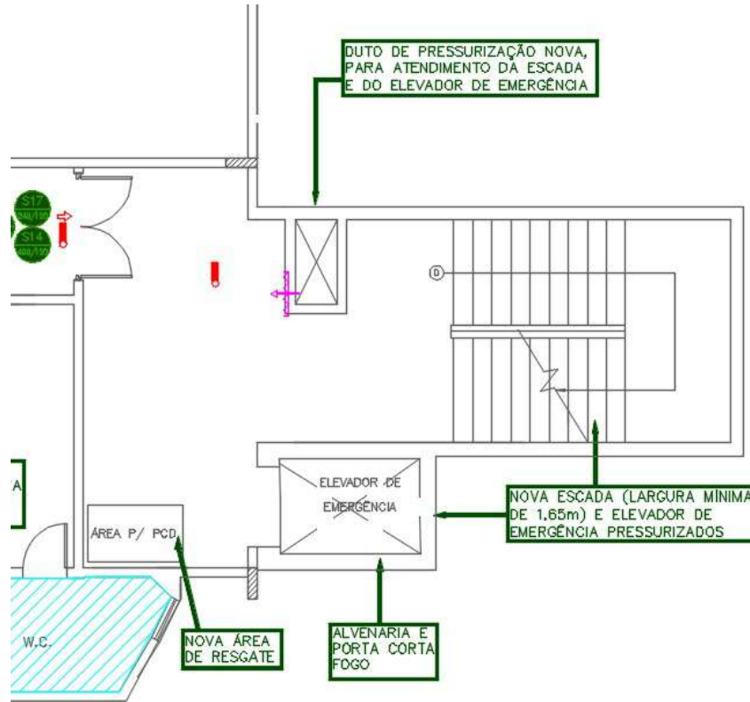
Figura 51 –2º PAVIMENTO– CONJUNTO EMERGÊNCIA 02 – Novo layout
