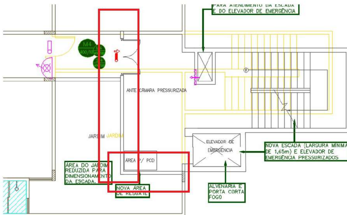
Figura 19 – 4º PAVIMENTO – Demolição (amarelo) /reconstrução paredes
