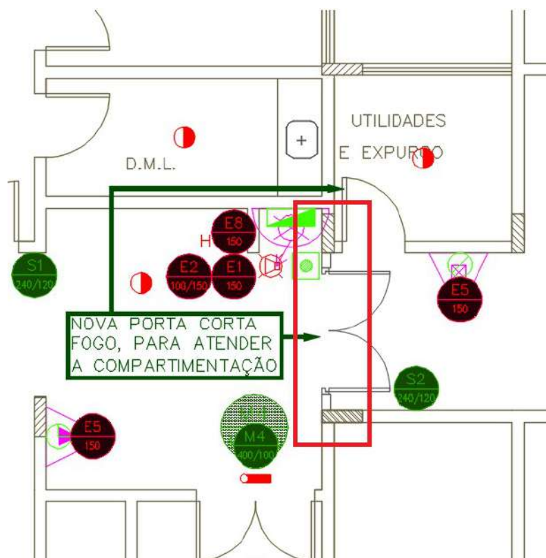
Figura 16 – 4º PAVIMENTO – Construção de parede para compartimentação
