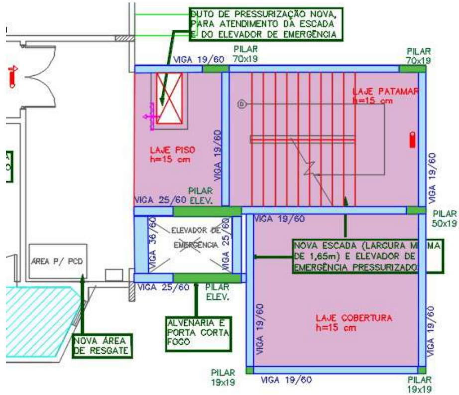
Figura 55 – 1º PAVIMENTO– CONJUNTO EMERGÊNCIA 02 – Croqui estrutura
