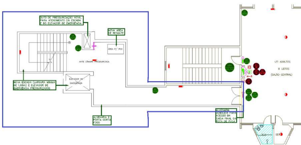
Figura 34 –2º PAVIMENTO– CONJUNTO EMERGÊNCIA 01 – Novo layout
