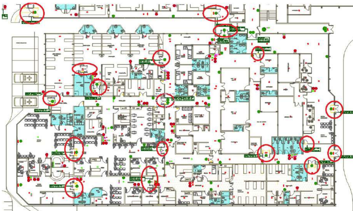
Figura 3 –PAVIMENTO TÉRREO – parte 3/3 - Inversão sentido de porta e remoção/Instalação de nova porta
