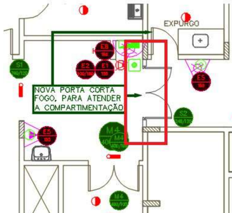
Figura 15 – 3º PAVIMENTO – Construção de parede para compartimentação
