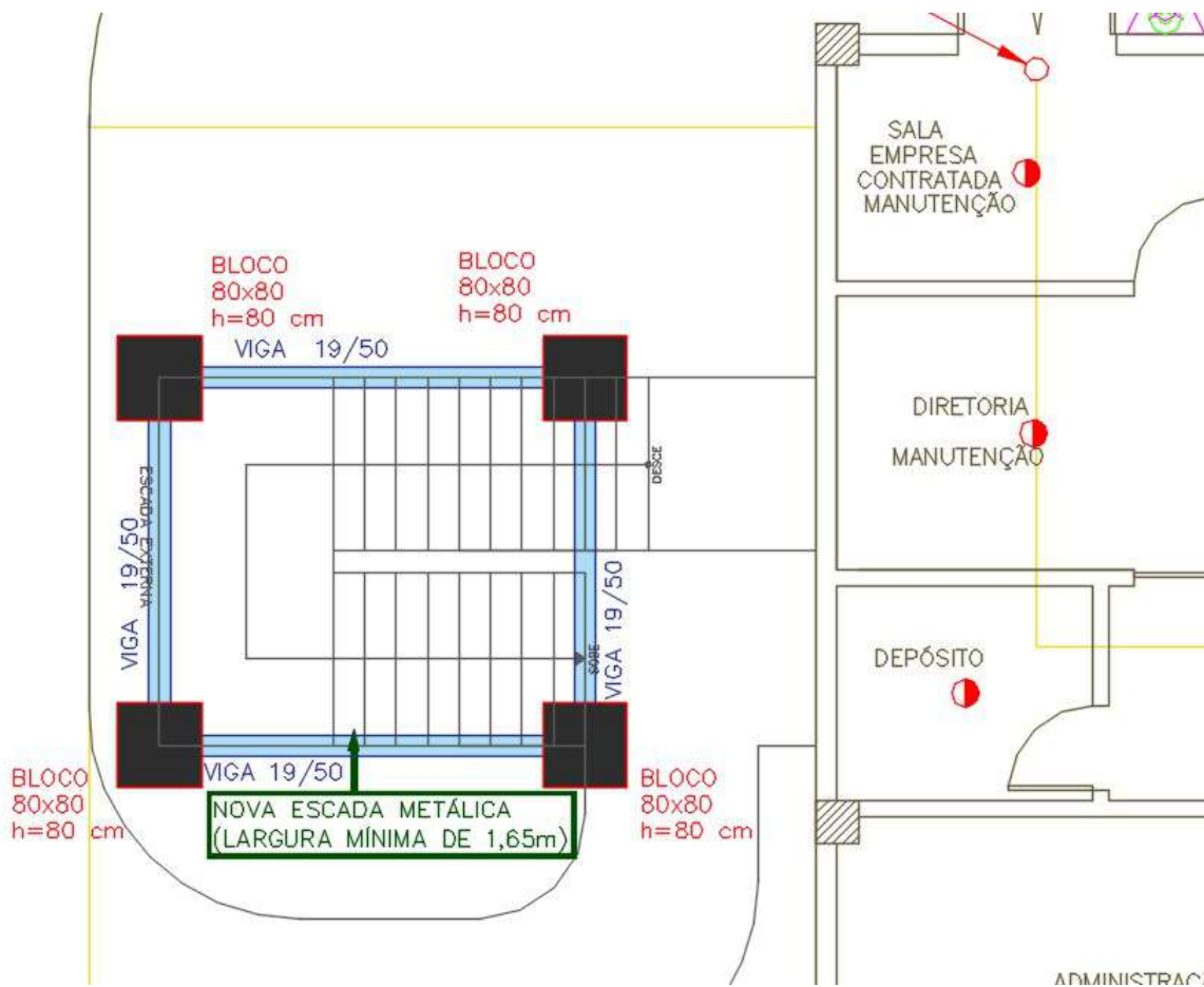
Figura 30 –PAVIMENTO TÉRREO – ESCADA 01 – Croqui estrutura
