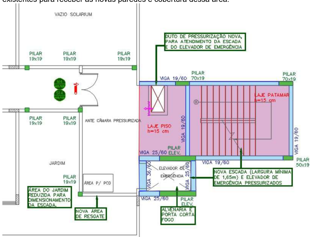
Figura 59 –4º PAVIMENTO– CONJUNTO EMERGÊNCIA 02 – Croqui estrutura
