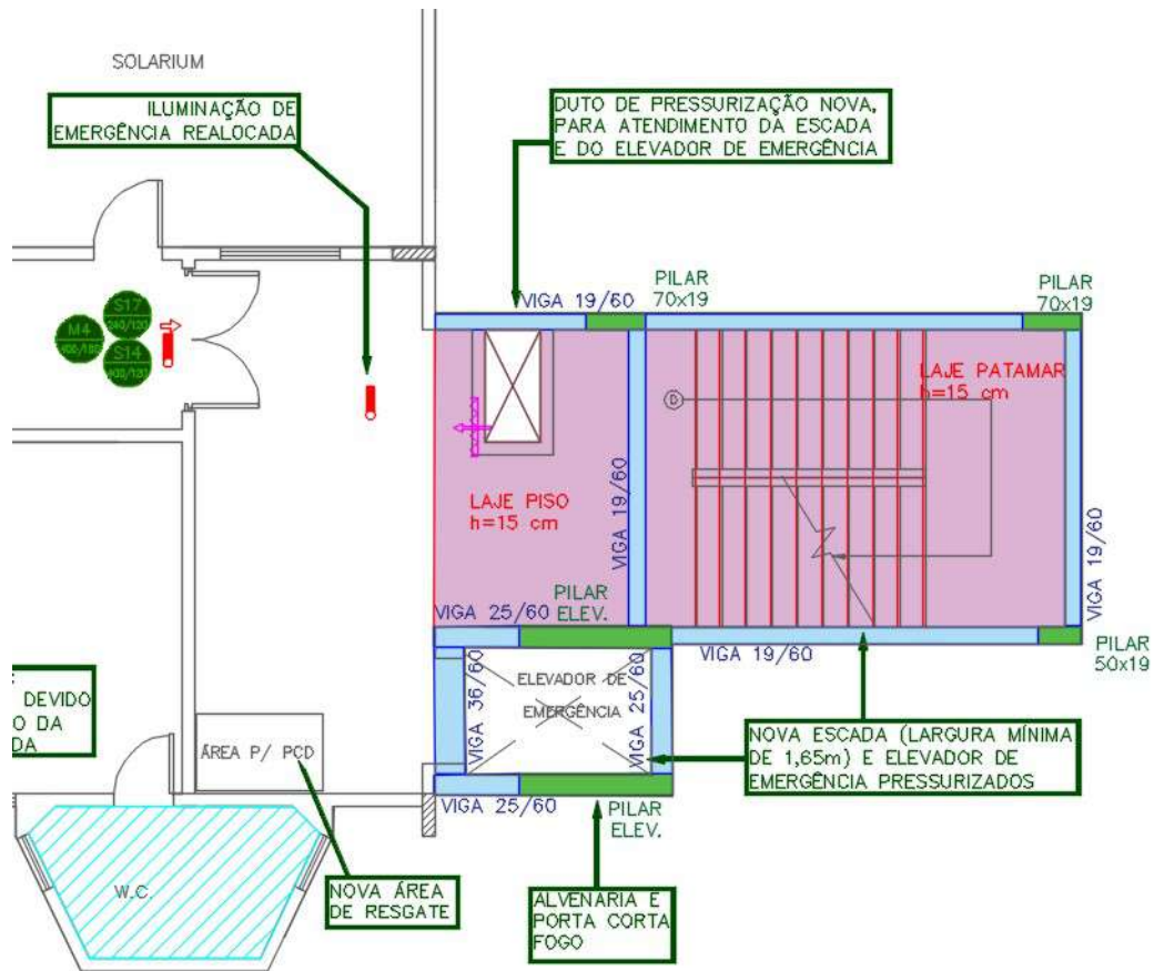
Figura 57 –3º PAVIMENTO– CONJUNTO EMERGÊNCIA 02 – Croqui estrutura
