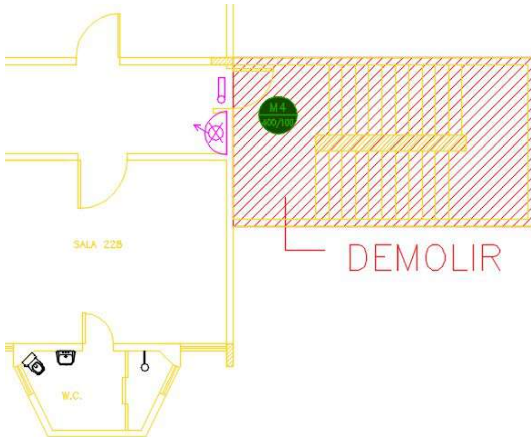
Figura 45 –CONJUNTO EMERGÊNCIA 02 – 1º PAVIMENTO – Levantamento escada existente/demolição
