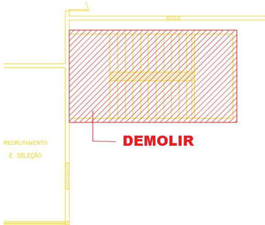
Figura 44 –CONJUNTO EMERGÊNCIA 02 – PAVIMENTO TÉRREO – Levantamento escada existente/demolição
