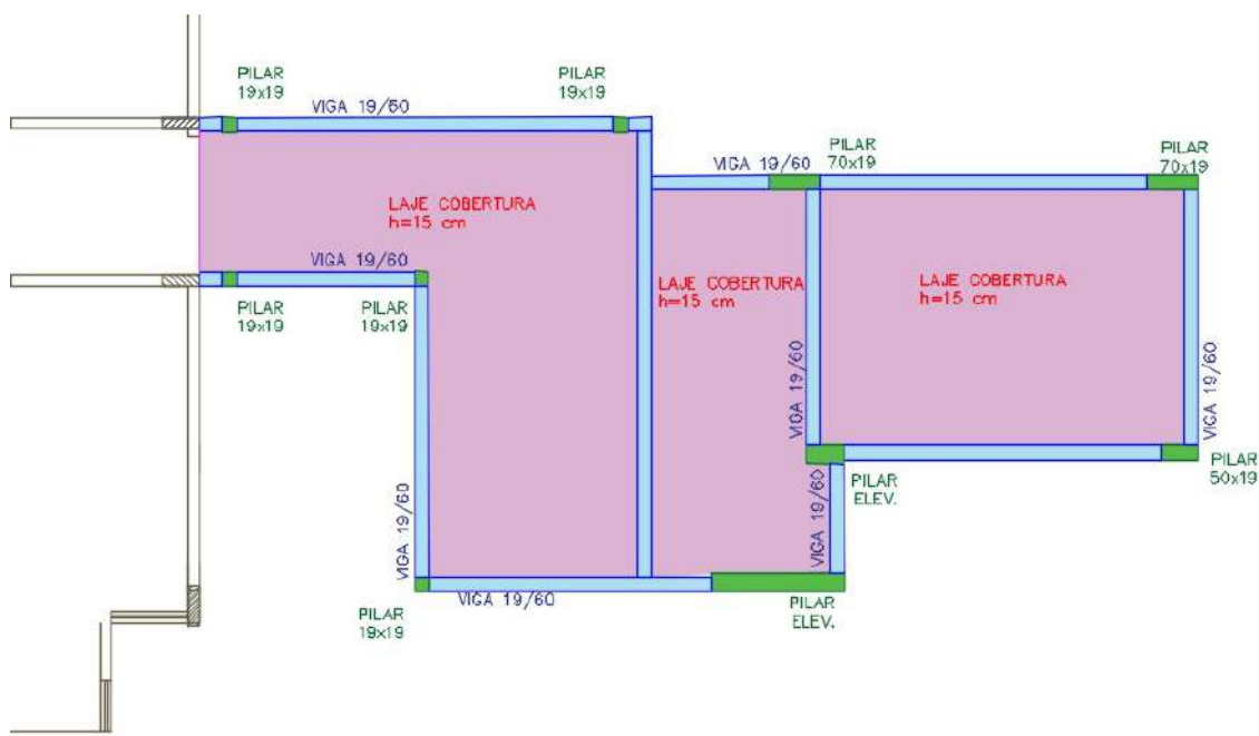
Figura 59 –4º PAVIMENTO– CONJUNTO EMERGÊNCIA 02 – Croqui estrutura
