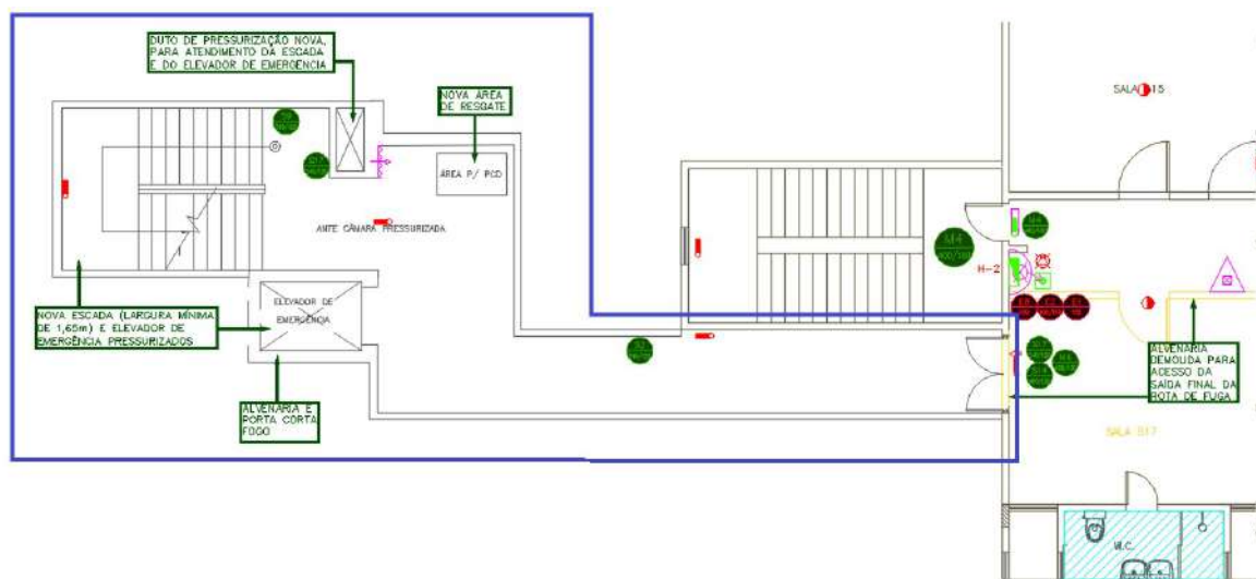
Figura 36 –4º PAVIMENTO– CONJUNTO EMERGÊNCIA 01 – Novo layout
