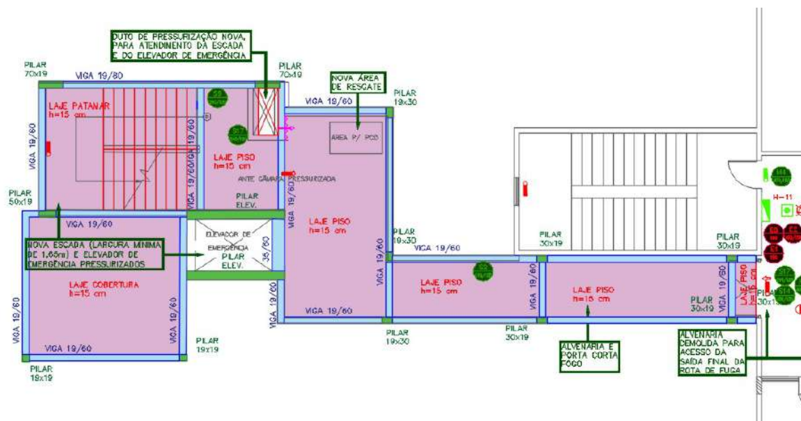
Figura 38 –1º PAVIMENTO– CONJUNTO EMERGÊNCIA 01 – Croqui estrutura
