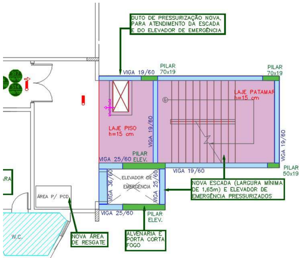
Figura 56 – 2º PAVIMENTO– CONJUNTO EMERGÊNCIA 02 – Croqui estrutura
