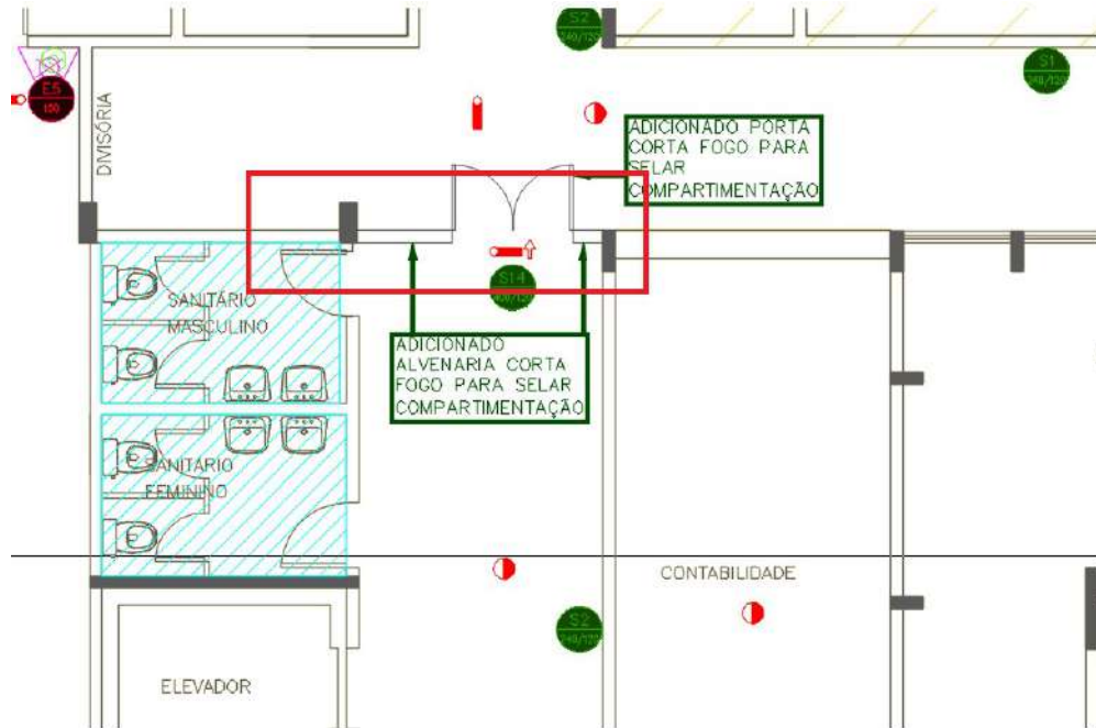
Figura 10 – PAVIMENTO TÉRREO - Construção de parede para compartimentação
