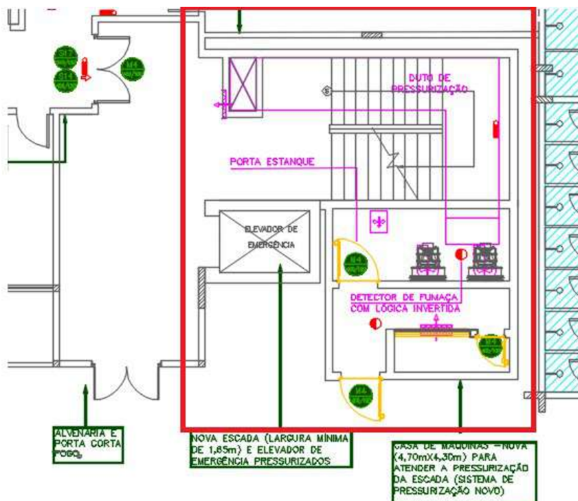
Figura 18 – TÉRREO - Novas alvenarias fechamento conjunto emergência 02 e casa de máquinas
