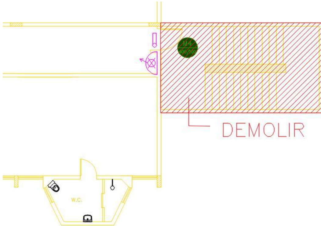
Figura 46 –CONJUNTO EMERGÊNCIA 02 – 2º PAVIMENTO – Levantamento escada existente/demolição
