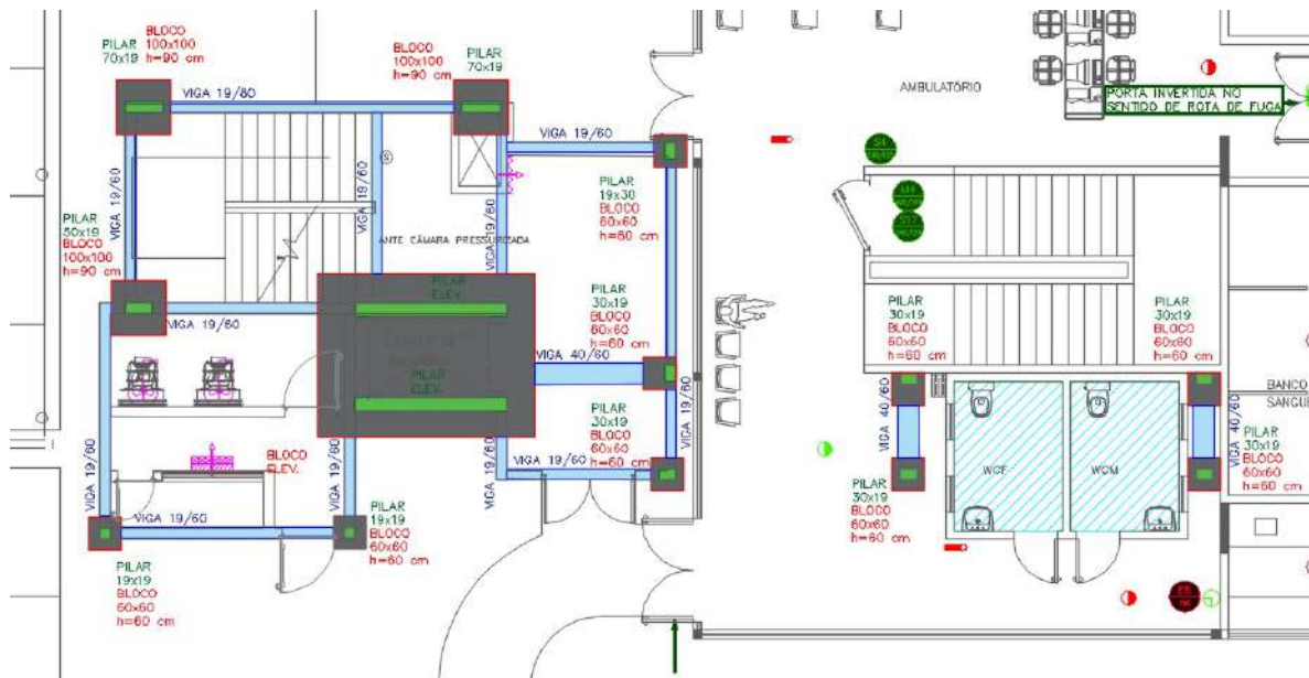
Figura 37 –PAVIMENTO TÉRREO– CONJUNTO EMERGÊNCIA 01 – Croqui estrutura
