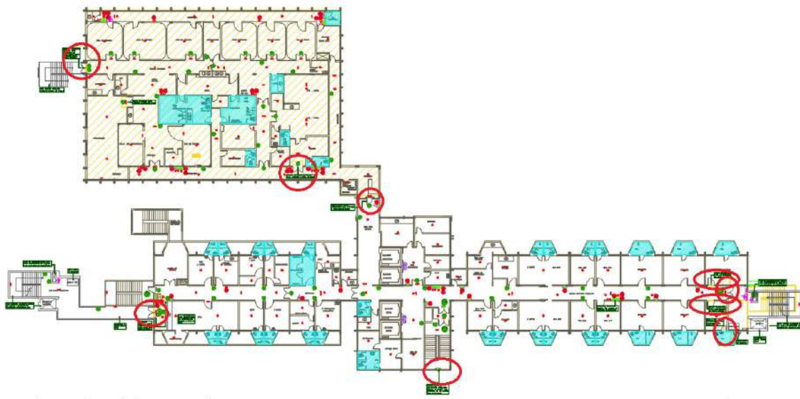
Figura 4 –1º PAVIMENTO - Inversão sentido de porta e remoção/Instalação de nova porta e janela
