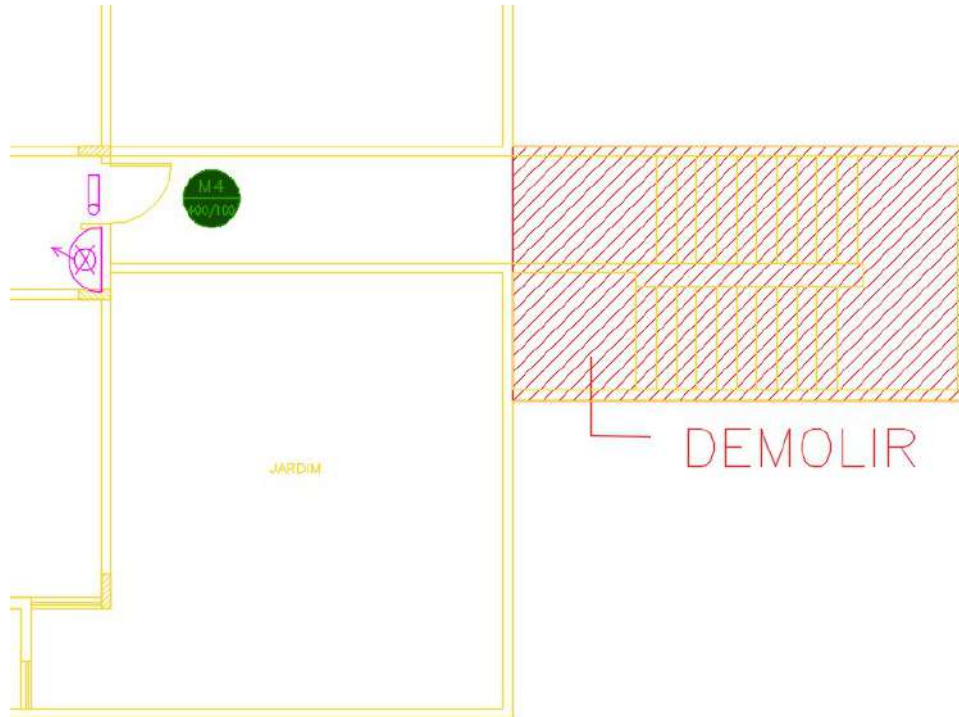
Figura 48 –CONJUNTO EMERGÊNCIA 02 – 4º PAVIMENTO – Levantamento escada existente/demolição
