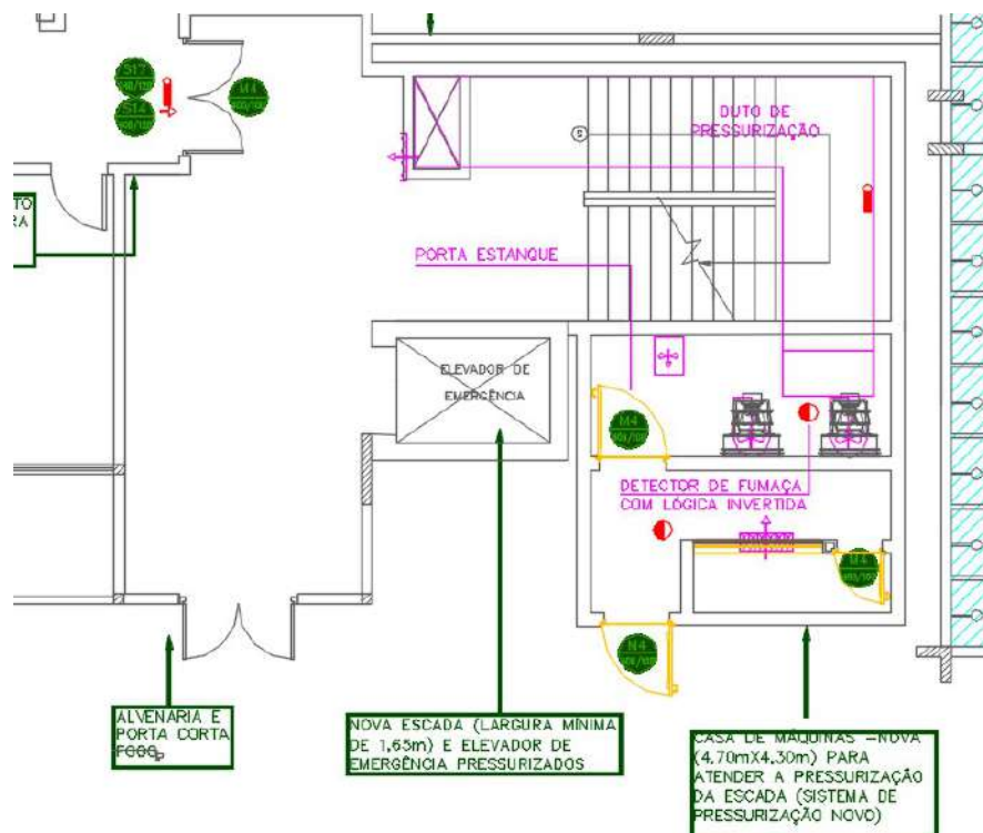
Figura 49 –PAVIMENTO TÉRREO– CONJUNTO EMERGÊNCIA 02 – Novo layout
