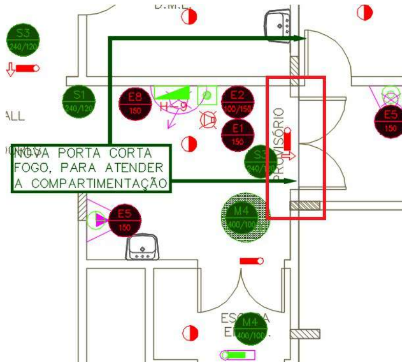
Figura 13 – 2º PAVIMENTO – Construção de parede para compartimentação
