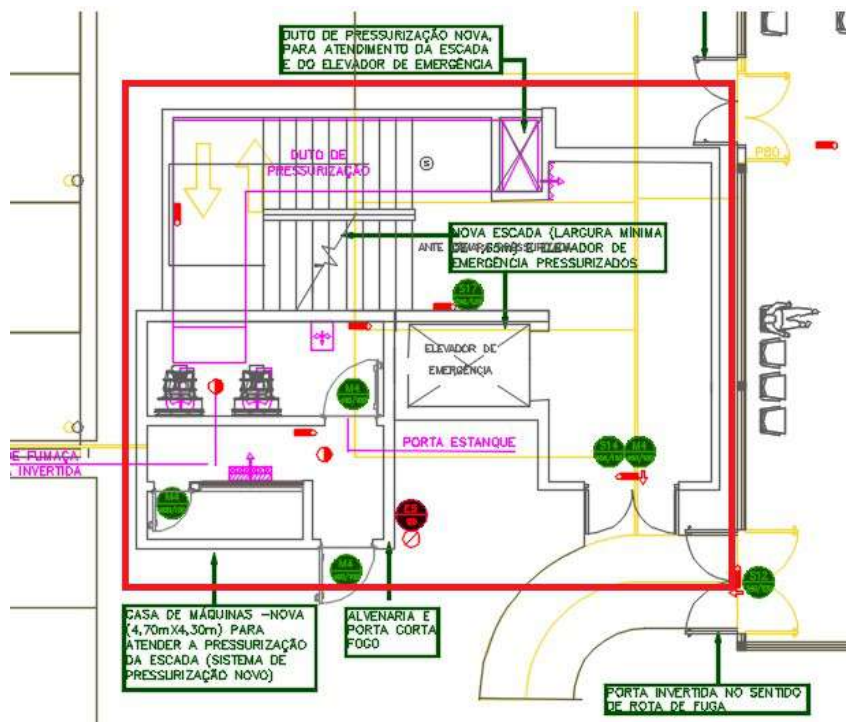
Figura 17 – TÉRREO - Novas alvenarias fechamento conjunto emergência 01 e casa de máquinas
