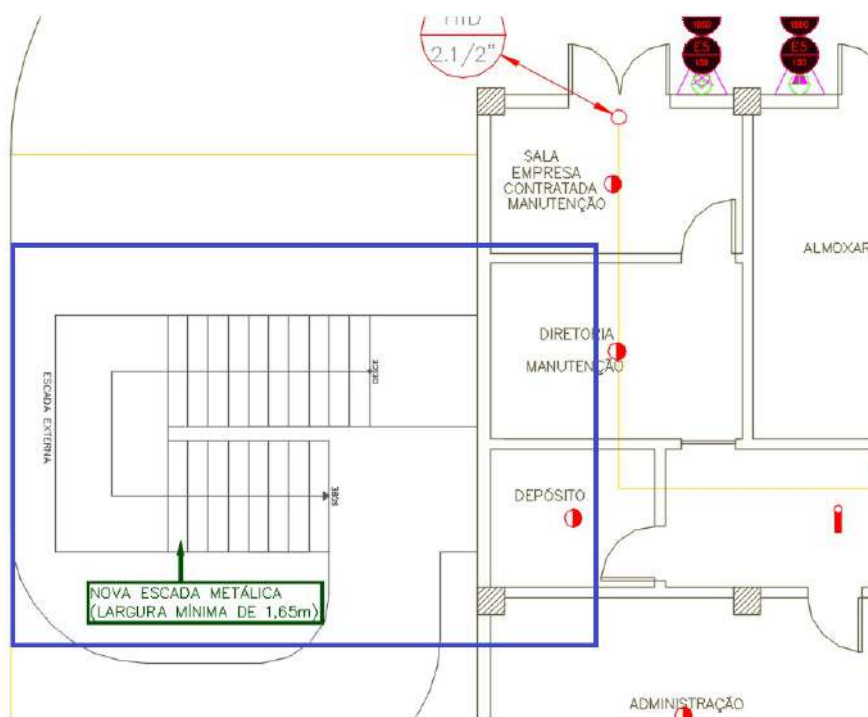
Figura 28 –PAVIMENTO TÉRREO – ESCADA 01 – Layout da saída da nova escada metálica externa
