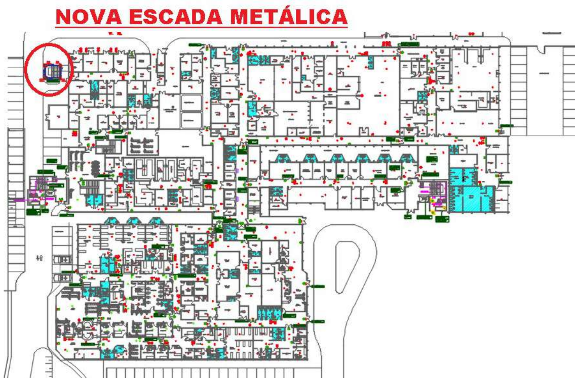
Figura 27 –PAVIMENTO TÉRREO – ESCADA 01 – Locação
