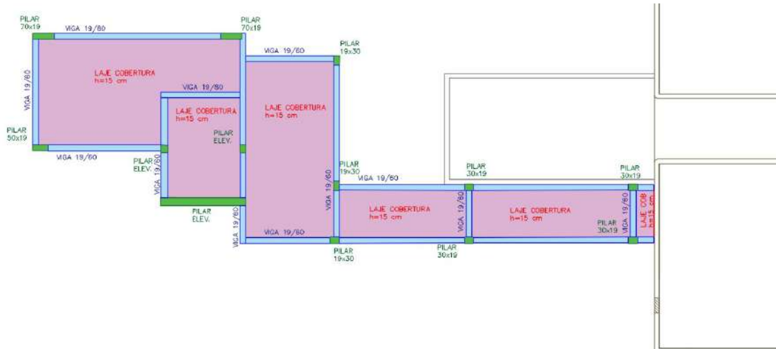
Figura 42 –5º PAVIMENTO– CONJUNTO EMERGÊNCIA 01 – Croqui estrutura
