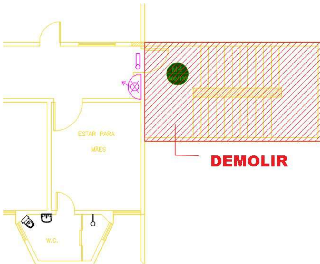
Figura 47 –CONJUNTO EMERGÊNCIA 02 – 3º PAVIMENTO – Levantamento escada existente/demolição
