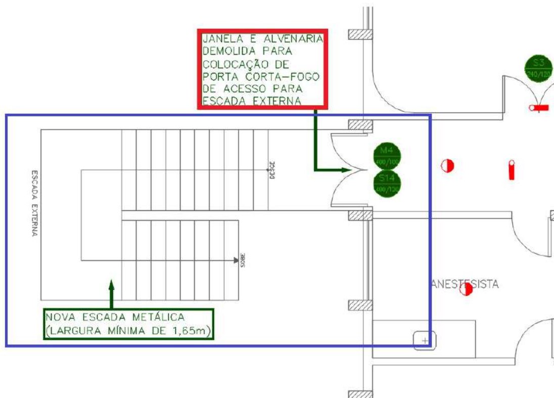
Figura 29 – 1º PAVIMENTO – ESCADA 01 – Layout da chegada da nova escada metálica externa
