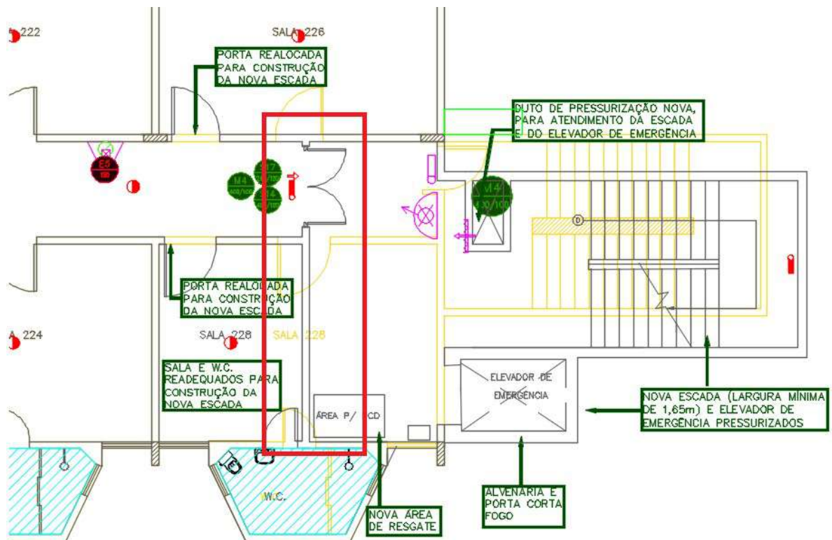
Figura 11 – 1º PAVIMENTO – Demolição (amarelo) /reconstrução paredes
