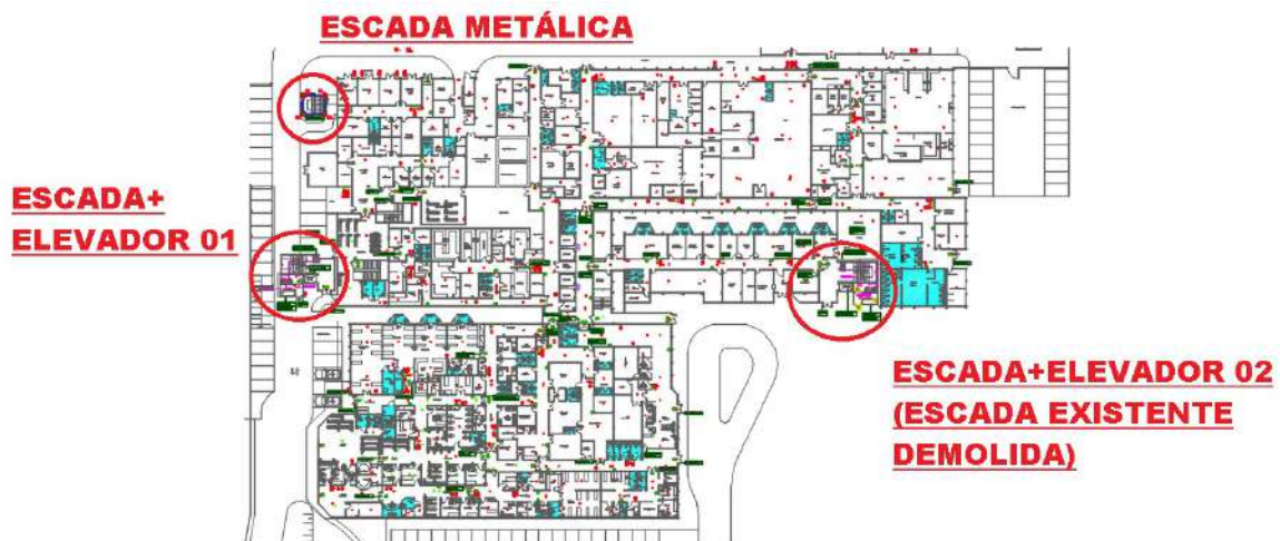
Figura 22 –IMPLANTAÇÃO NOVAS ESCADAS – Layout Térreo
