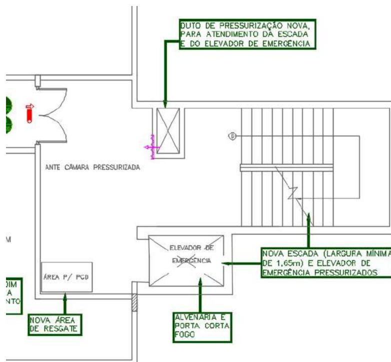
Figura 53 –4º PAVIMENTO– CONJUNTO EMERGÊNCIA 02 – Novo layout
