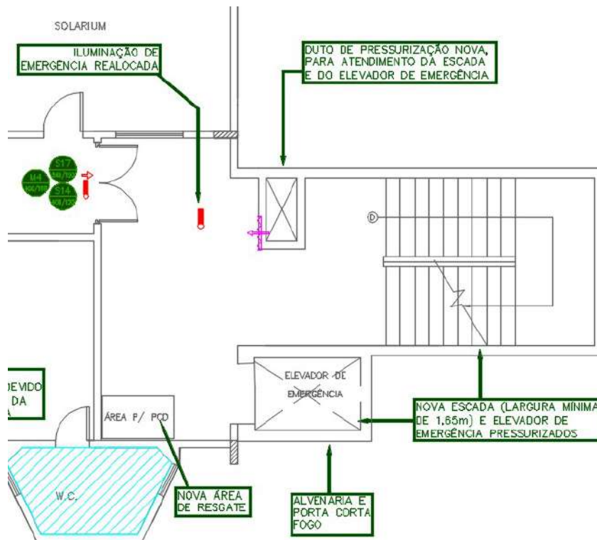
Figura 52 –3º PAVIMENTO– CONJUNTO EMERGÊNCIA 02 – Novo layout
