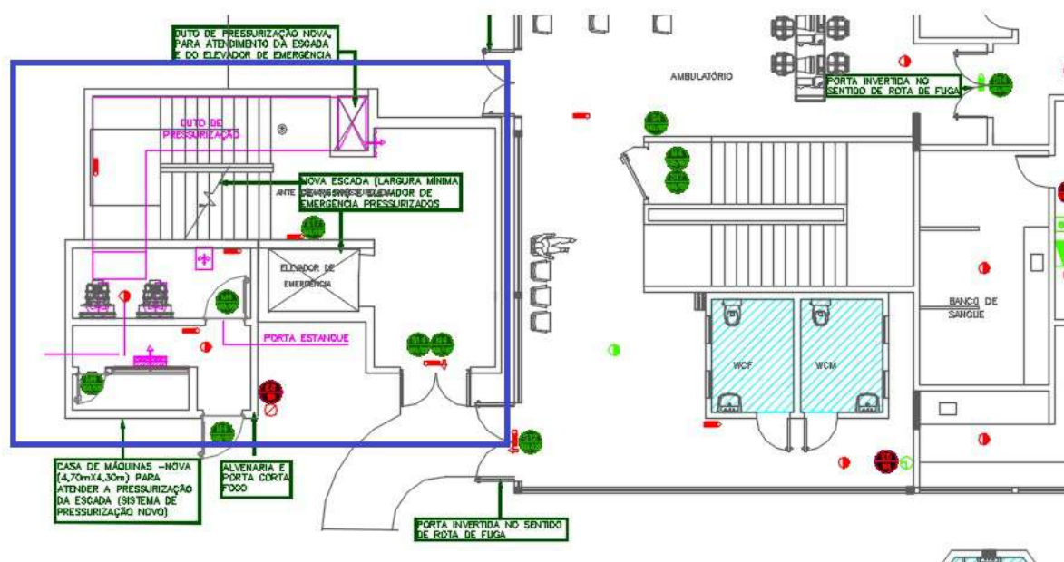
Figura 32 –PAVIMENTO TÉRREO– CONJUNTO EMERGÊNCIA 01 – Novo layout
