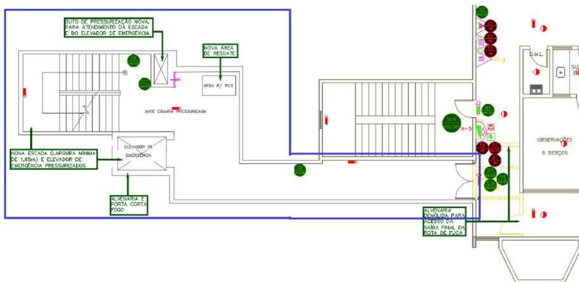
Figura 35 –3º PAVIMENTO– CONJUNTO EMERGÊNCIA 01 – Novo layout
