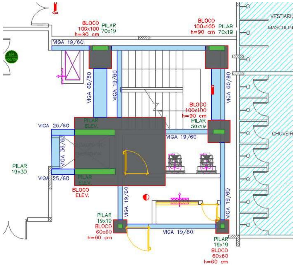
Figura 54 –PAVIMENTO TÉRREO– CONJUNTO EMERGÊNCIA 02 – Croqui estrutura
