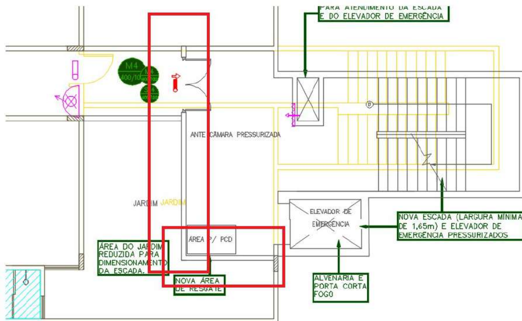
Figura 58 – 4º PAVIMENTO – Novas paredes
