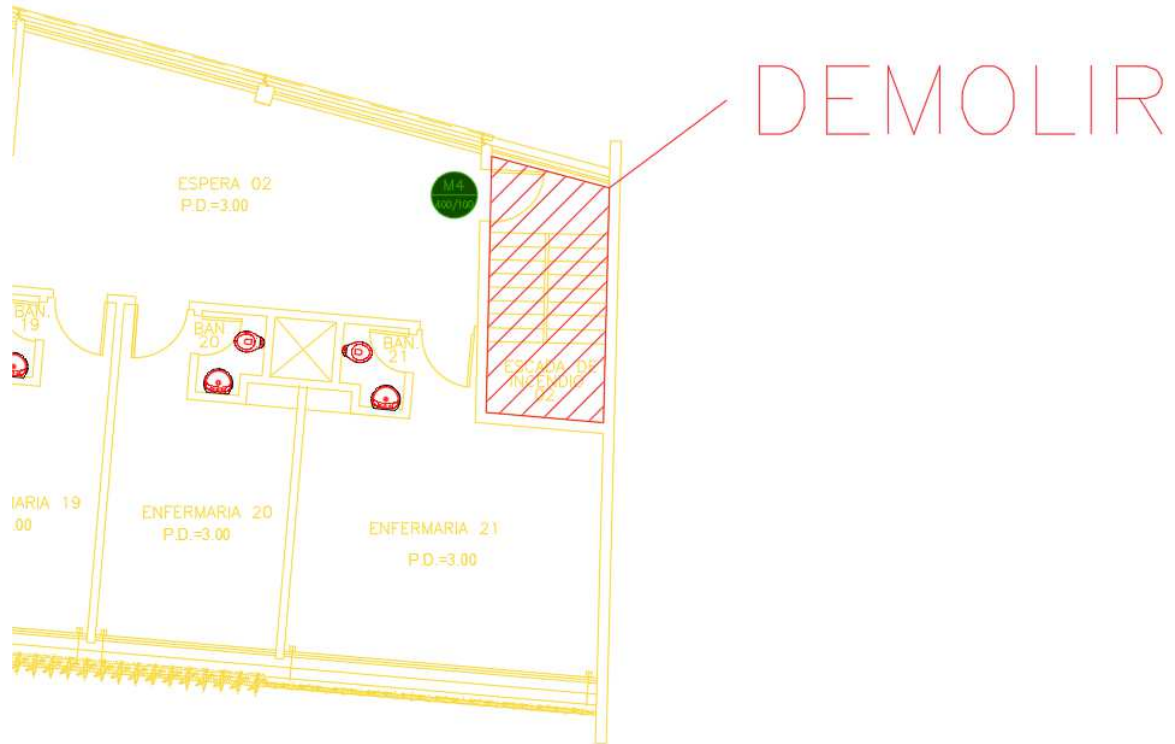
Figura 54 – LEVANTAMENTO ESTRUTURA EXISTENTE - 6º PAVIMENTO – trecho a demolir
