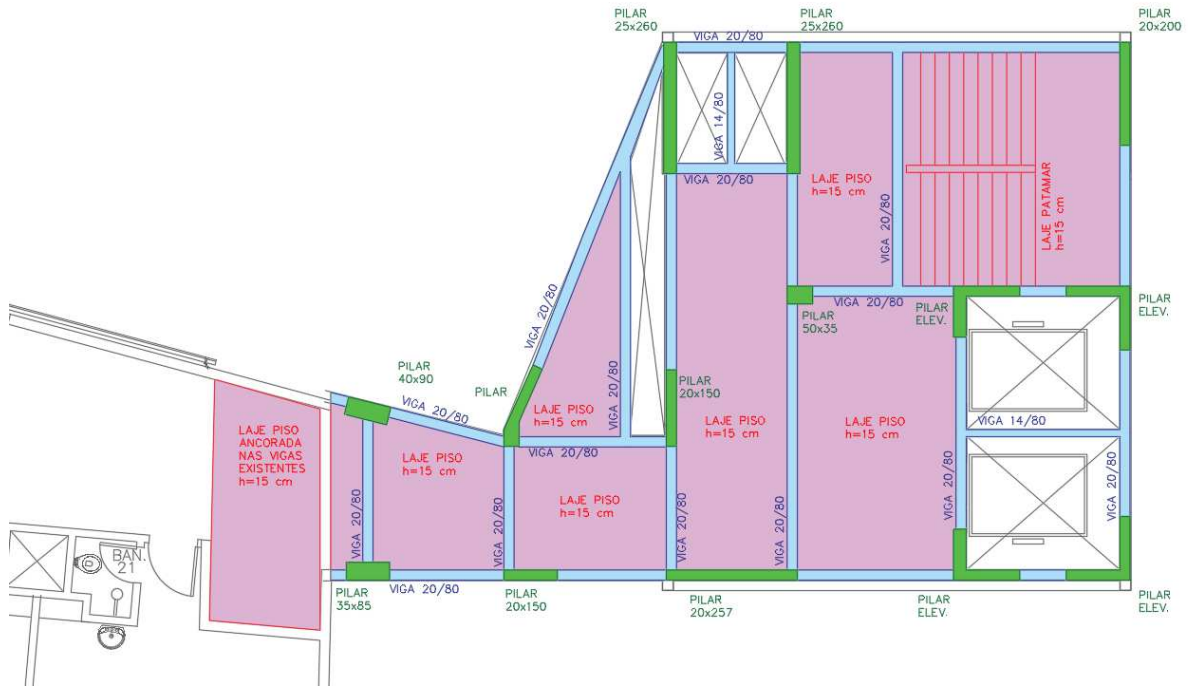
Figura 66 – NOVO CONJUNTO EMERGÊNCIA 01 – 2º AO 9º PAVIMENTO – Croqui Estrutura Tipo
