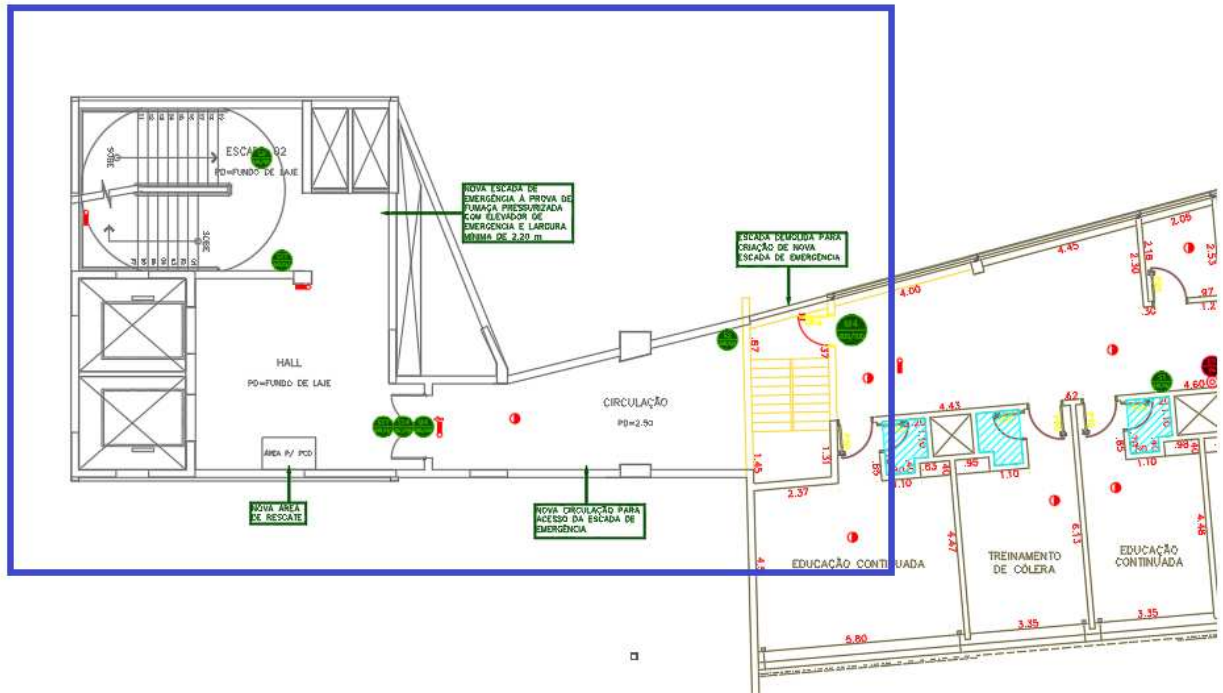
Figura 93 – NOVO CONJUNTO EMERGENCIA 02 – 9º PAVIMENTO - Novo Layout (em amarelo escada existente a ser demolida e fechada)
