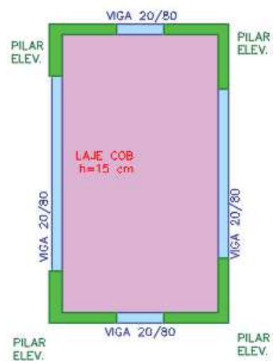
Figura 69 – NOVO CONJUNTO EMERGÊNCIA 01 – COBERTURA C.MÁQ ELEV.– Croqui Estrutura
