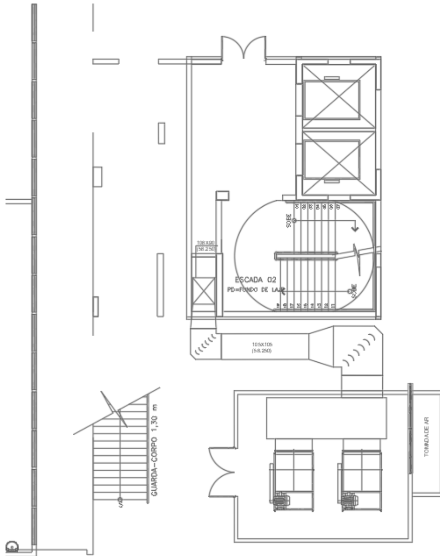
Figura 18 – CONJUNTO 02 – Paredes fechamento escada e casa de máquinas
