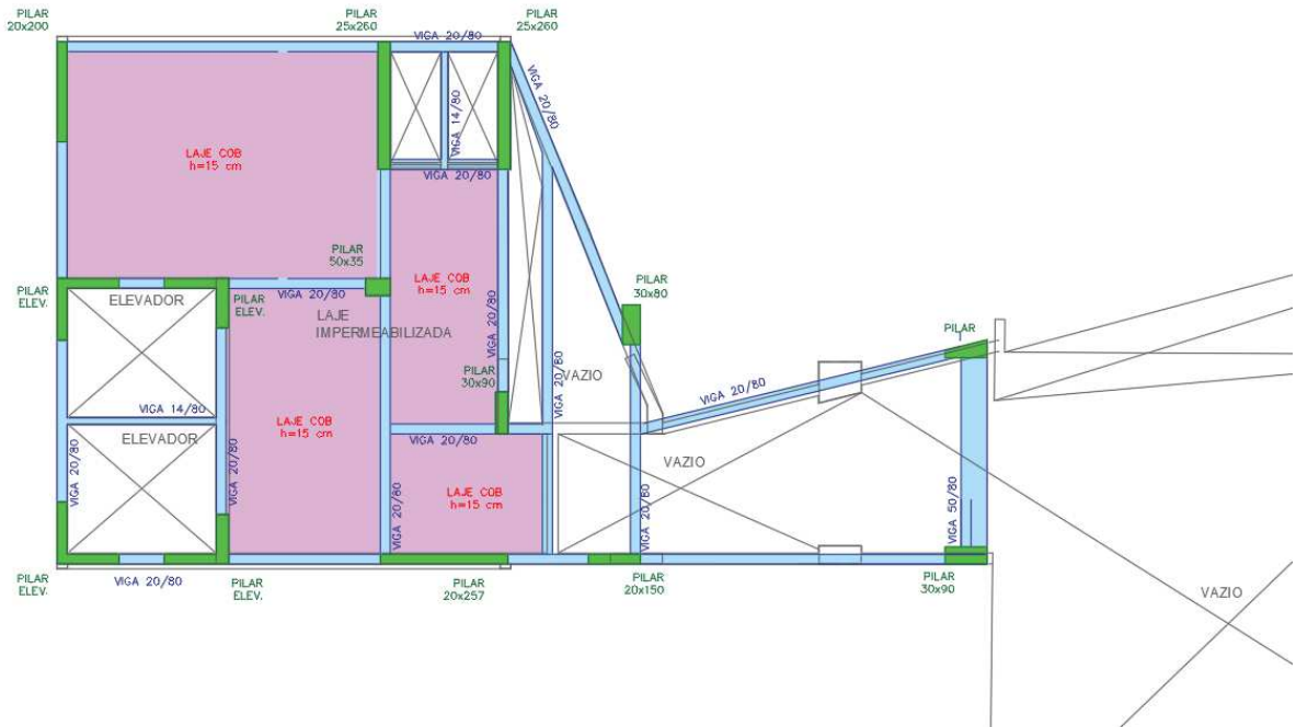
Figura 100 – NOVO CONJUNTO EMERGÊNCIA 02 – COBERTURA – Croqui Estrutura
