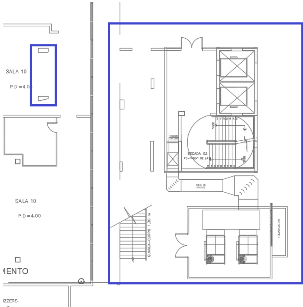
Figura 72 – NOVO CONJUNTO EMERGÊNCIA 02 – TÉRREO - Layout da saída da escada + casa de máquinas
