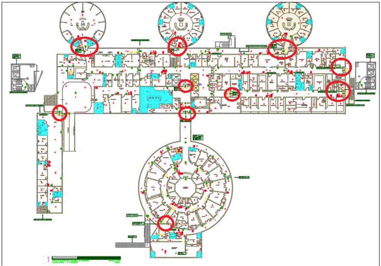
Figura 3 – 1º PAVIMENTO – Inversão no sentido de portas/Remoção e instalação de novas portas
