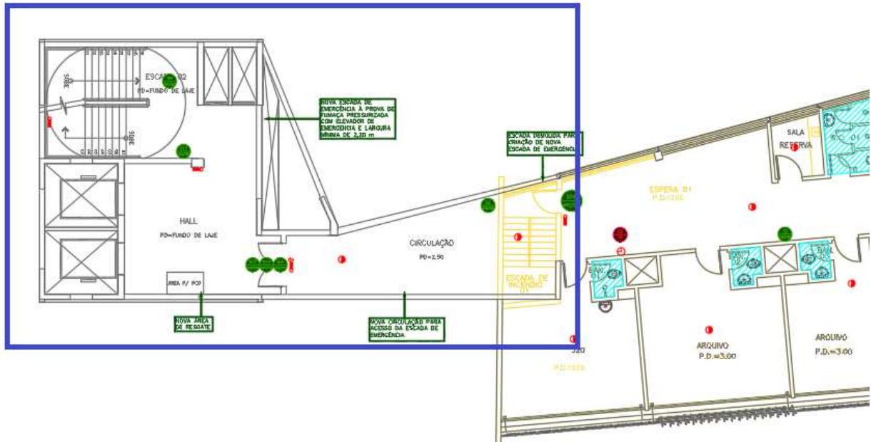
Figura 81 – NOVO CONJUNTO EMERGENÇA 02 – 3º PAVIMENTO - Novo Layout (em amarelo escada existente a ser demolida e fechada)
