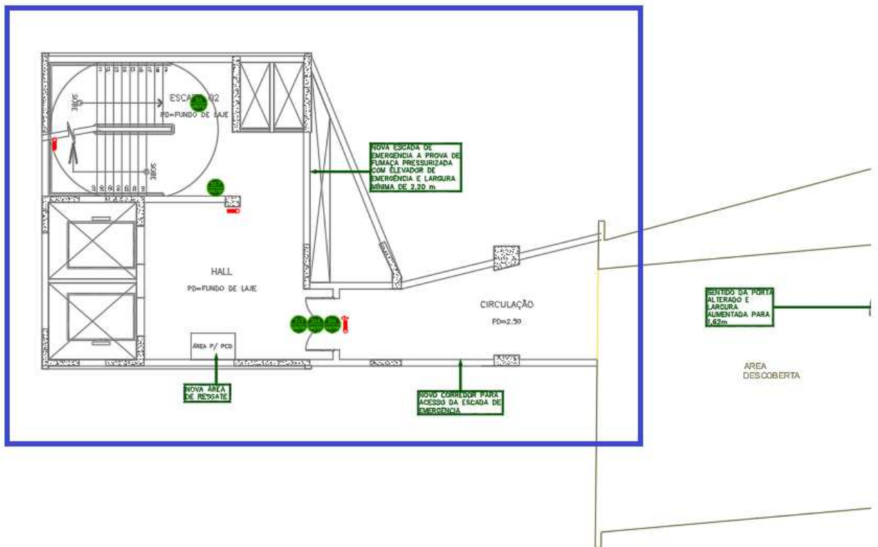
Figura 94 – NOVO CONJUNTO EMERGENCIA 02 – 10º PAVIMENTO - Novo Layout
