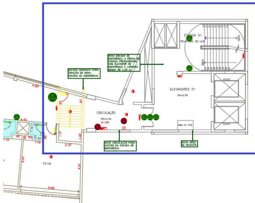
Figura 57 – NOVO CONJUNTO EMERGÊNCIA 01 – 7º PAVIMENTO - Novo Layout (em amarelo escada existente a ser demolida e fechada)
