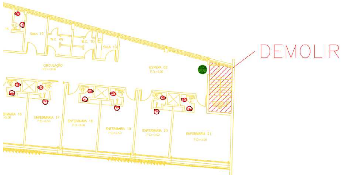
Figura 58 – LEVANTAMENTO ESTRUTURA EXISTENTE - 8º PAVIMENTO – trecho a demolir
