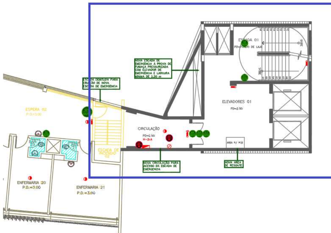
Figura 51 – NOVO CONJUNTO EMERGÊNCIA 01 – 4º PAVIMENTO - Novo Layout (em amarelo escada existente a ser demolida e fechada)
