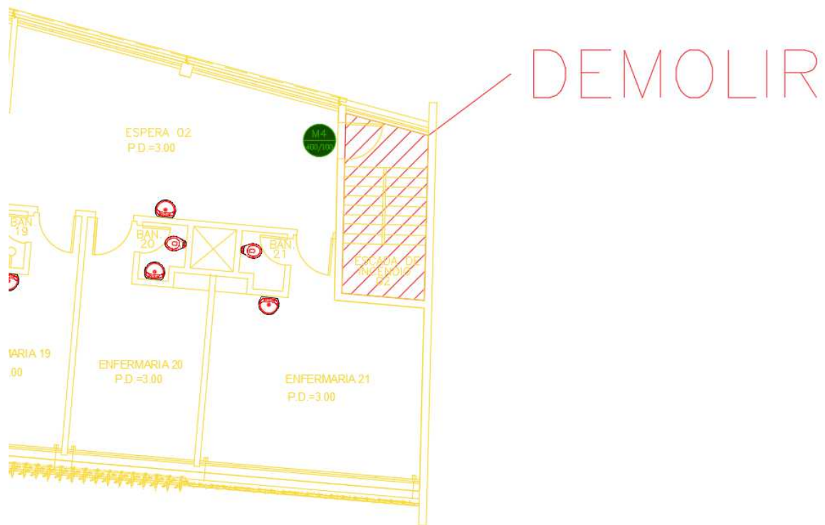
Figura 50 – LEVANTAMENTO ESTRUTURA EXISTENTE - 4º PAVIMENTO – trecho a demolir
