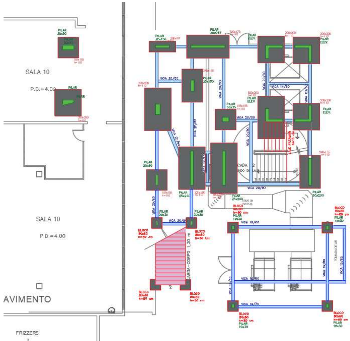
Figura 96 – NOVO CONJUNTO EMERGÊNCIA 02 – TÉRREO – Croqui Estrutura
