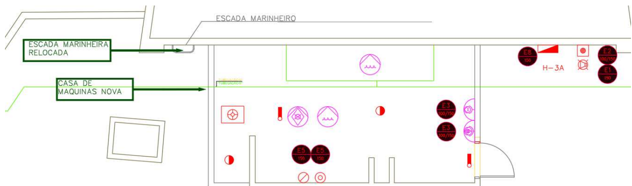
Figura 19 – NOVA CASA MÁQUINAS COBERTURA – Paredes fechamento
