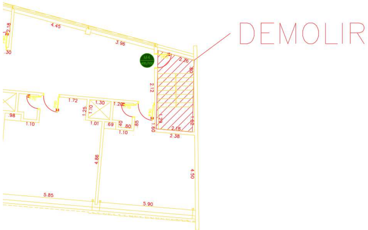
Figura 60 – LEVANTAMENTO ESTRUTURA EXISTENTE - 9º PAVIMENTO – trecho a demolir
