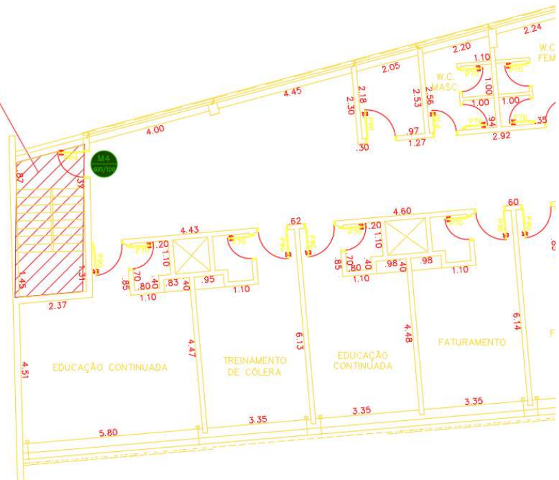
Figura 92 – LEVANTAMENTO ESTRUTURA EXISTENTE - 9º PAVIMENTO – trecho a demolir
