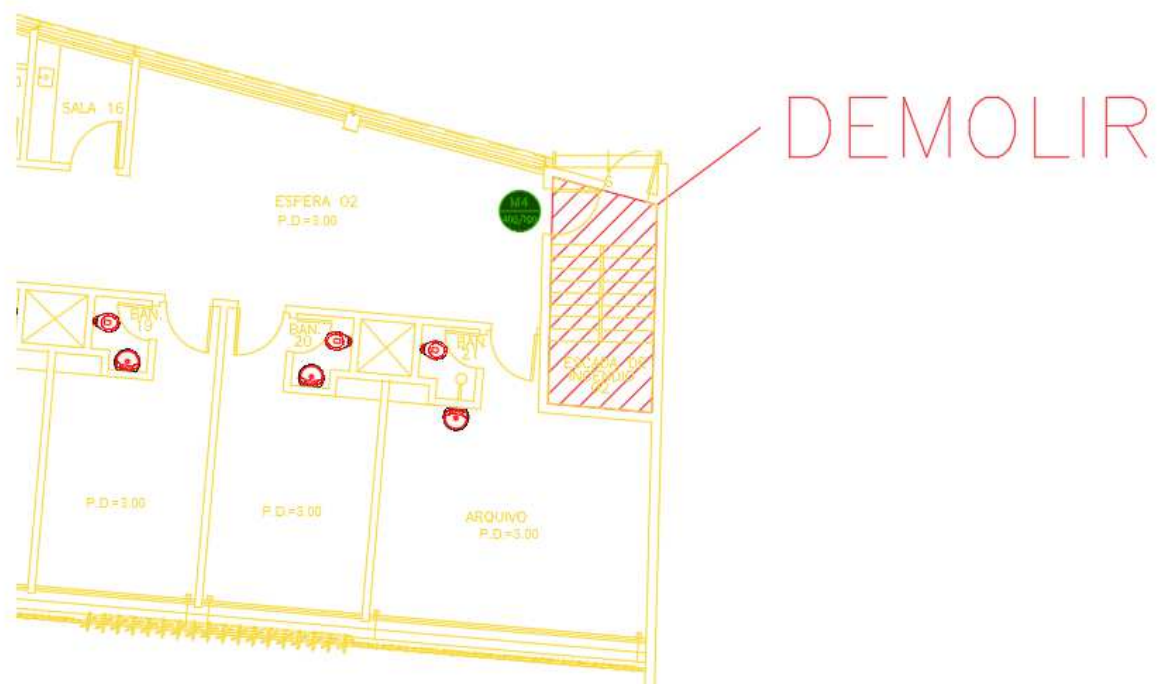
Figura 46 – LEVANTAMENTO ESTRUTURA EXISTENTE - 2º PAVIMENTO – trecho a demolir
