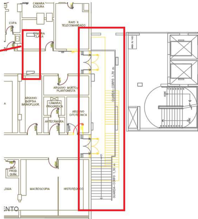
Figura 75 – NOVO CONJUNTO EMERGÊNCIA 02 – 1º PAVIMENTO – Sobreposição novo layout x escada existente á demolir (amarelo)
