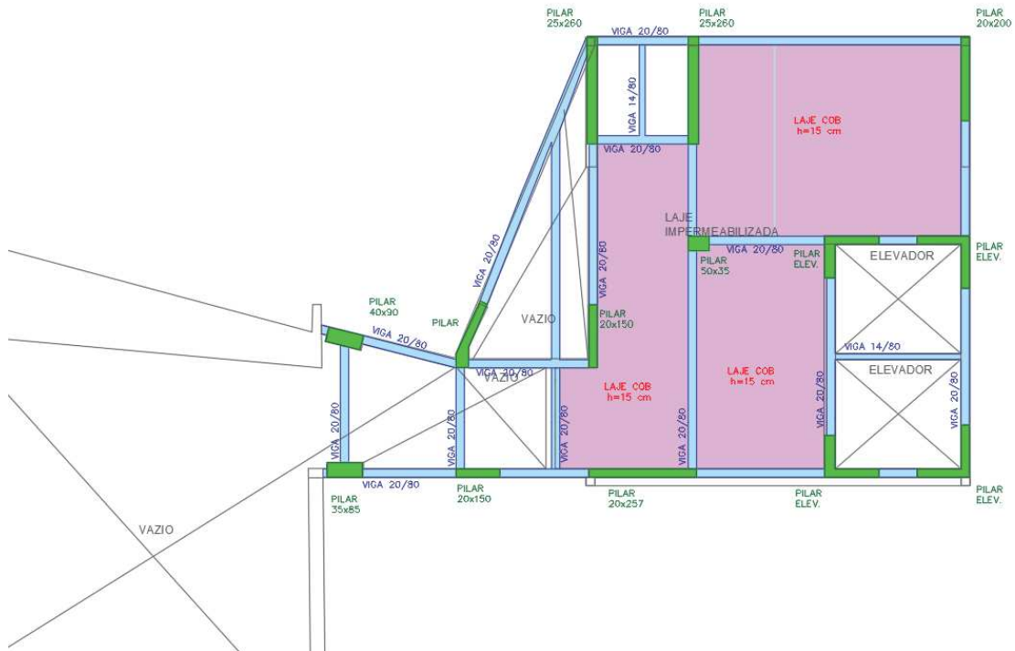
Figura 68 – NOVO CONJUNTO EMERGÊNCIA 01 – COBERTURA – Croqui Estrutura
