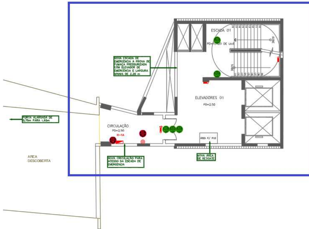
Figura 62 – NOVO CONJUNTO EMERGÊNCIA 01 – 10º PAVIMENTO - Novo Layout
