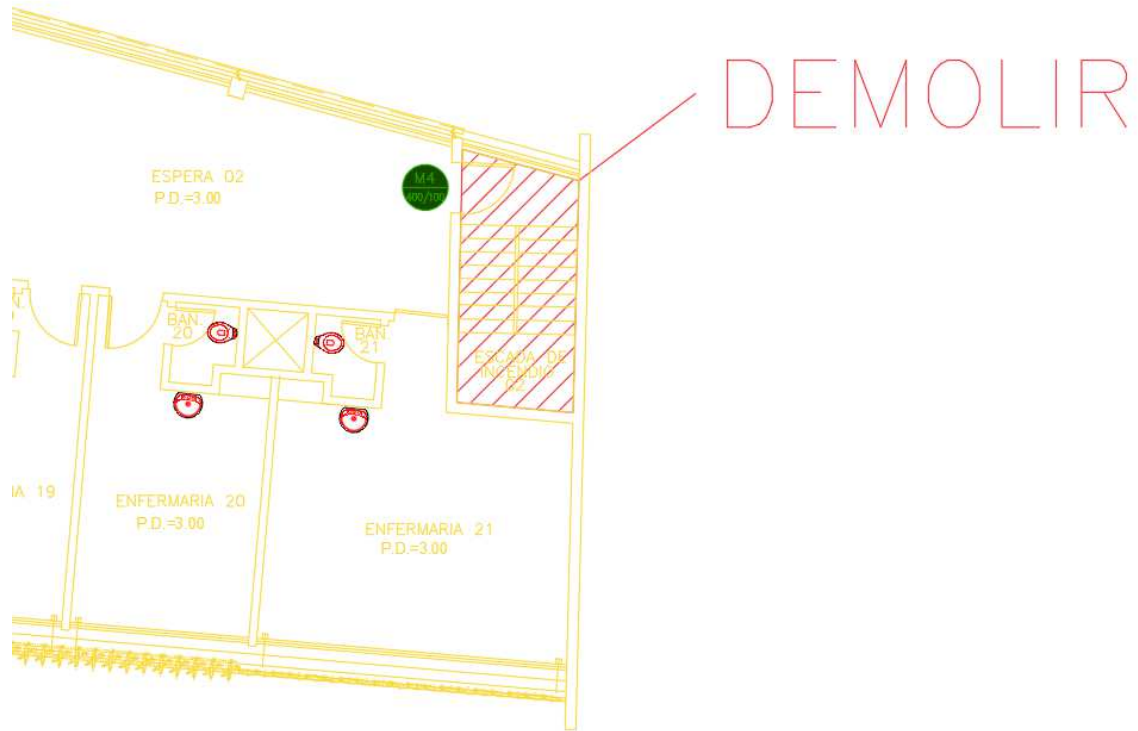
Figura 52 – LEVANTAMENTO ESTRUTURA EXISTENTE - 5º PAVIMENTO – trecho a demolir
