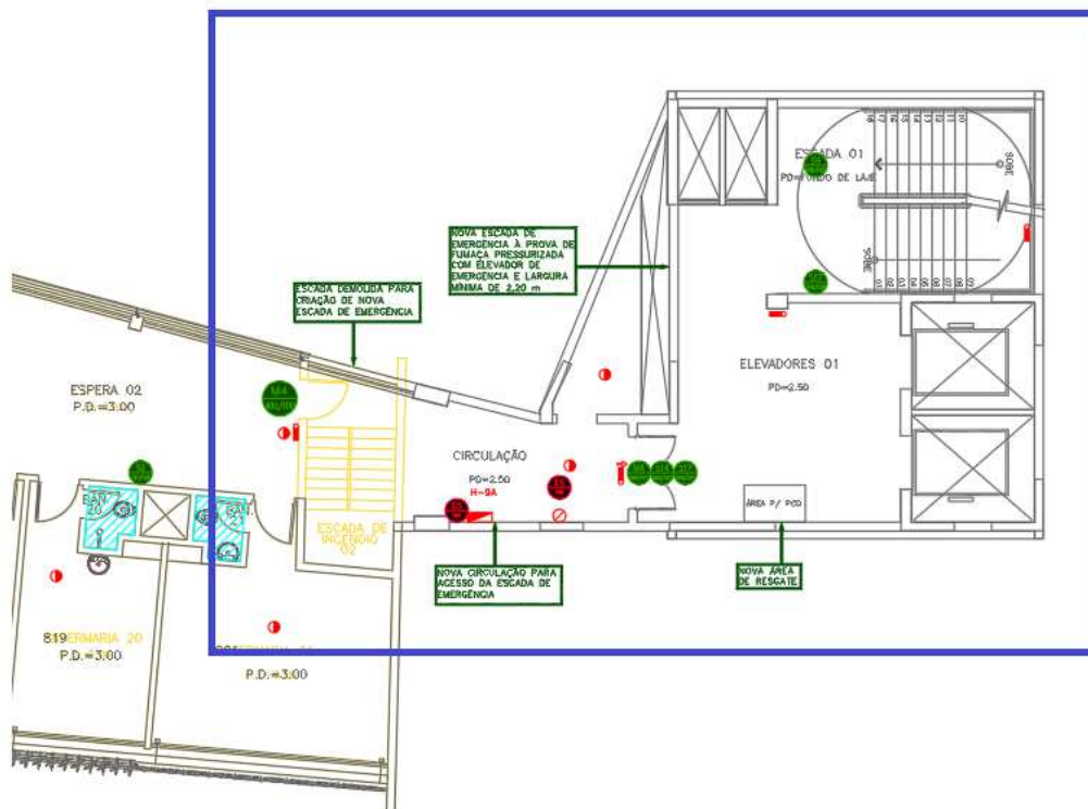
Figura 59 – NOVO CONJUNTO EMERGENCIA 01 – 8º PAVIMENTO - Novo Layout (em amarelo escada existente a ser demolida e fechada)
