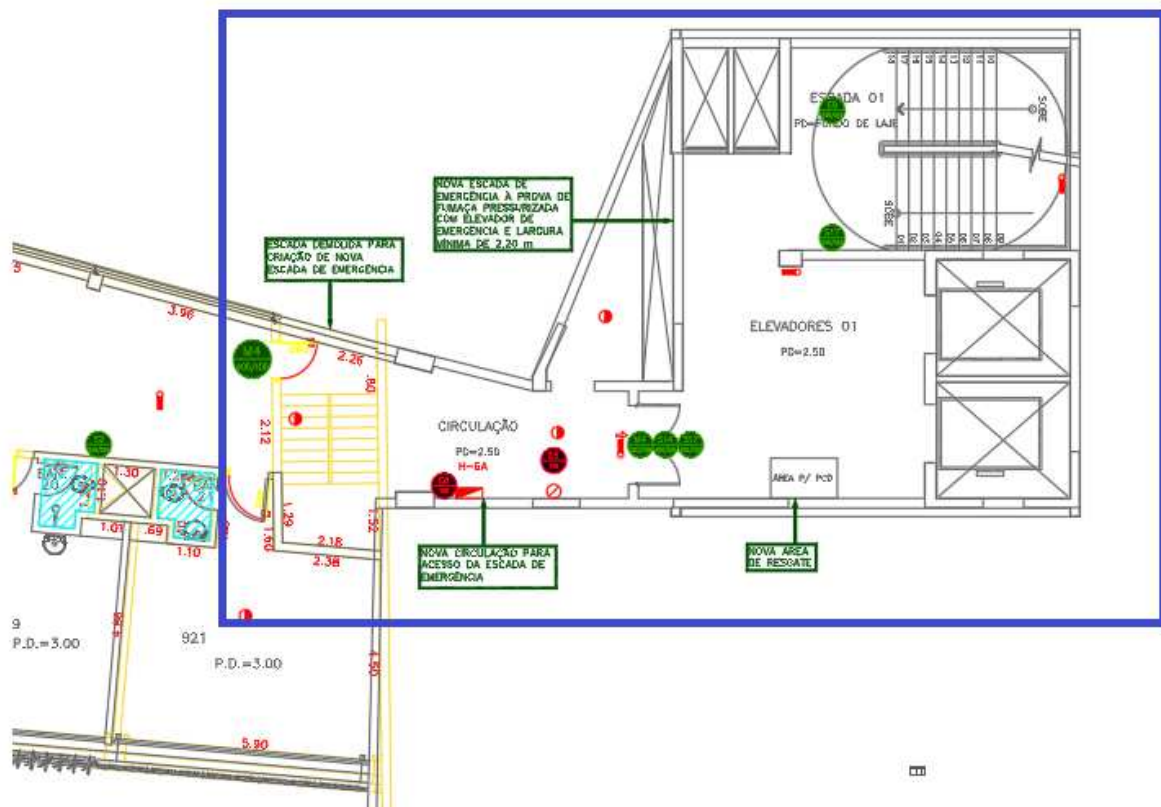
Figura 61 – NOVO CONJUNTO EMERGÊNCIA 01 – 9º PAVIMENTO - Novo Layout (em amarelo escada existente a ser demolida e fechada)
