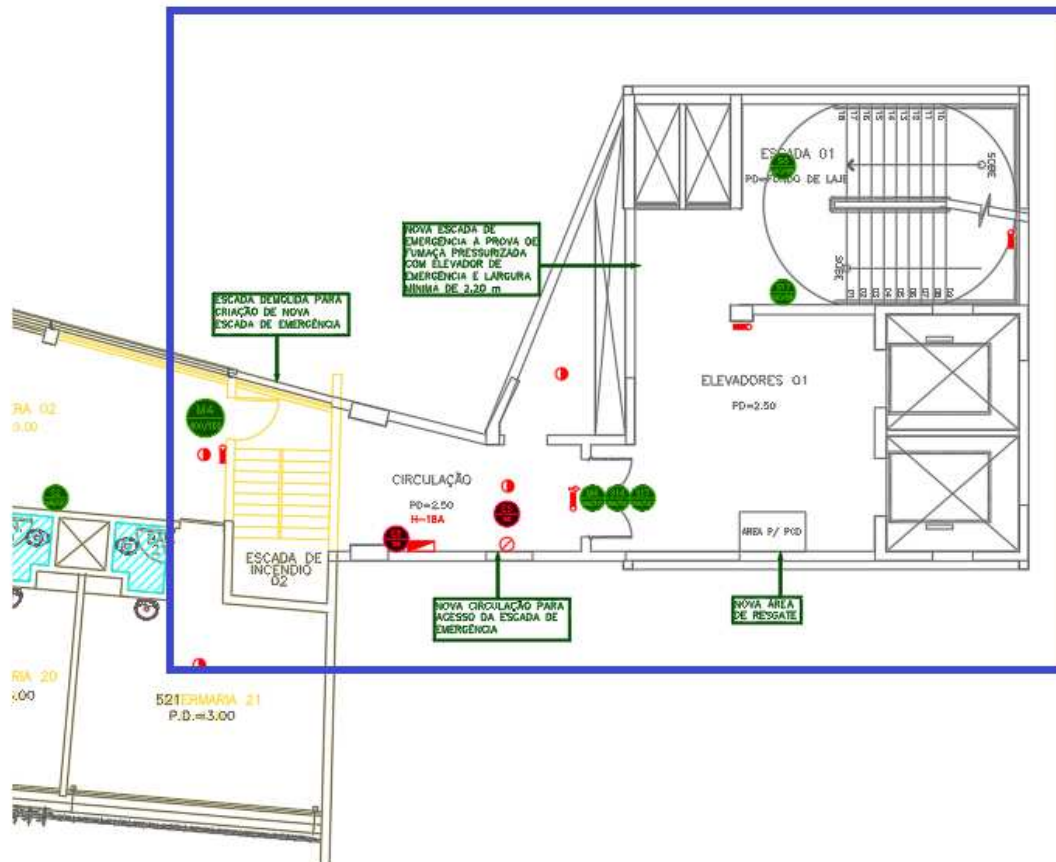
Figura 53 – NOVO CONJUNTO EMERGÊNCIA 01 – 5º PAVIMENTO - Novo Layout (em amarelo escada existente a ser demolida e fechada)
