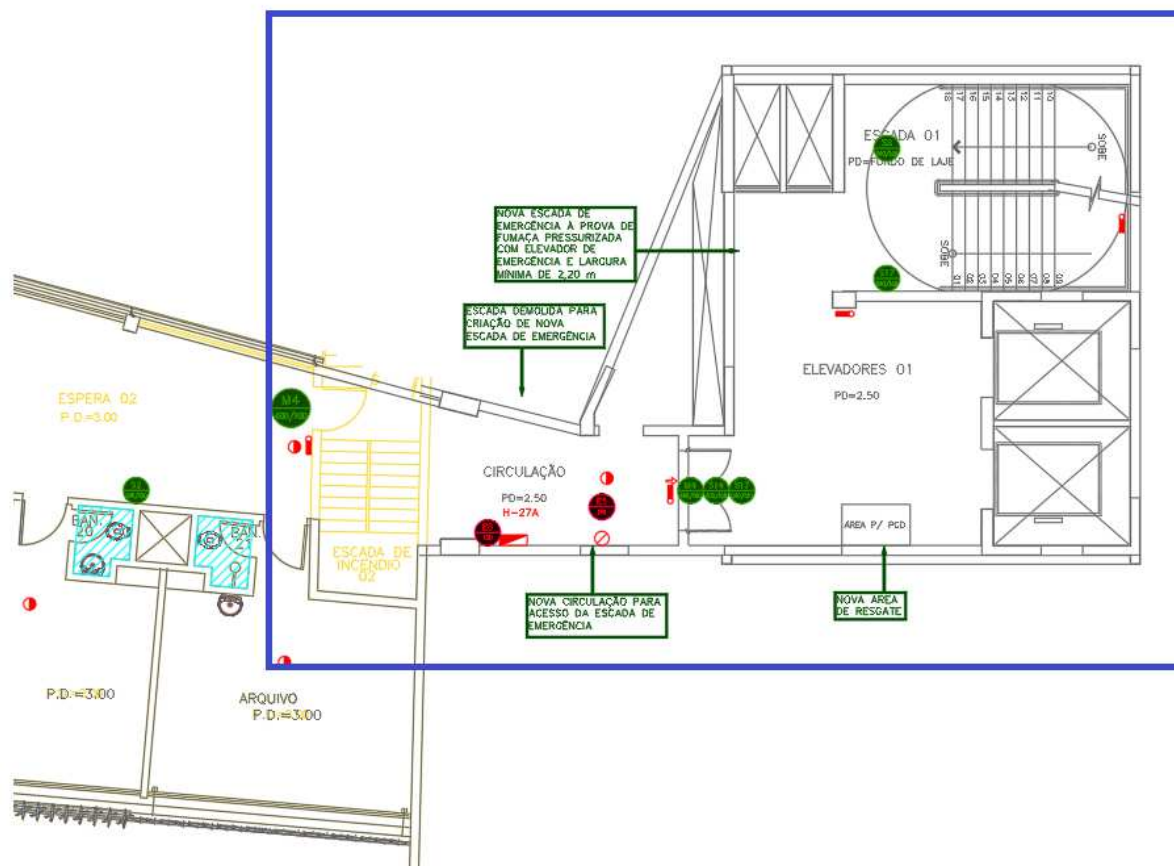
Figura 47 – NOVO CONJUNTO EMERGÊNCIA 01 – 2º PAVIMENTO – Novo Layout (em amarelo escada existente a ser demolida e fechada)
