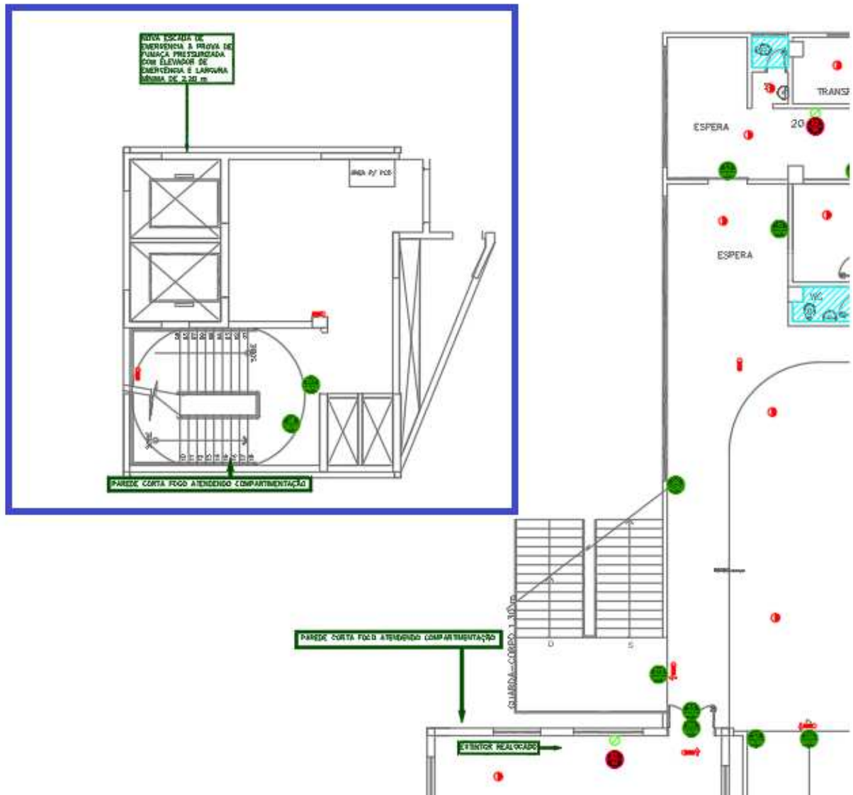
Figura 45 – NOVO CONJUNTO EMERGÊNCIA 01 – 1ºPAVIMENTO - Layout
