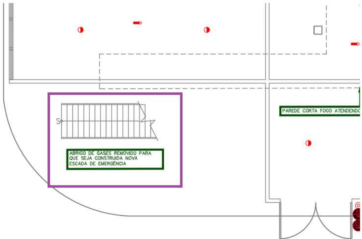
Figura 39 – NOVA ESCADA METÁLICA 02 – TÉRREO – Layout da saída da escada
