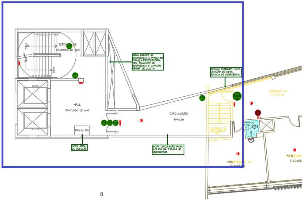
Figura 85 – NOVO CONJUNTO EMERGENCIA 02 – 5º PAVIMENTO - Novo Layout (em amarelo escada existente a ser demolida e fechada)
