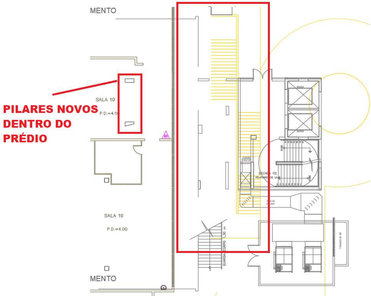
Figura 73 – NOVO CONJUNTO EMERGÊNCIA 02 – TÉRREO – Sobreposição novo layout x escada existente á demolir (amarelo)
