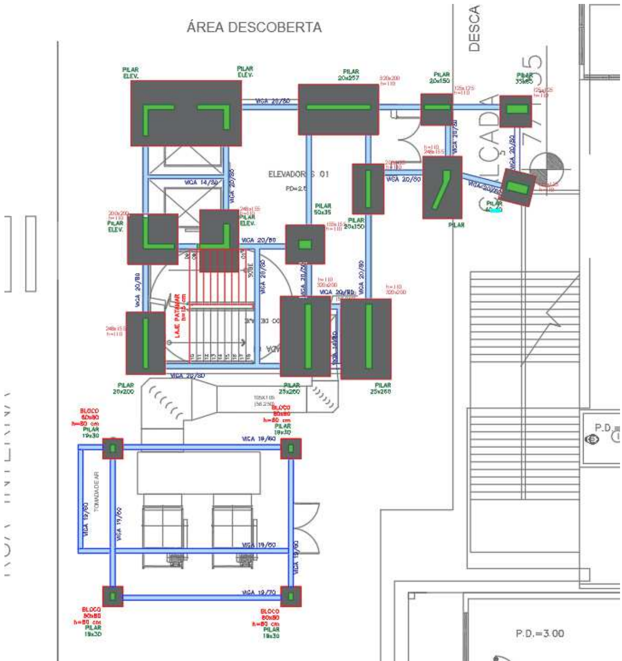
Figura 64 – NOVO CONJUNTO EMERGÊNCIA 01 – TÉRREO – Croqui Estrutura
