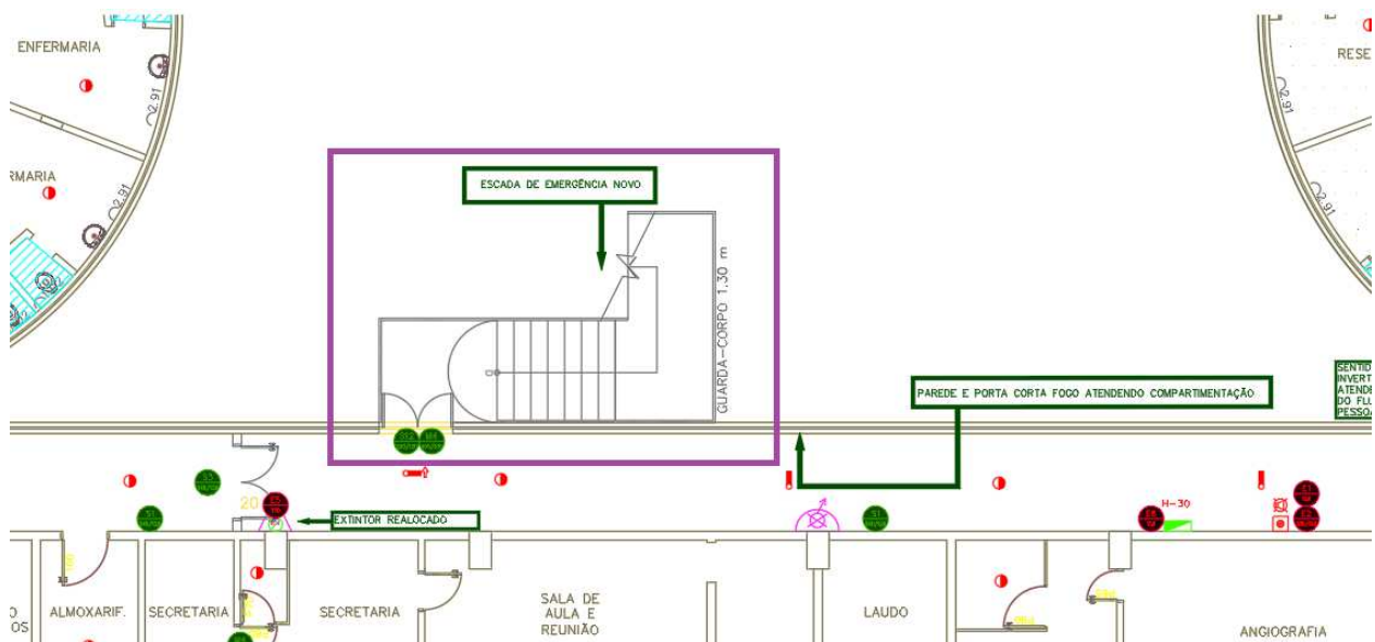
Figura 34 – NOVA ESCADA METÁLICA 01 – 1º PAVIMENTO - Layout da chegada da nova escada metálica externa
