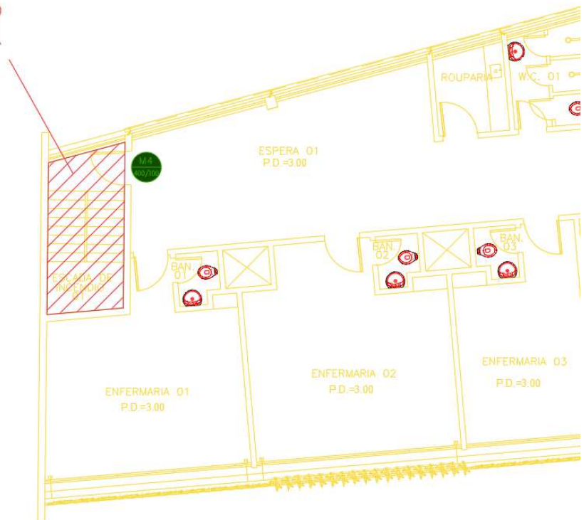
Figura 86 – LEVANTAMENTO ESTRUTURA EXISTENTE - 6º PAVIMENTO – trecho a demolir
