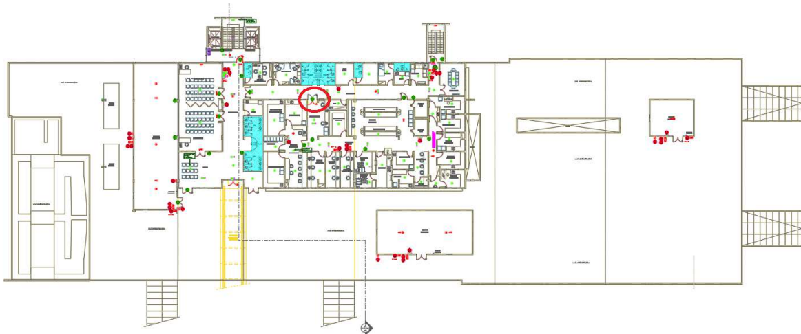
Figura 14 –AMBULATÓRIO – 1º PAVIMENTO – Inversão sentido de porta
