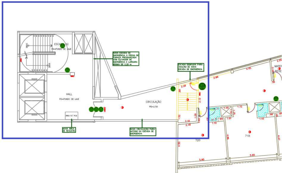
Figura 89 – NOVO CONJUNTO EMERGENCIA 02 – 7º PAVIMENTO - Novo Layout (em amarelo escada existente a ser demolida e fechada)
