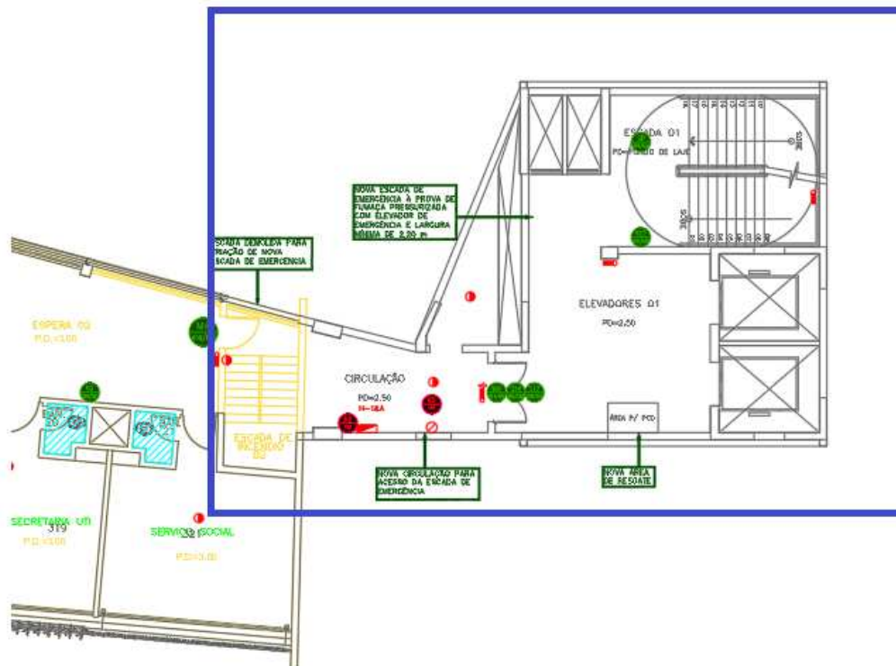
Figura 49 – NOVO CONJUNTO EMERGÊNCIA 01 – 3º PAVIMENTO - Novo Layout (em amarelo escada existente a ser demolida e fechada)
