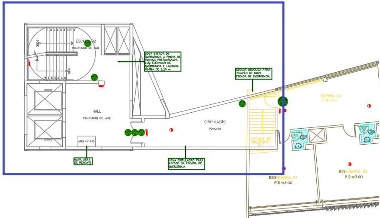
Figura 91 – NOVO CONJUNTO EMERGÊNCIA 02 – 8º PAVIMENTO - Novo Layout (em amarelo escada existente a ser demolida e fechada)
