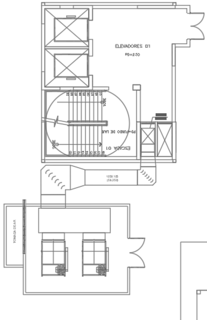
Figura 17 – CONJUNTO 01 – Paredes fechamento escada e casa de máquinas
