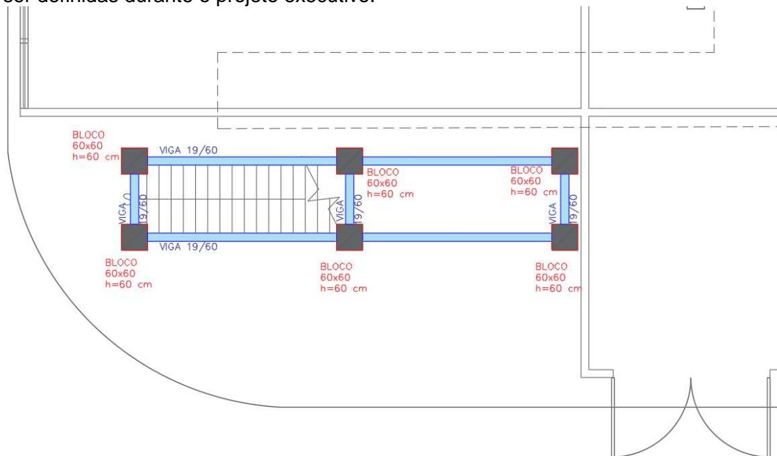
Figura 41 – NOVA ESCADA METÁLICA 02 – TÉRREO – Croqui estrutura
