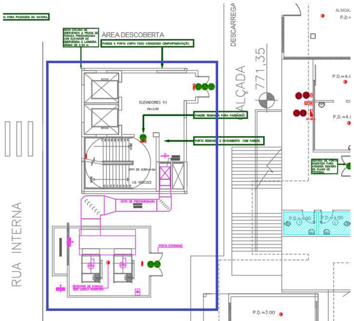
Figura 44 – NOVO CONJUNTO EMERGÊNCIA 01 – TÉRREO - Layout da saída da escada + casa de máquinas
