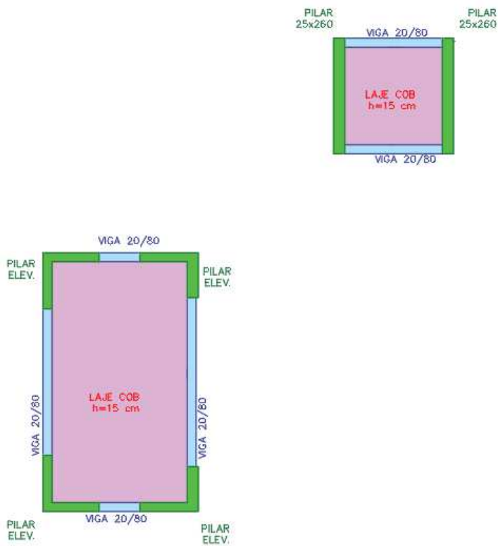
Figura 101 – NOVO CONJUNTO EMERGÊNCIA 02 – COBERTURA C.MÁQ ELEV.- Croqui Estrutura
