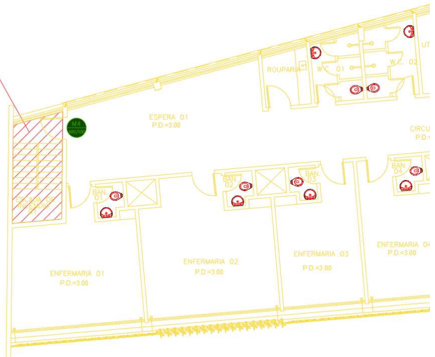
Figura 89 – NOVO CONJUNTO EMERGENCIA 02 – 7º PAVIMENTO - Novo Layout (em amarelo escada existente a ser demolida e fechada)
