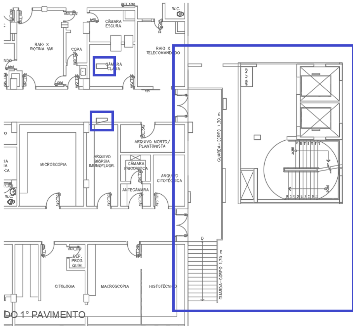
Figura 77 – NOVO CONJUNTO EMERGÊNCIA 02 – 1º PAVIMENTO - Layout
