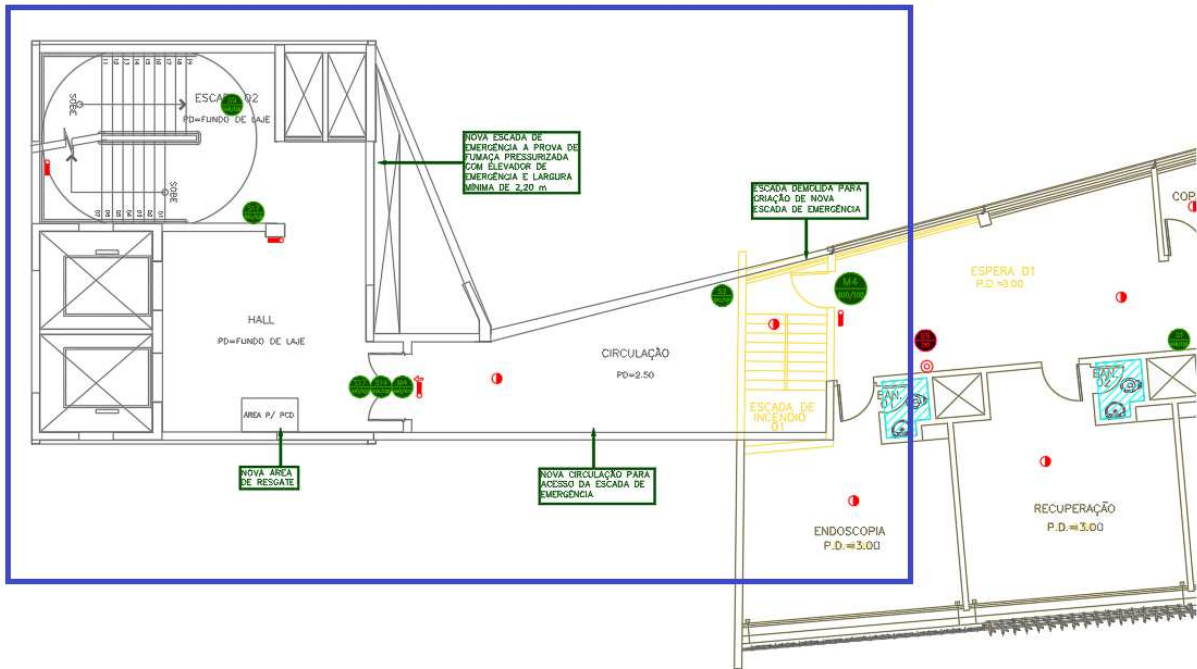
Figura 79 – NOVO CONJUNTO EMERGÊNCIA 02 – 2º PAVIMENTO - Novo Layout (em amarelo escada existente a ser demolida e fechada)
