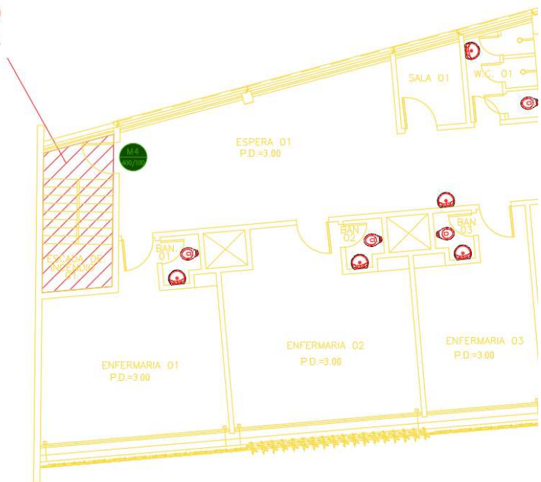
Figura 82 – LEVANTAMENTO ESTRUTURA EXISTENTE - 4º PAVIMENTO – trecho a demolir
