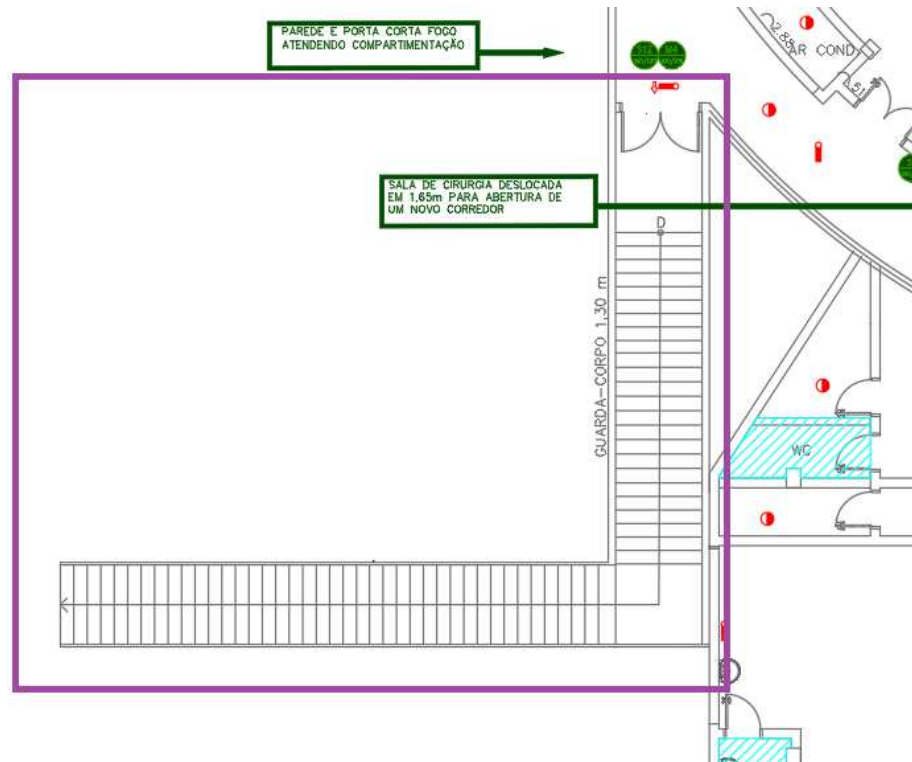
Figura 40 – NOVA ESCADA METÁLICA 02 – 1º PAVIMENTO - Layout da chegada da nova escada metálica externa
