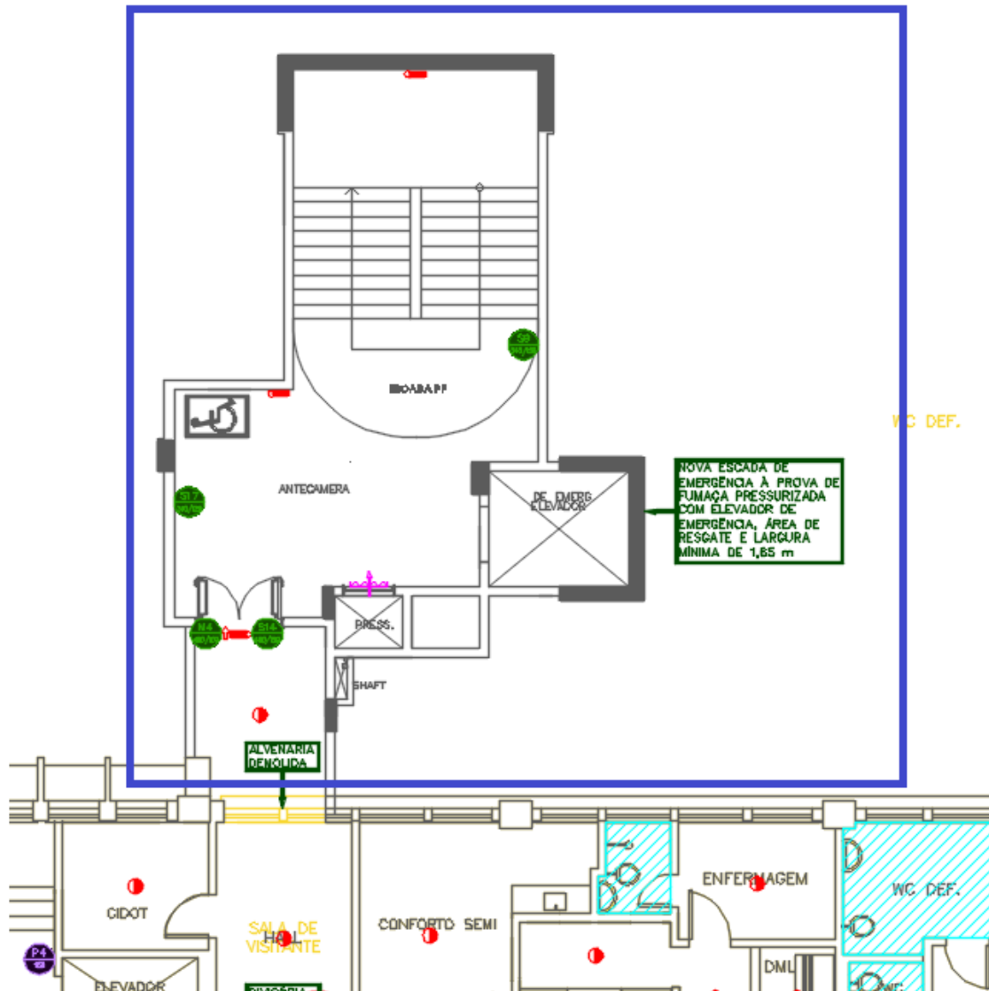
Figura 88 – 4º PAVIMENTO– CONJUNTO EMERGÊNCIA 02 – Novo layout
