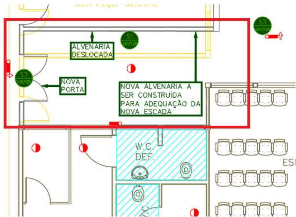
Figura 32 – 1º PAVIMENTO – Demolição(amarelo)/reconstrução paredes para mudança de layout
