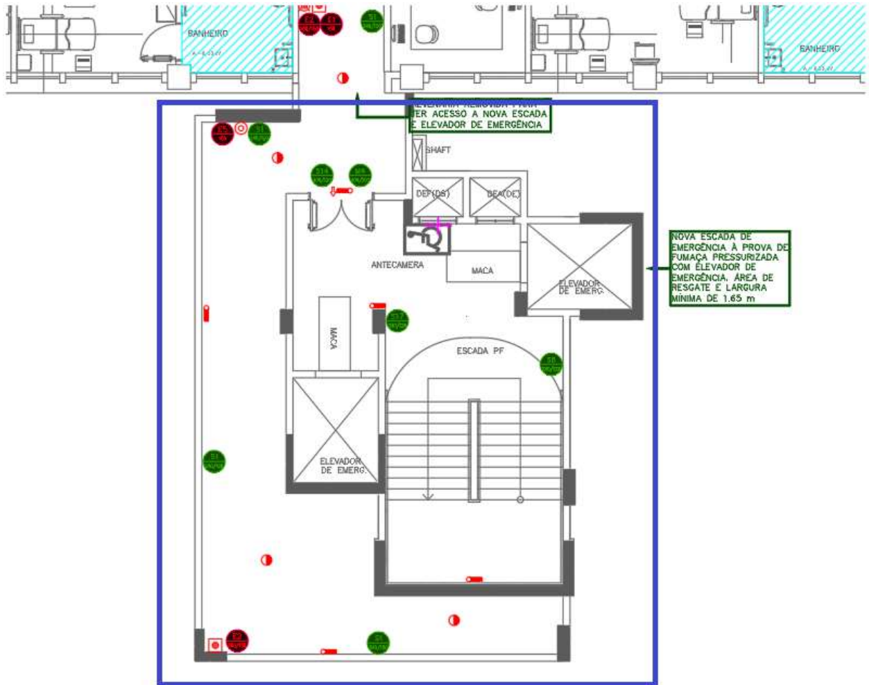
Figura 72 – 8º PAVIMENTO– CONJUNTO EMERGÊNCIA 01 – Novo layout
