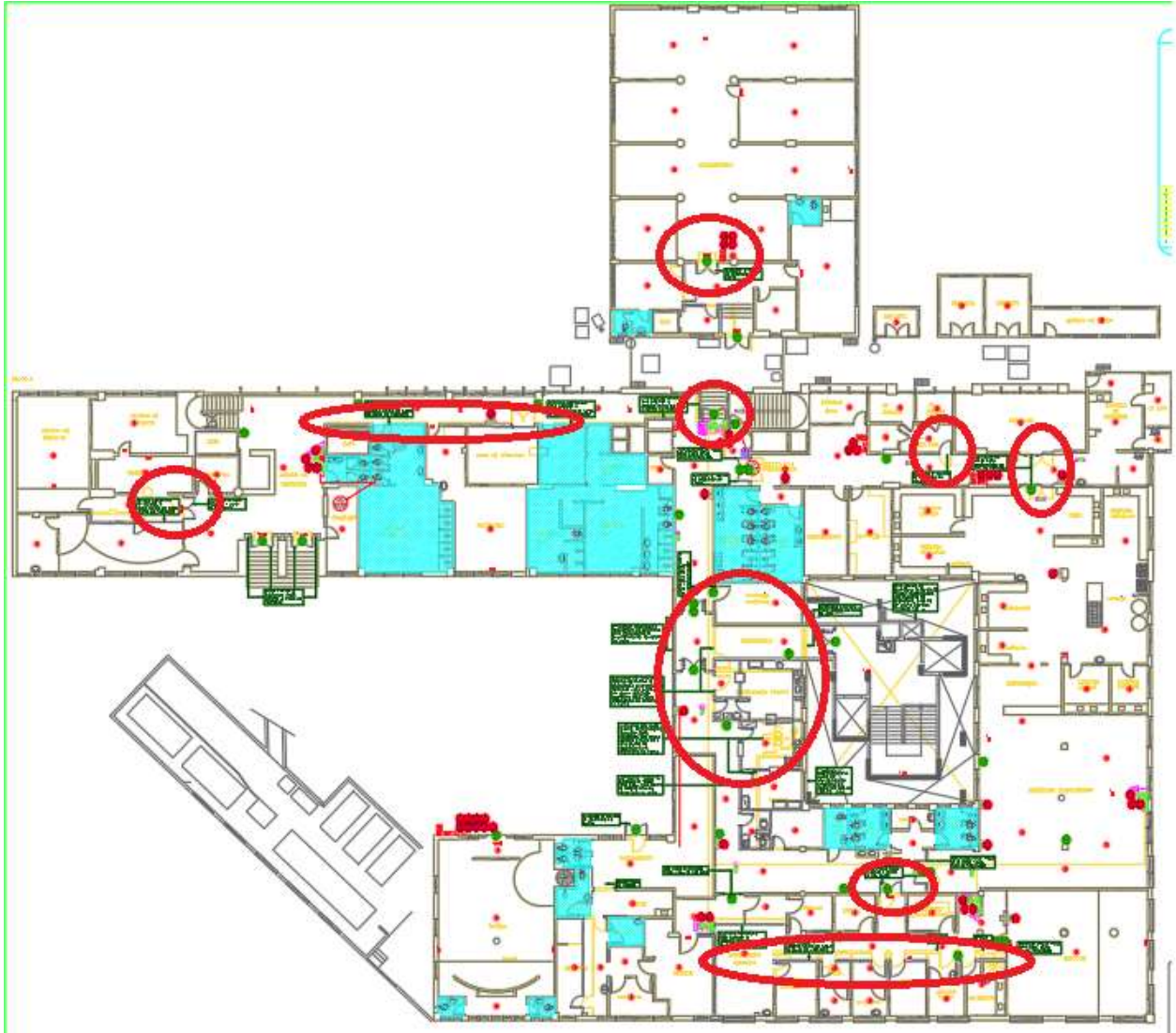
Figura 10 – 1º SUBSOLO – Inversão no sentido de porta/Remoção e instalação de novas portas
