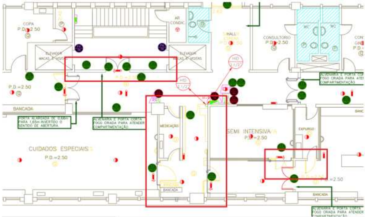
Figura 42 – 7º PAVIMENTO – Demolição(amarelo)/reconstrução paredes para mudança de layout
