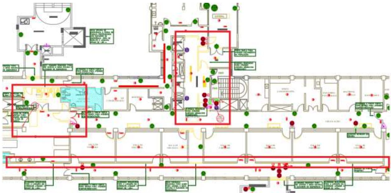
Figura 41 – 6º PAVIMENTO – Demolição(amarelo)/reconstrução paredes para mudança de layout
