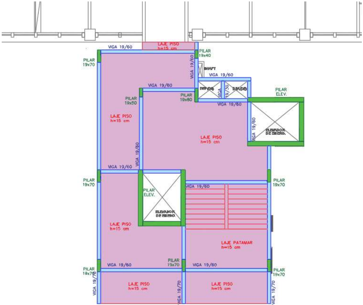
Figura 80 – 2º ao 11º PAVIMENTO – CONJUNTO EMERGÊNCIA 01 – Croqui Estrutura Tipo
