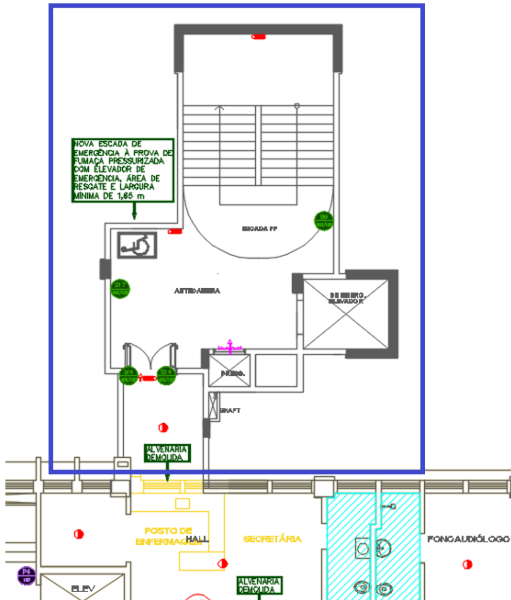
Figura 86 – 2º PAVIMENTO– CONJUNTO EMERGÊNCIA 02 – Novo layout
