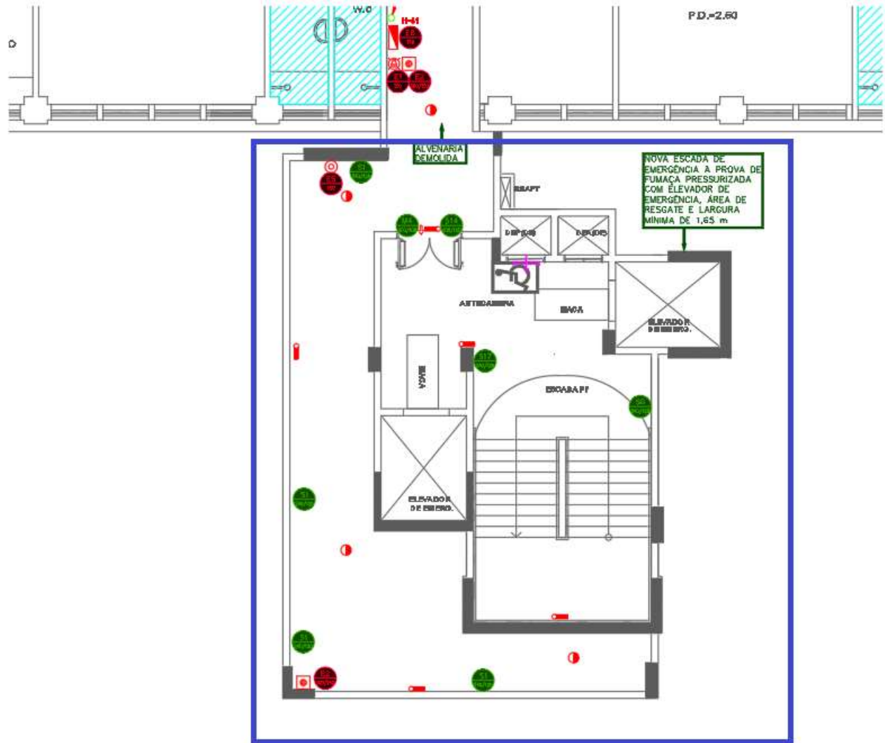
Figura 67 – 3º PAVIMENTO– CONJUNTO EMERGÊNCIA 01 – Novo layout
