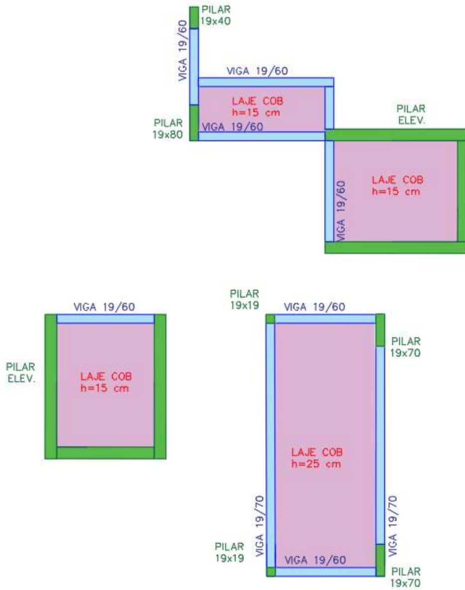
Figura 82 – COBERTURA ESCADA E C.MÁQ ELEV – CONJUNTO EMERGÊNCIA 01 – Croqui Estrutura
