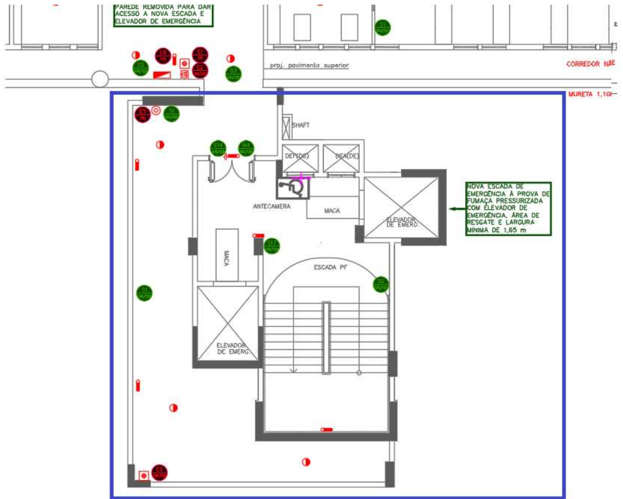
Figura 75 – 11º PAVIMENTO– CONJUNTO EMERGÊNCIA 01 – Novo layout
