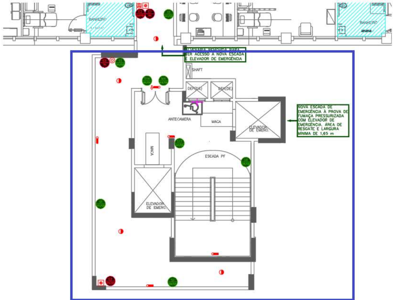
Figura 73 – 9º PAVIMENTO– CONJUNTO EMERGÊNCIA 01 – Novo layout
