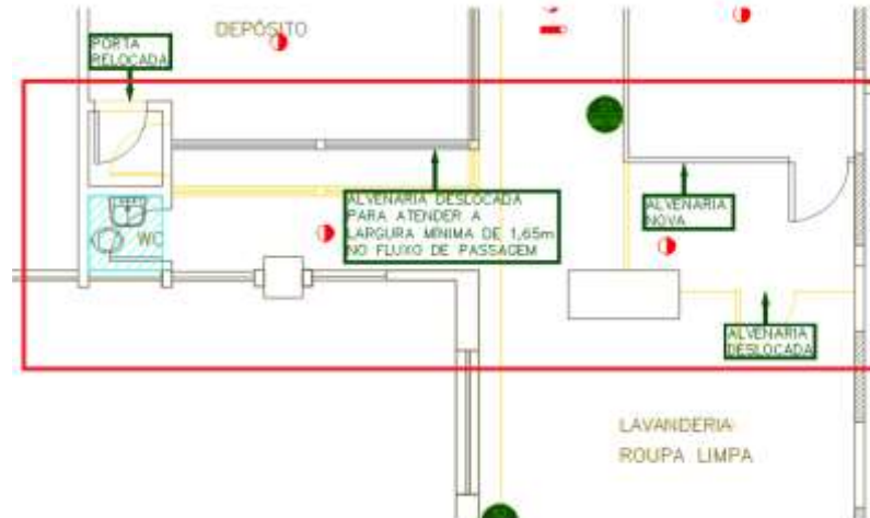
Figura 22 – 2º SUBSOLO – Demolição(amarelo)/reconstrução paredes
