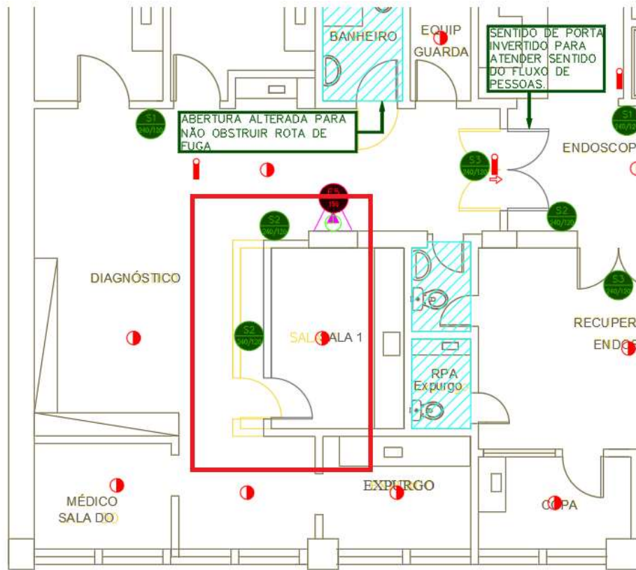
Figura 40 – 6º PAVIMENTO – Demolição(amarelo)/reconstrução paredes para mudança de layout
