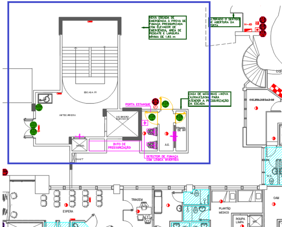
Figura 85 – 1º PAVIMENTO– CONJUNTO EMERGENCIA 02 – Novo layout
