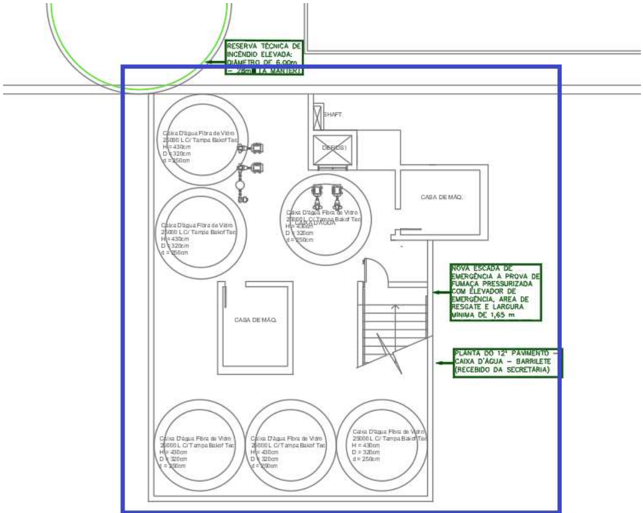
PLANTA DÉCIMO SEGUNDO PAVIMENTO - CAIXA D'ÁGUA-BARRILETE ESC. 1:75
