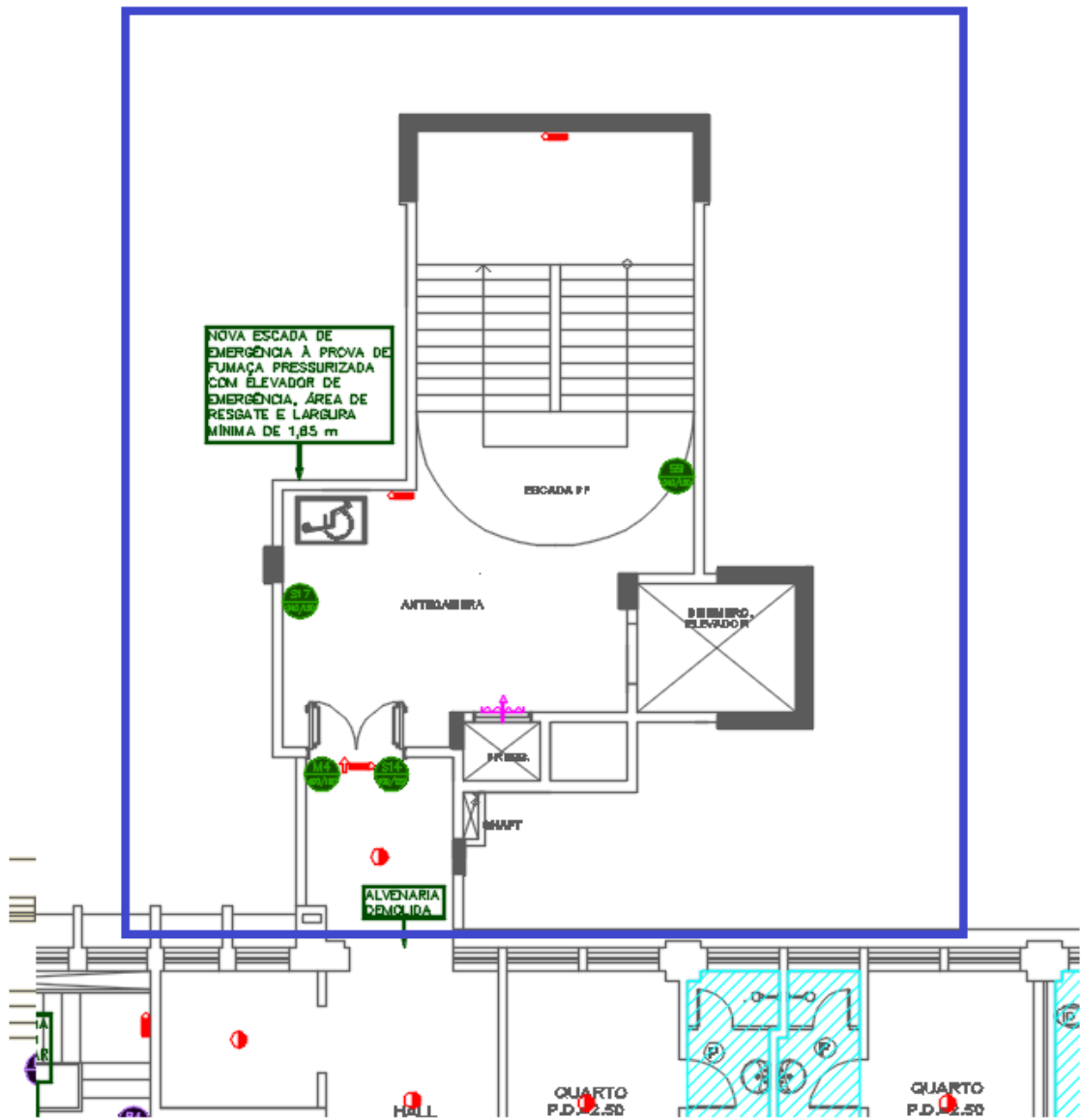
Figura 87 – 3º PAVIMENTO– CONJUNTO EMERGÊNCIA 02 – Novo layout
