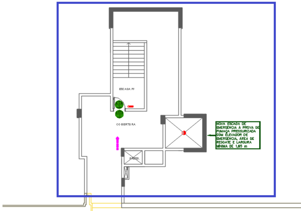
Figura 96 – COBERTURA– CONJUNTO EMERGÊNCIA 02 – Novo layout
