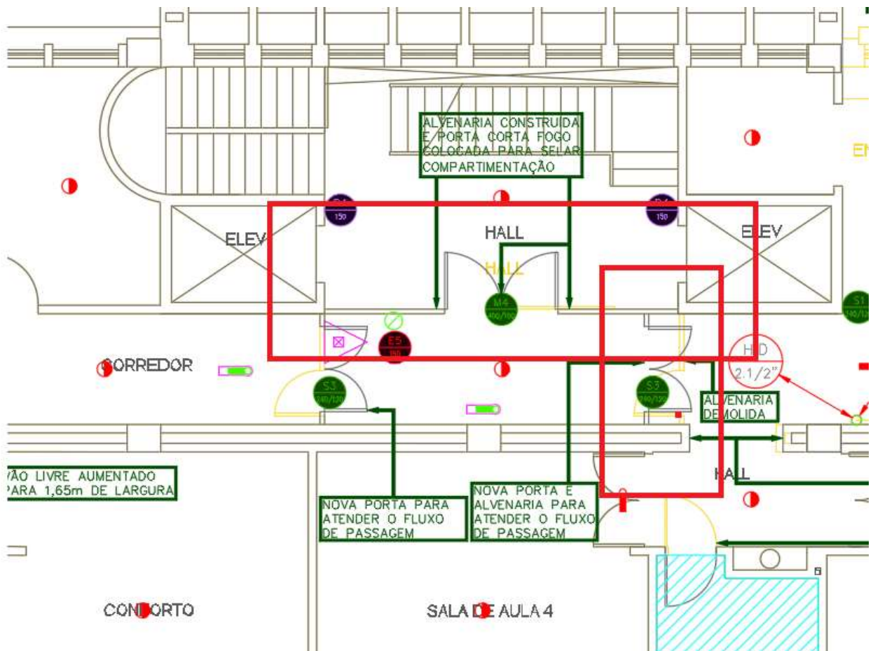
Figura 33 – 2º PAVIMENTO – Demolição(amarelo)/reconstrução paredes para mudança de layout
