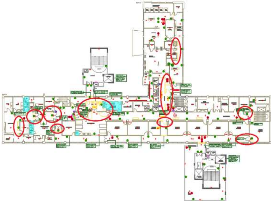
Figura 16 – 6º PAVIMENTO – Inversão no sentido de porta/Remoção e instalação de novas portas
