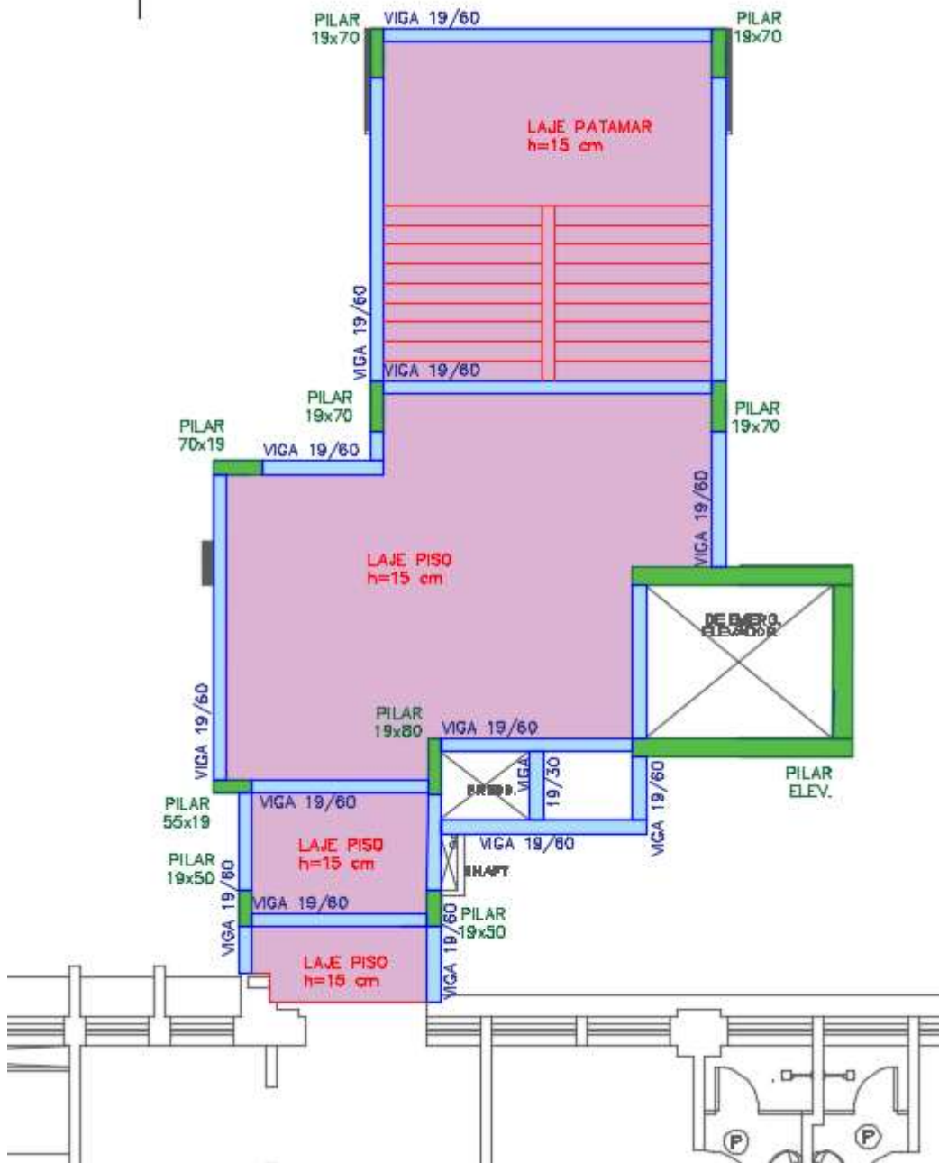
Figura 99 – 3º PAVIMENTO AO 11º PAVIMENTO– CONJUNTO EMERGÊNCIA 02 – Croqui Estrutura Tipo
