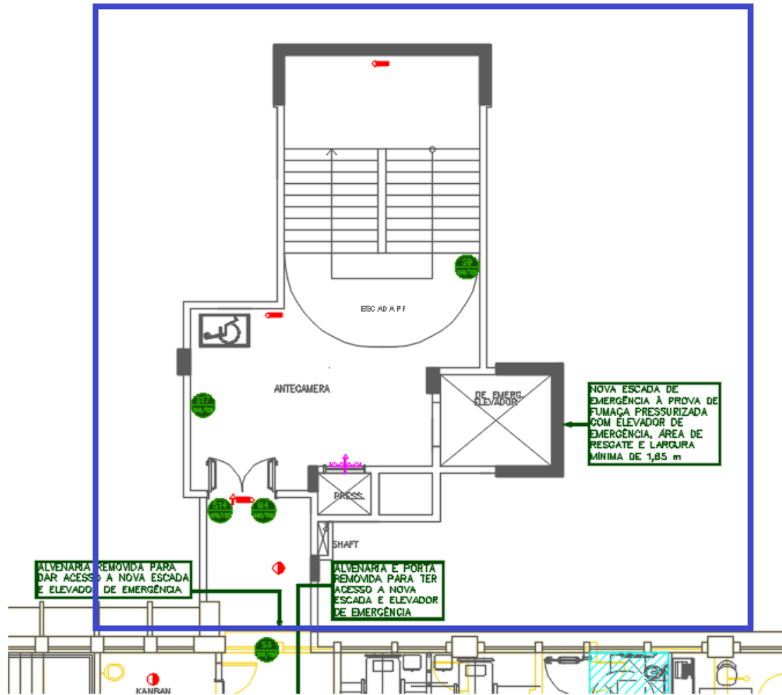
Figura 94 – 10º PAVIMENTO– CONJUNTO EMERGÊNCIA 02 – Novo layout
