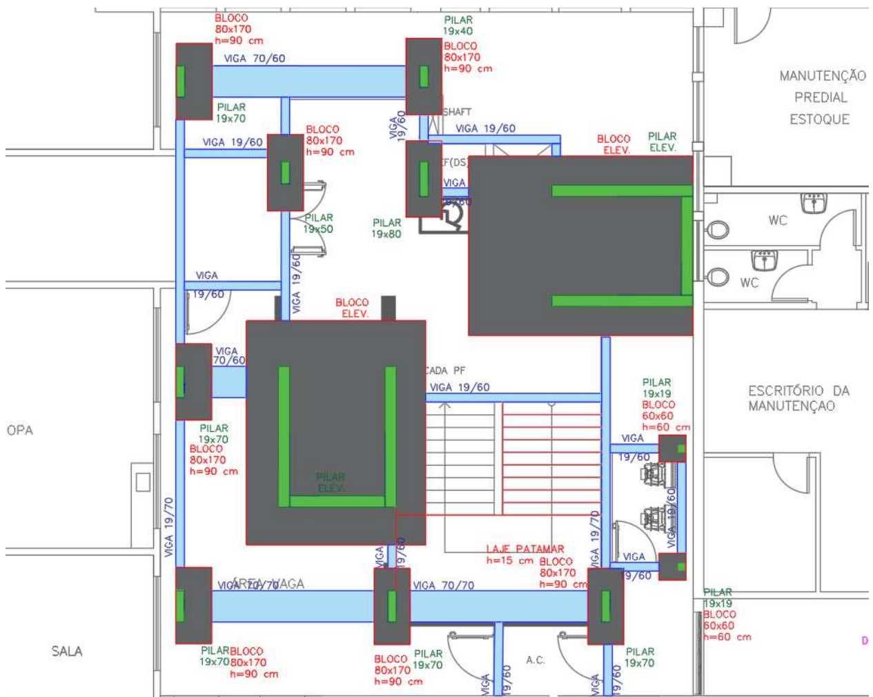
Figura 77 – 2º SUBSOLO – CONJUNTO EMERGÊNCIA 01 – Croqui Estrutura
