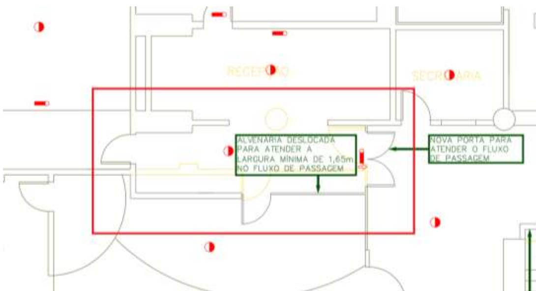
Figura 26 – 1º SUBSOLO – Demolição(amarelo)/reconstrução paredes
