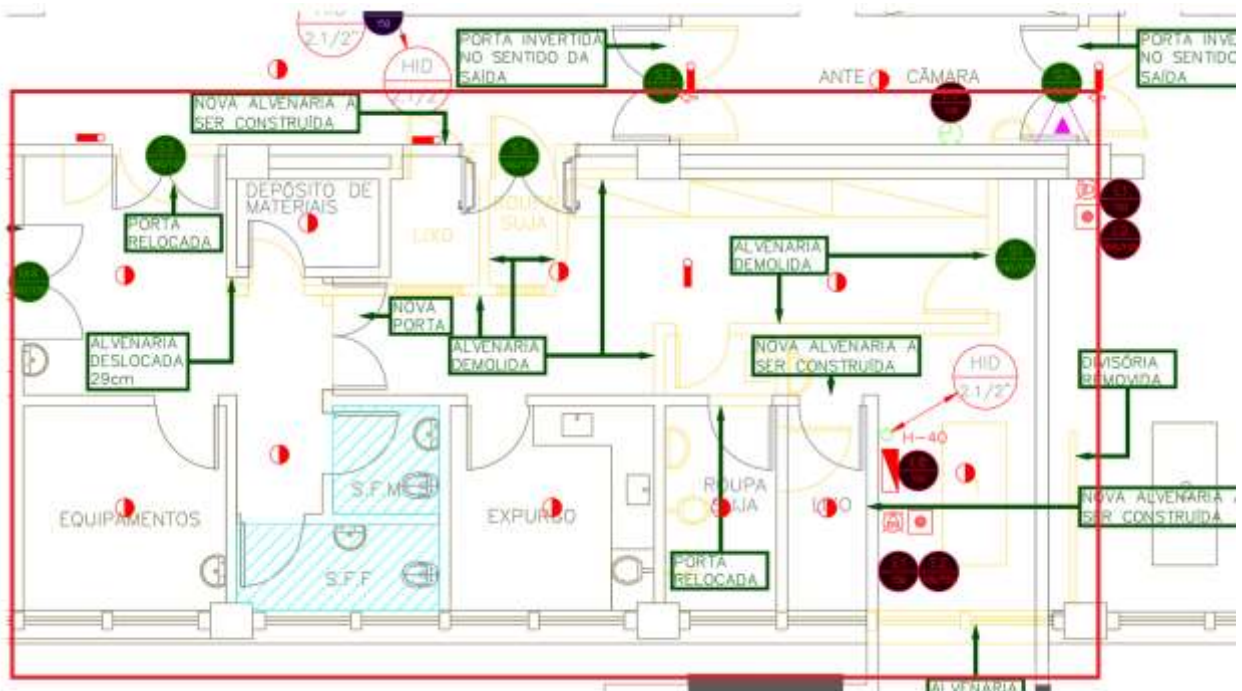
Figura 37 – 4º PAVIMENTO – Demolição(amarelo)/reconstrução paredes para mudança de layout
