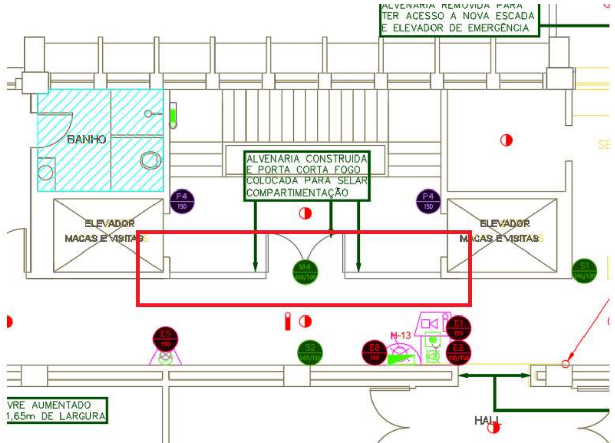
Figura 38 – 5º PAVIMENTO – construção paredes
