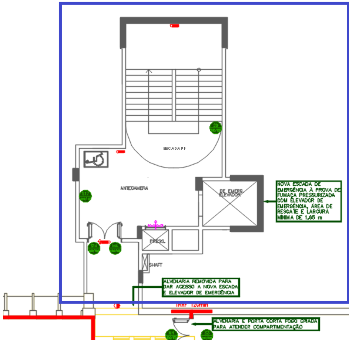
Figura 95 – 11º PAVIMENTO– CONJUNTO EMERGÊNCIA 02 – Novo layout
