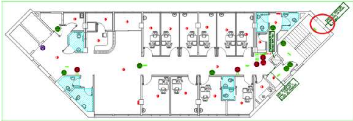
Figura 5 – AMBULATÓRIO – 3º PAVIMENTO – Instalação de nova janela
