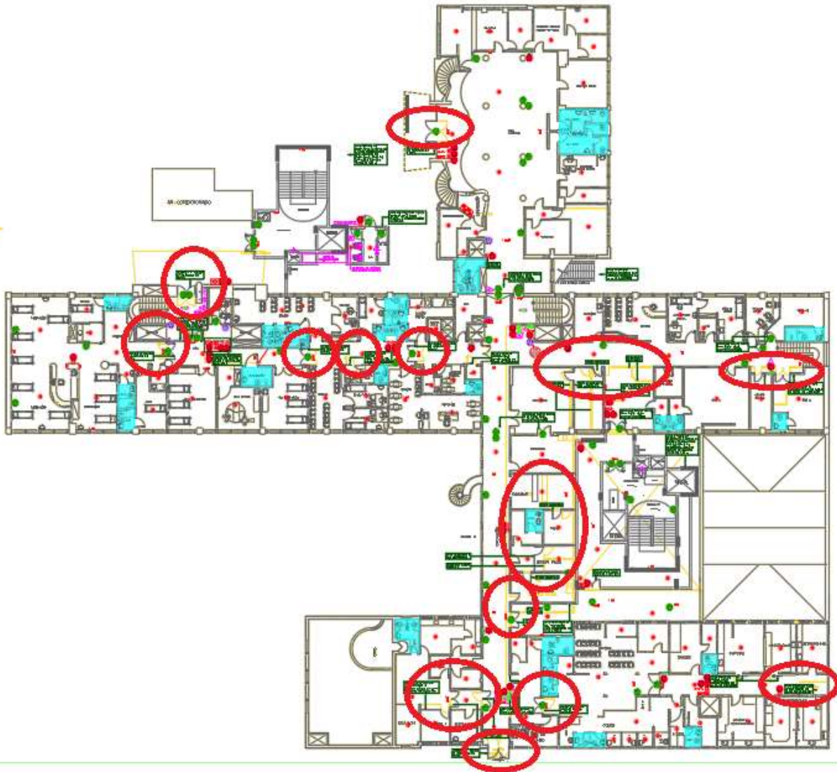
Figura 11 – 1º PAVIMENTO – Inversão no sentido de porta/Remoção e instalação de novas portas
