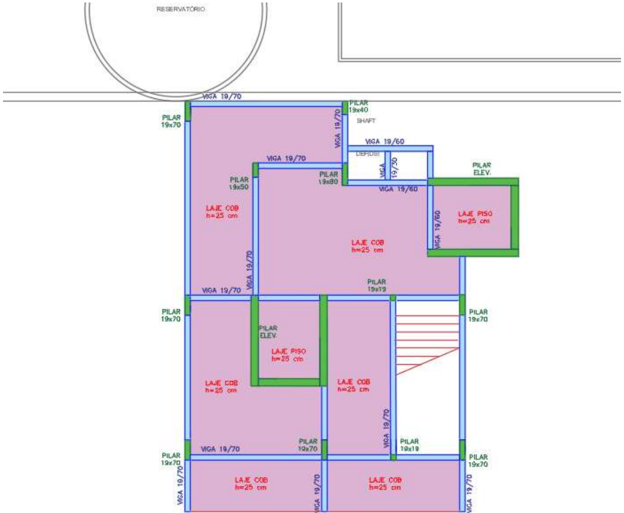
Figura 81 – COBERTURA – CONJUNTO EMERGÊNCIA 01 – Croqui Estrutura
