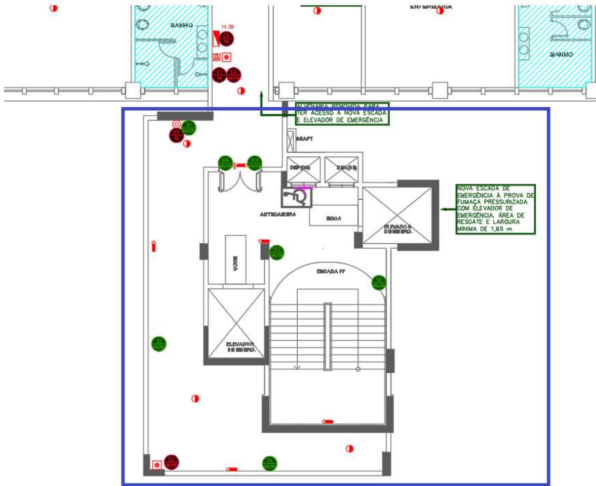
Figura 69 – 5º PAVIMENTO– CONJUNTO EMERGÊNCIA 01 – Novo layout
