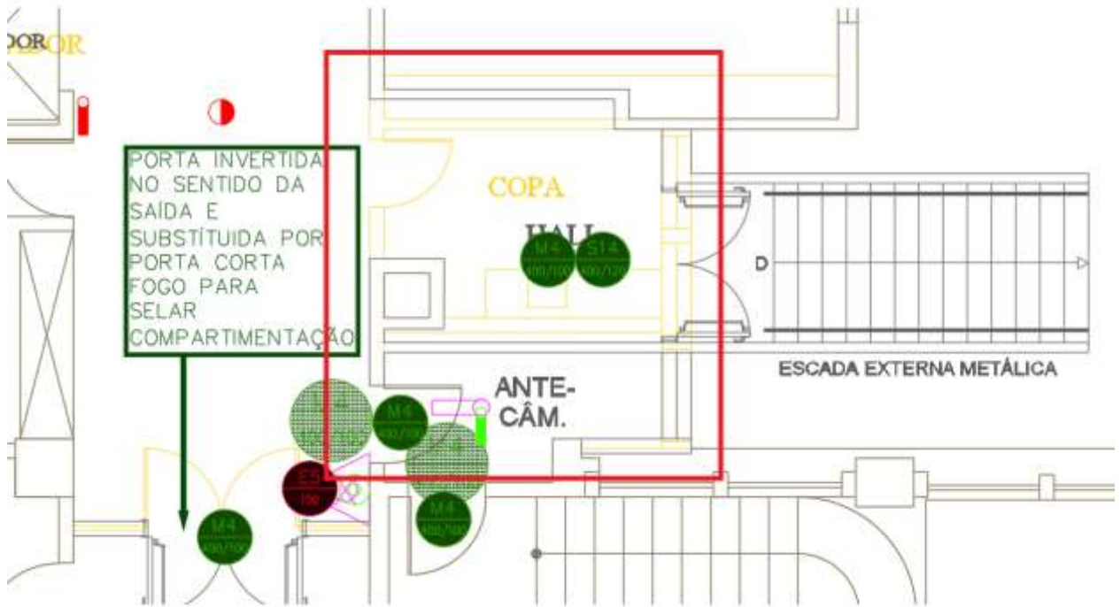
Figura 34 – 2º PAVIMENTO – Demolição(amarelo)/reconstrução paredes para mudança de layout
