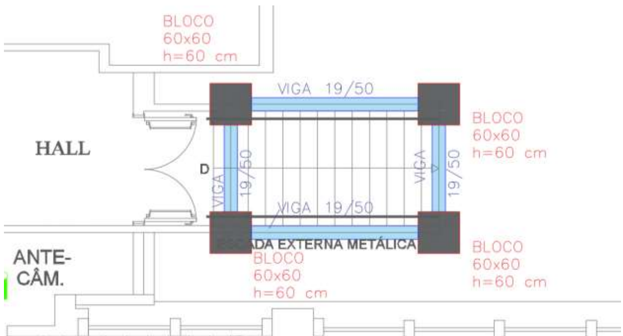
Figura 57 – ESCADA METÁLICA – 1º PAVIMENTO – Croqui estrutura
