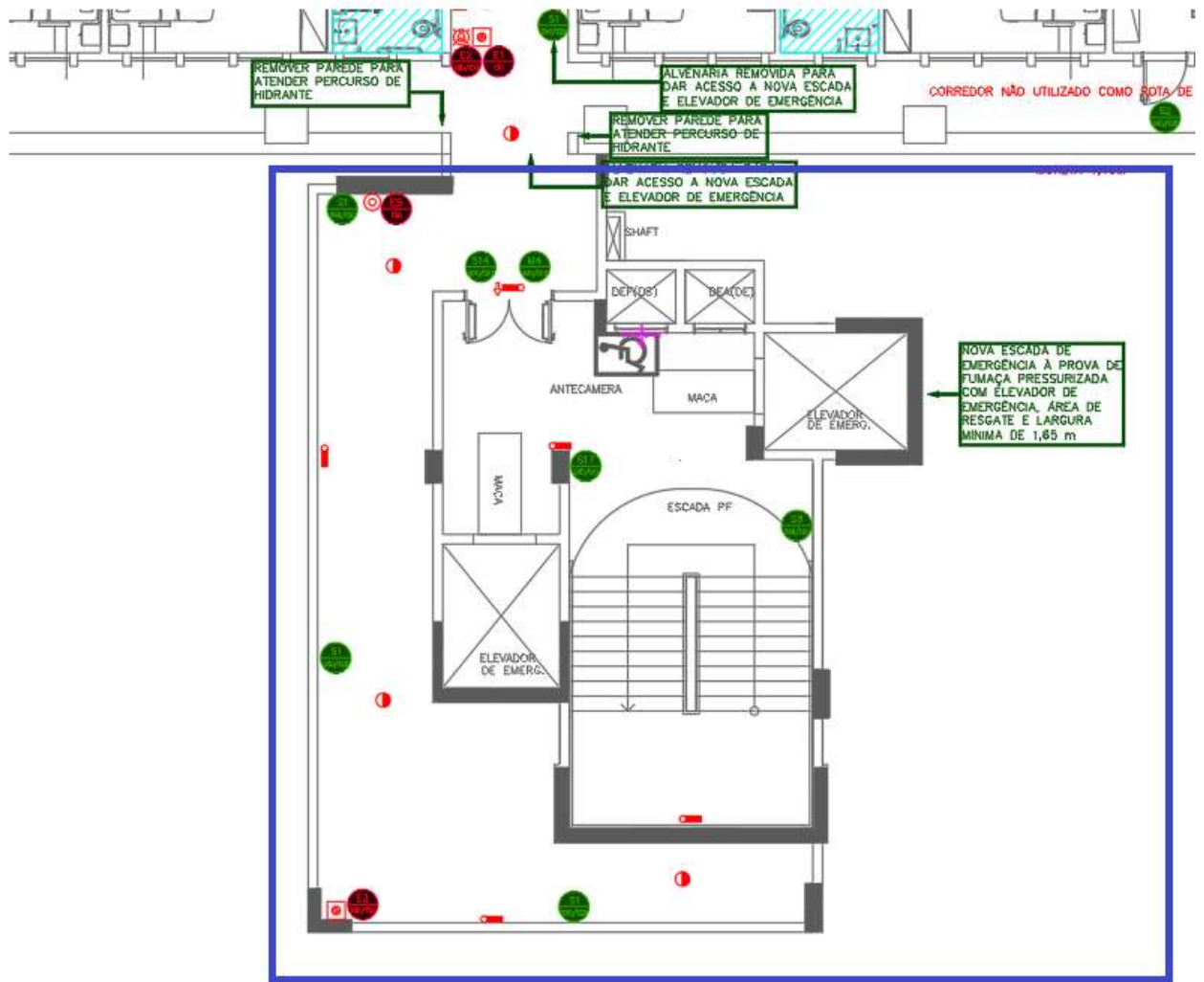
Figura 74 – 10º PAVIMENTO– CONJUNTO EMERGÊNCIA 01 – Novo layout
