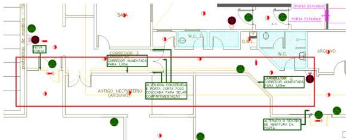
Figura 25 – 2º SUBSOLO – Demolição(amarelo)/reconstrução paredes
