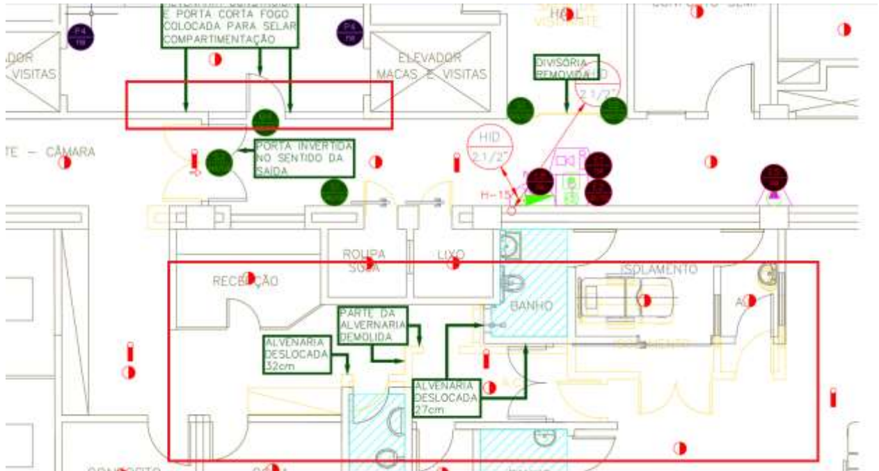
Figura 36 – 4º PAVIMENTO – Demolição(amarelo)/reconstrução paredes para mudança de layout
