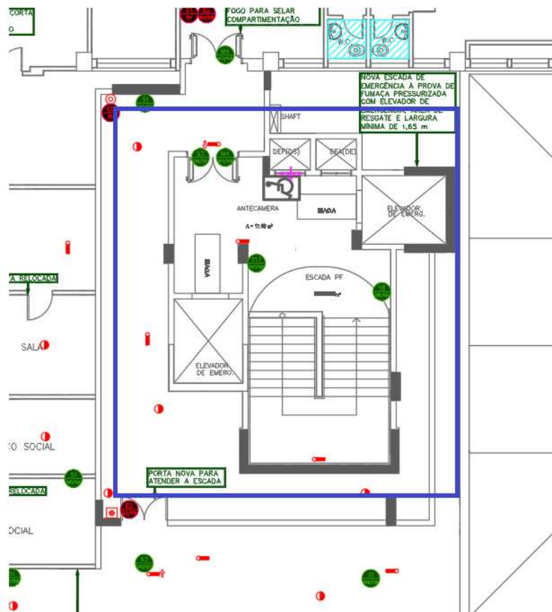
Figura 65 – 1º PAVIMENTO– CONJUNTO EMERGÊNCIA 01 – Novo layout
