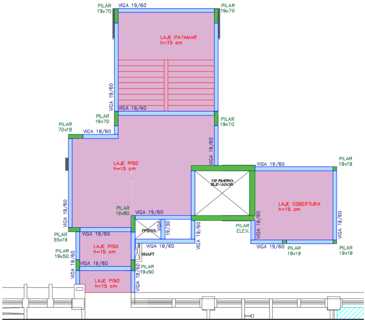
Figura 98 – 2º PAVIMENTO– CONJUNTO EMERGÊNCIA 02 – Croqui Estrutura
