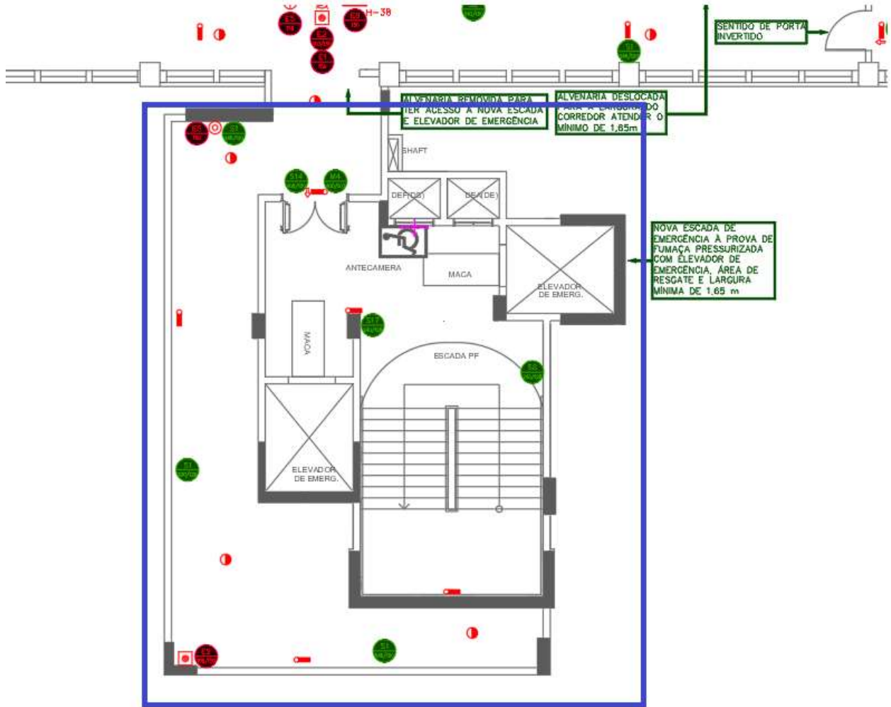
Figura 70 – 6º PAVIMENTO– CONJUNTO EMERGÊNCIA 01 – Novo layout
