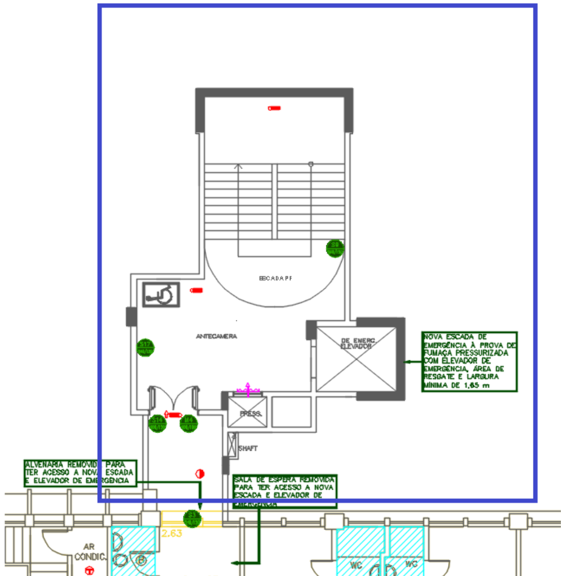
Figura 91 – 7º PAVIMENTO– CONJUNTO EMERGÊNCIA 02 – Novo layout
