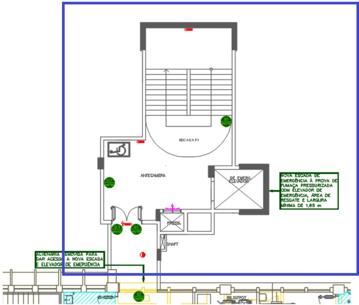
Figura 92 – 8º PAVIMENTO– CONJUNTO EMERGÊNCIA 02 – Novo layout
