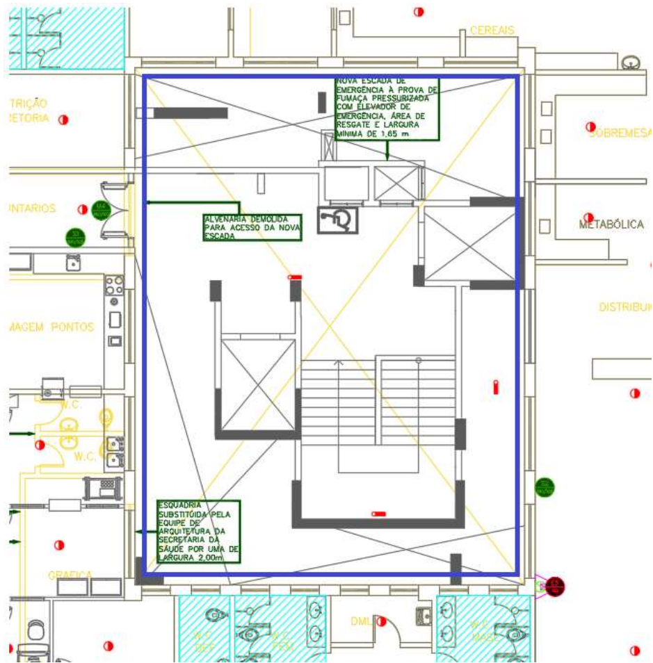
Figura 63 – 1º SUBSOLO – CONJUNTO EMERGÊNCIA 01 – Novo layout
