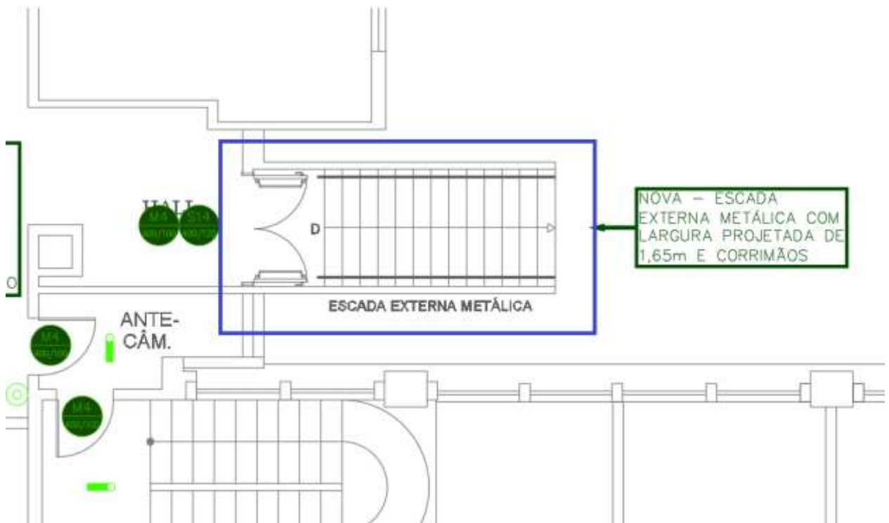
Figura 56 – ESCADA METÁLICA – 2º PAVIMENTO - Layout da chegada da nova escada metálica externa
