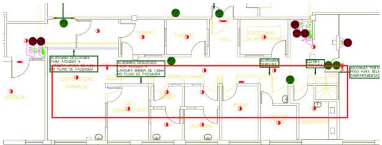
Figura 28 – 1º SUBSOLO – Demolição(amarelo)/reconstrução paredes
