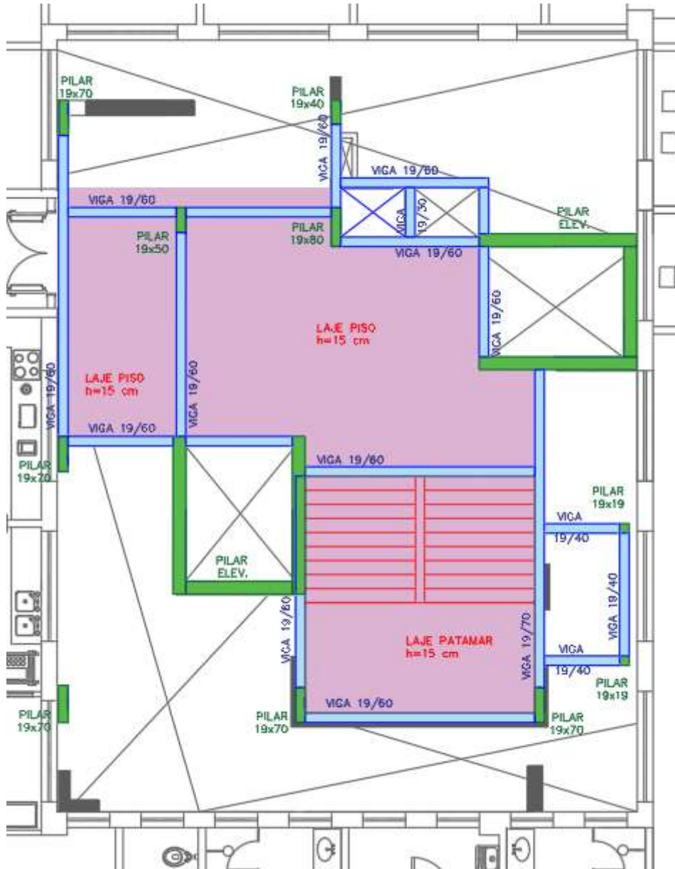
Figura 78 – 1º SUBSOLO – CONJUNTO EMERGÊNCIA 01 – Croqui Estrutura
