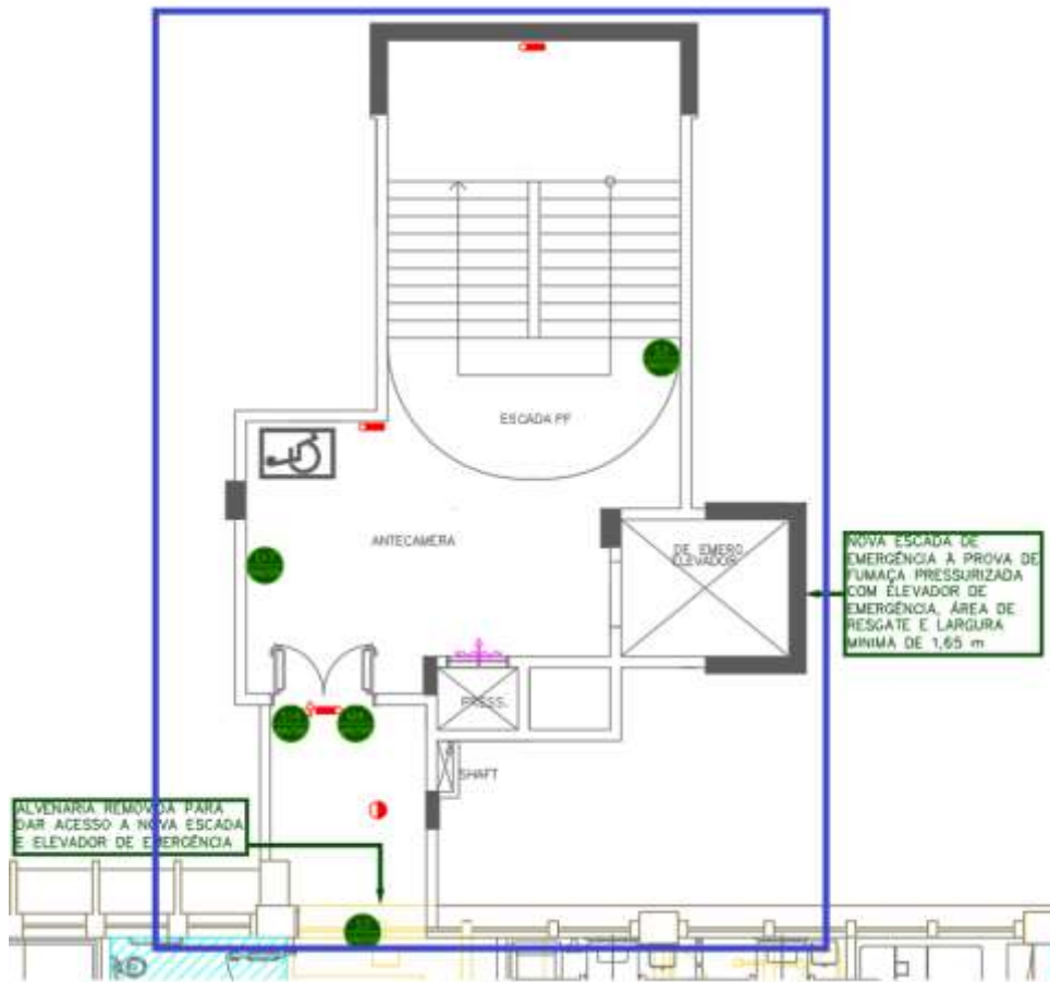
Figura 93 – 9º PAVIMENTO– CONJUNTO EMERGÊNCIA 02 – Novo layout
