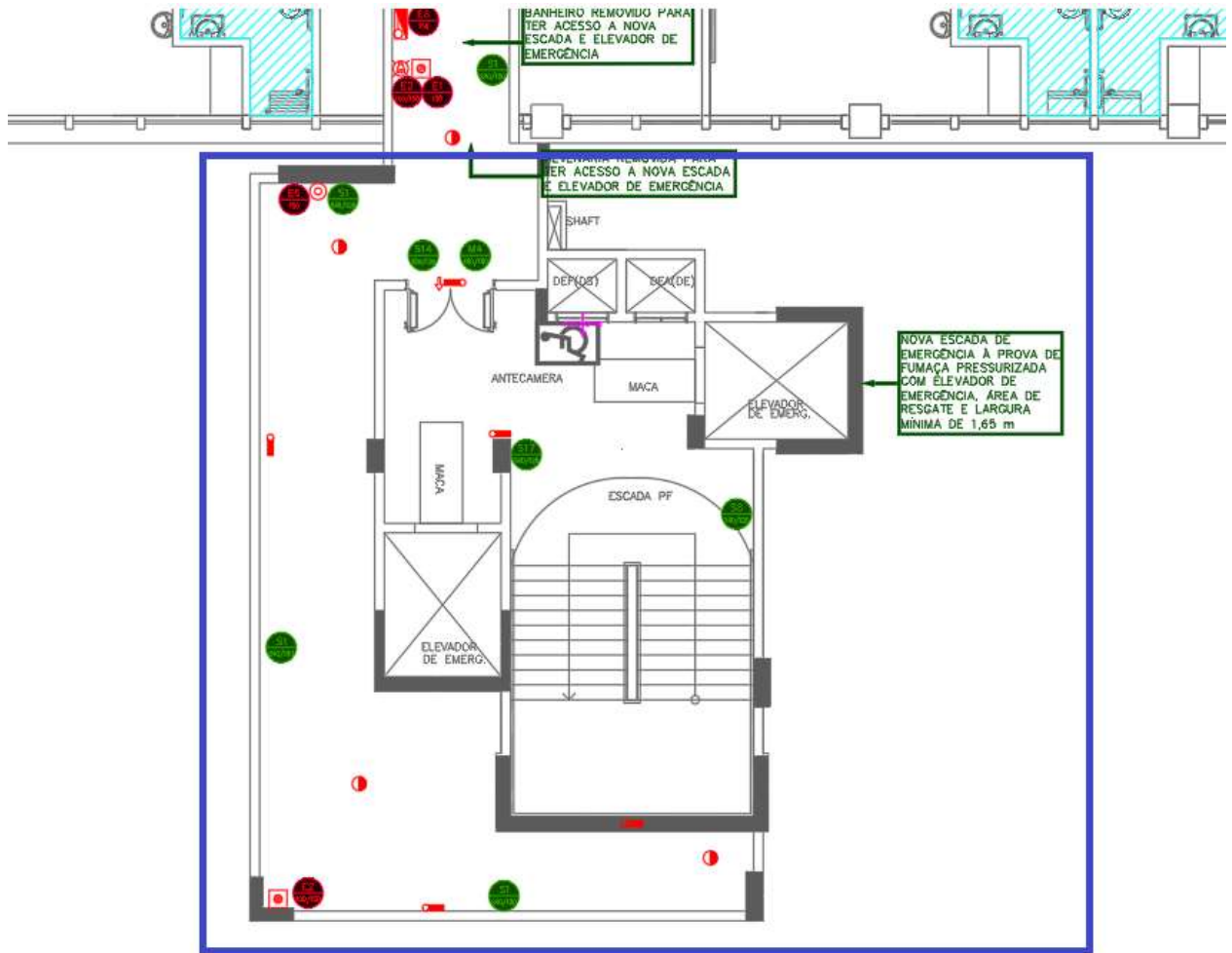
Figura 71 – 7º PAVIMENTO– CONJUNTO EMERGÊNCIA 01 – Novo layout
