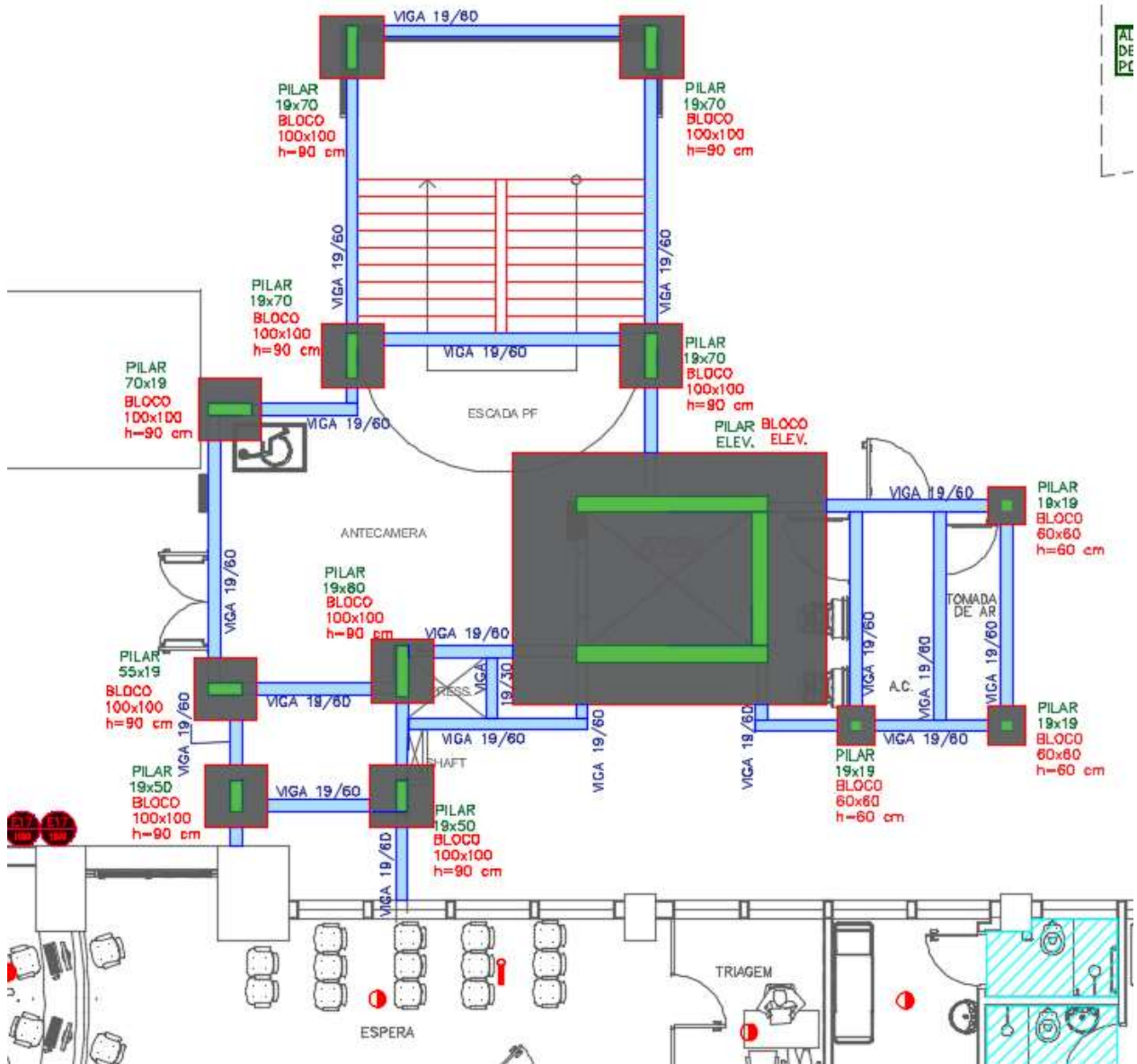
Figura 97 – 1º PAVIMENTO- CONJUNTO EMERGÊNCIA 02 – Croqui Estrutura
