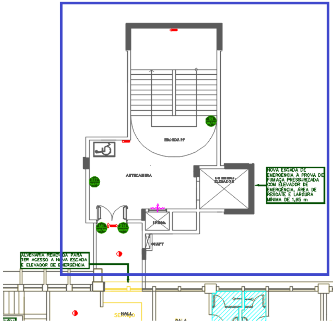
Figura 89 – 5º PAVIMENTO– CONJUNTO EMERGÊNCIA 02 – Novo layout
