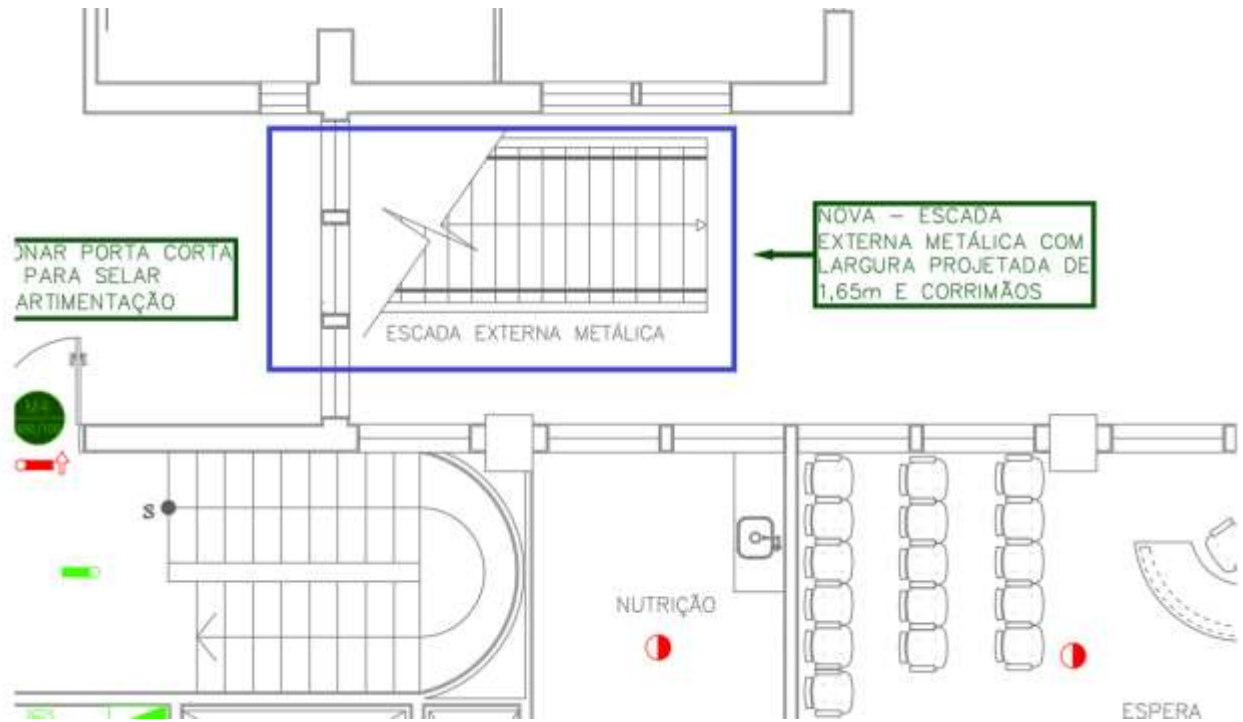
Figura 55 – ESCADA METÁLICA – 1º PAVIMENTO – Layout da saída da nova escada metálica externa
