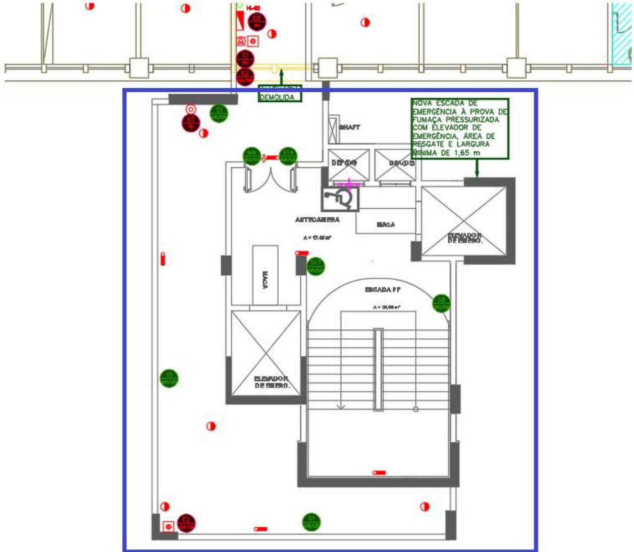
Figura 66 – 2º PAVIMENTO– CONJUNTO EMERGÊNCIA 01 – Novo layout
