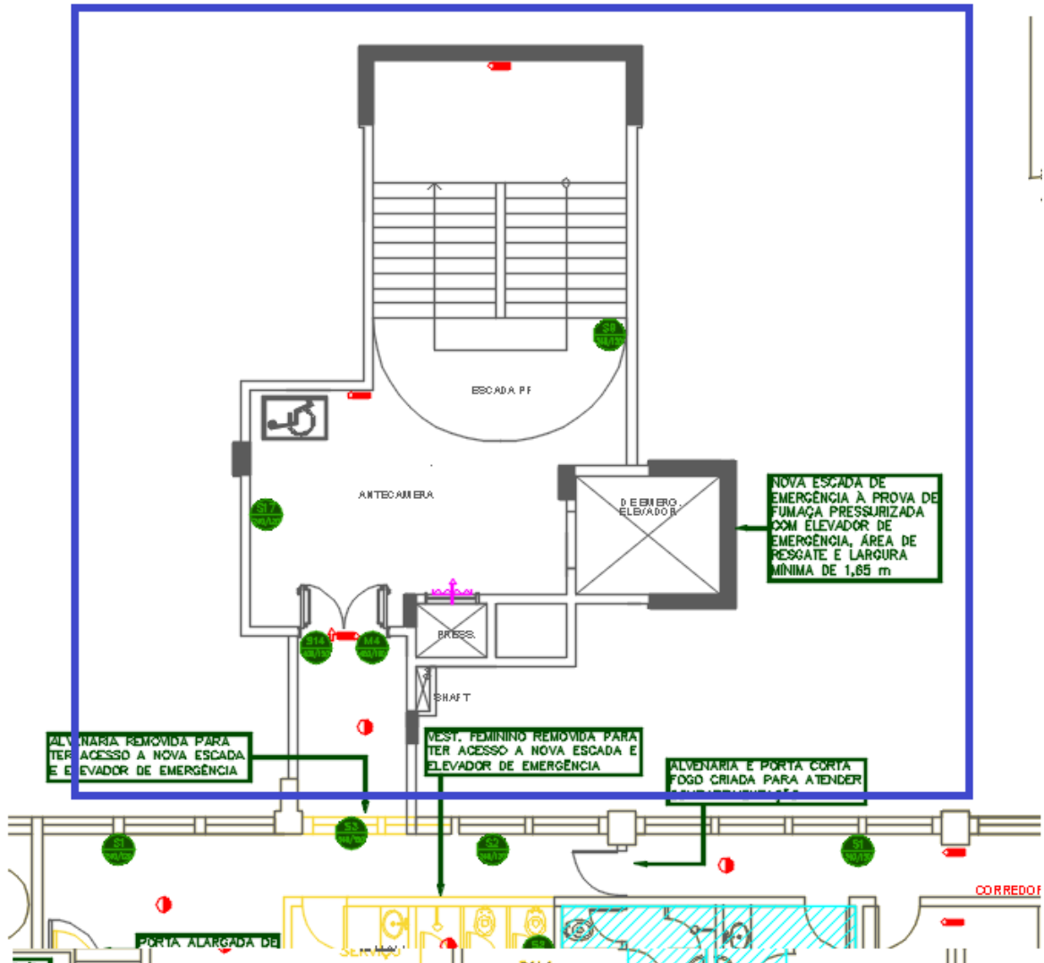
Figura 90 – 6º PAVIMENTO– CONJUNTO EMERGÊNCIA 02 – Novo layout
