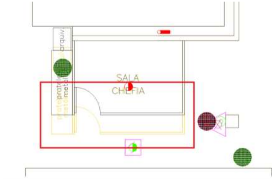
Figura 24 – 2º SUBSOLO – Demolição(amarelo)/reconstrução paredes
