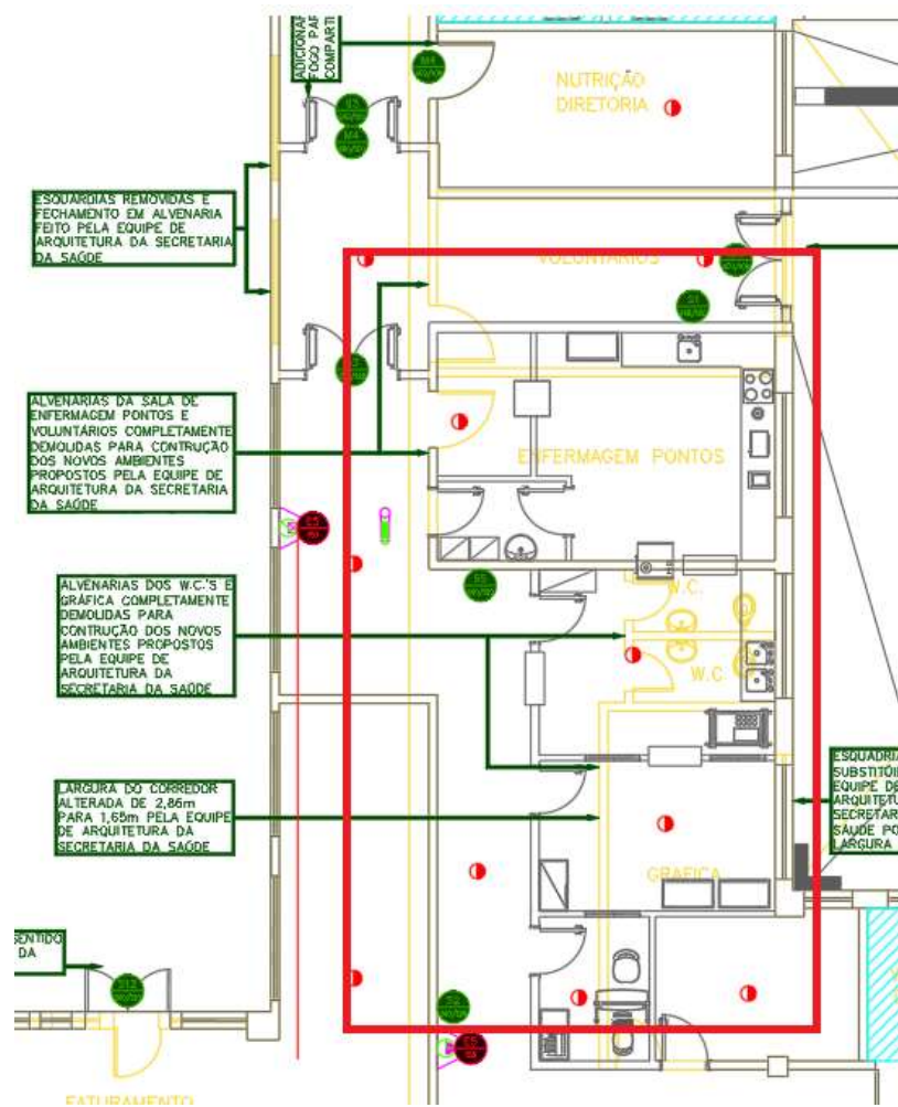
Figura 27 – 1º SUBSOLO – Demolição(amarelo)/reconstrução paredes para mudança de layout
