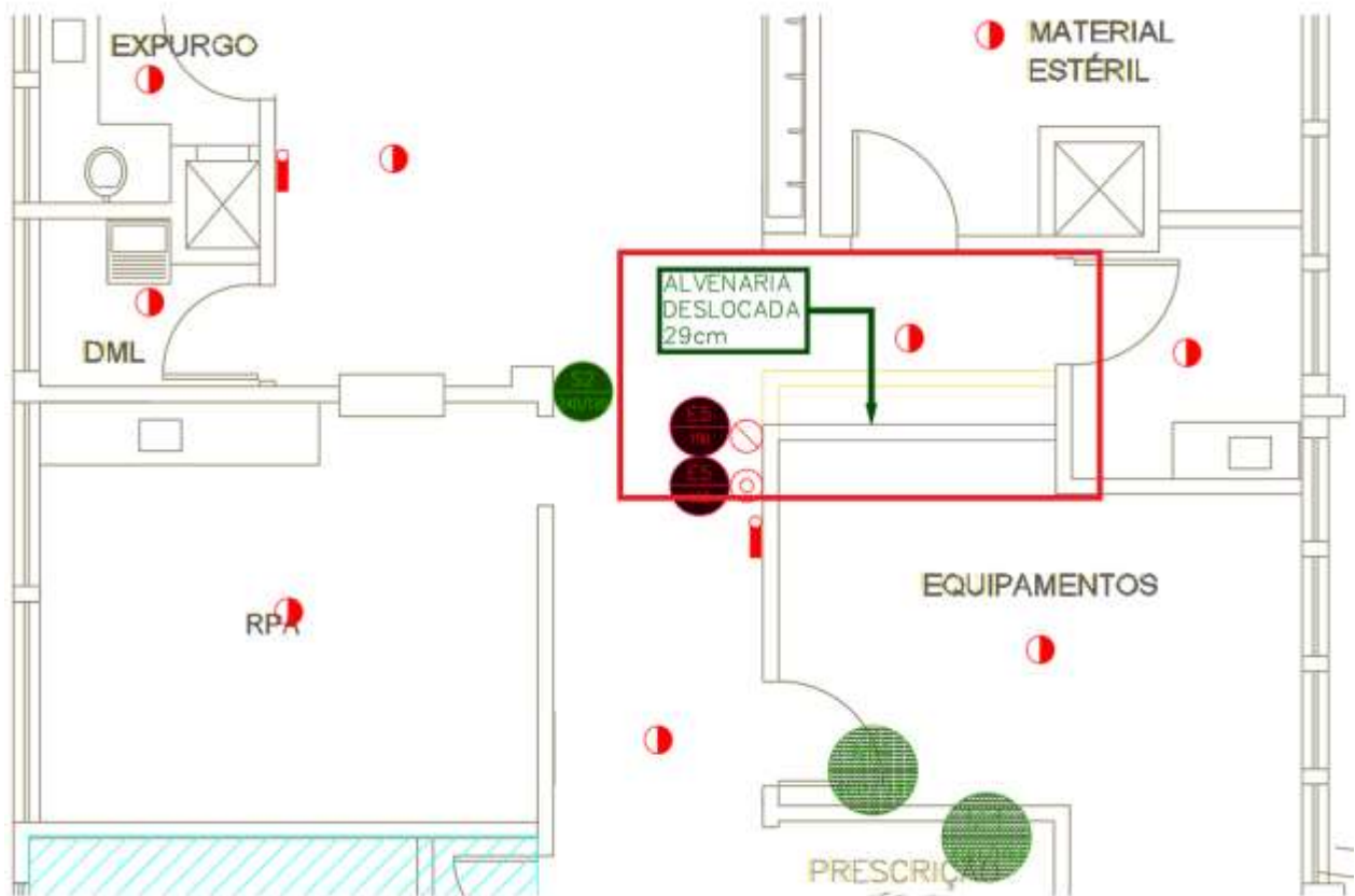
Figura 39 – 5º PAVIMENTO – Demolição(amarelo)/reconstrução paredes para mudança de layout
