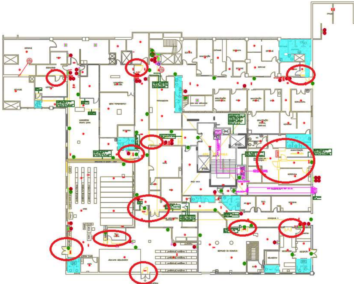
Figura 9 – 2º SUBSOLO – Inversão no sentido de porta/Remoção e instalação de novas portas
