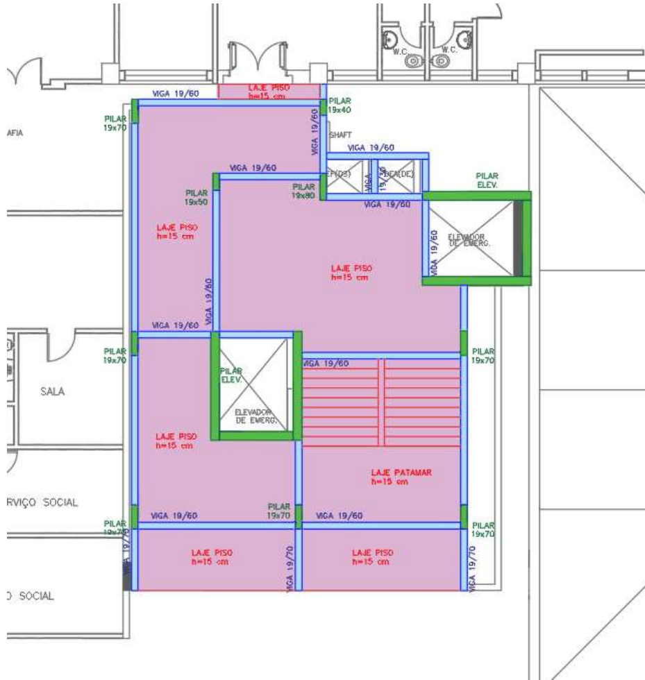
Figura 79 – 1º PAVIMENTO – CONJUNTO EMERGÊNCIA 01 – Croqui Estrutura
