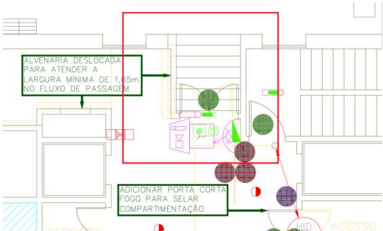
Figura 102 –1º SUBSOLO – Ampliações da escada –existente (amarelo) x nova
