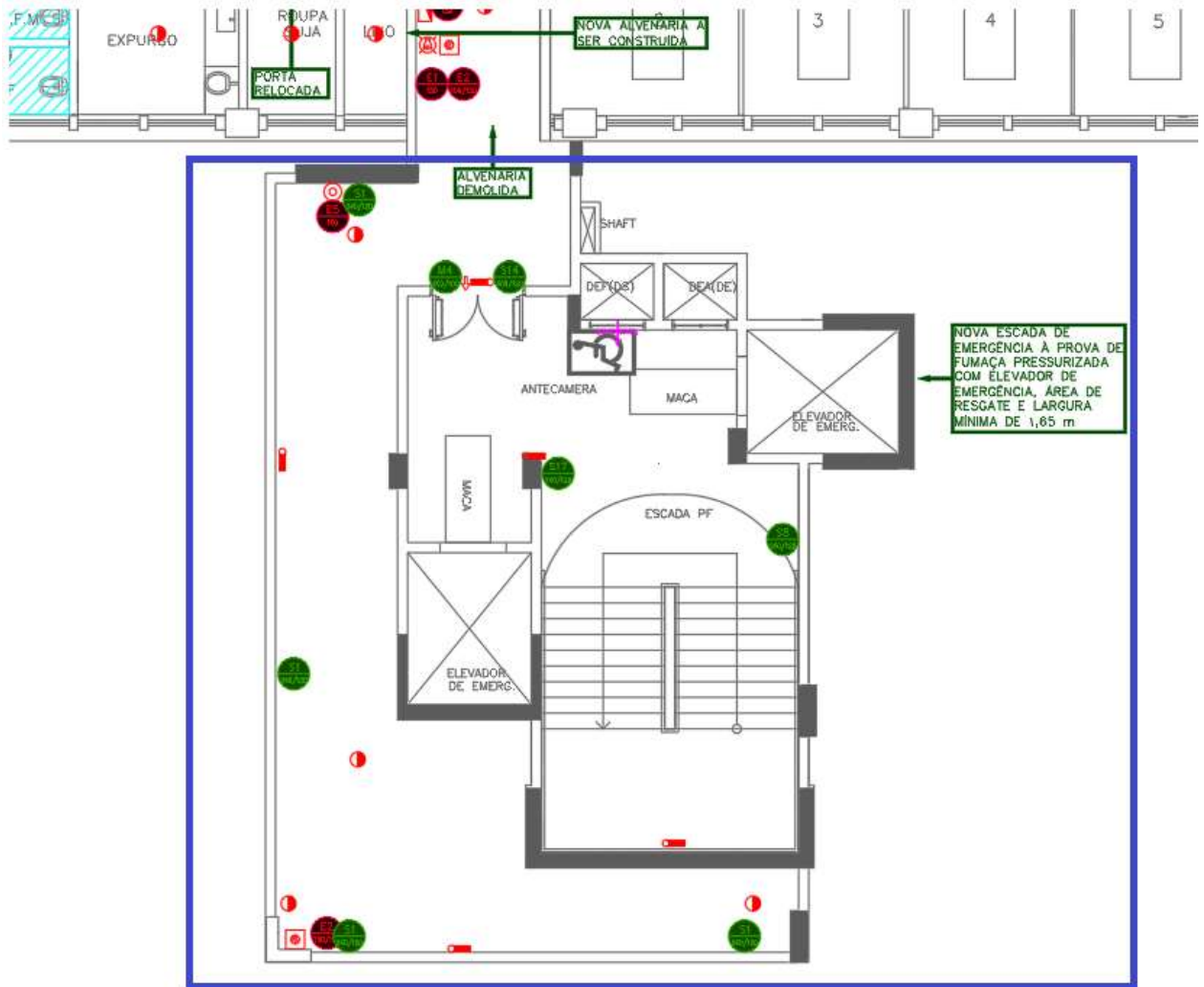
Figura 68 – 4º PAVIMENTO– CONJUNTO EMERGÊNCIA 01 – Novo layout
