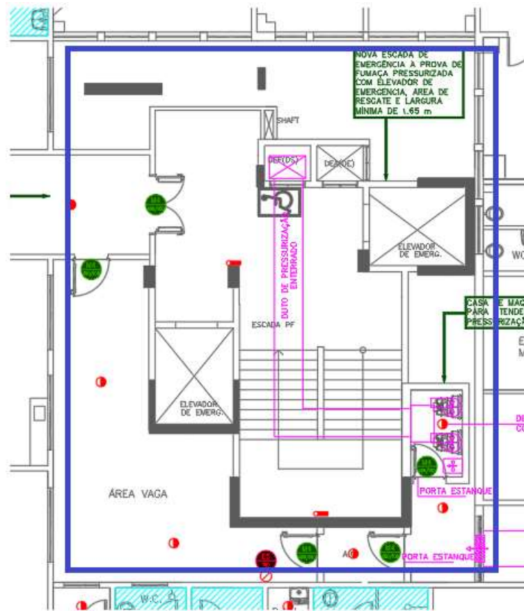
Figura 61 – 2º SUBSOLO – CONJUNTO EMERGÊNCIA 01 – Novo layout
